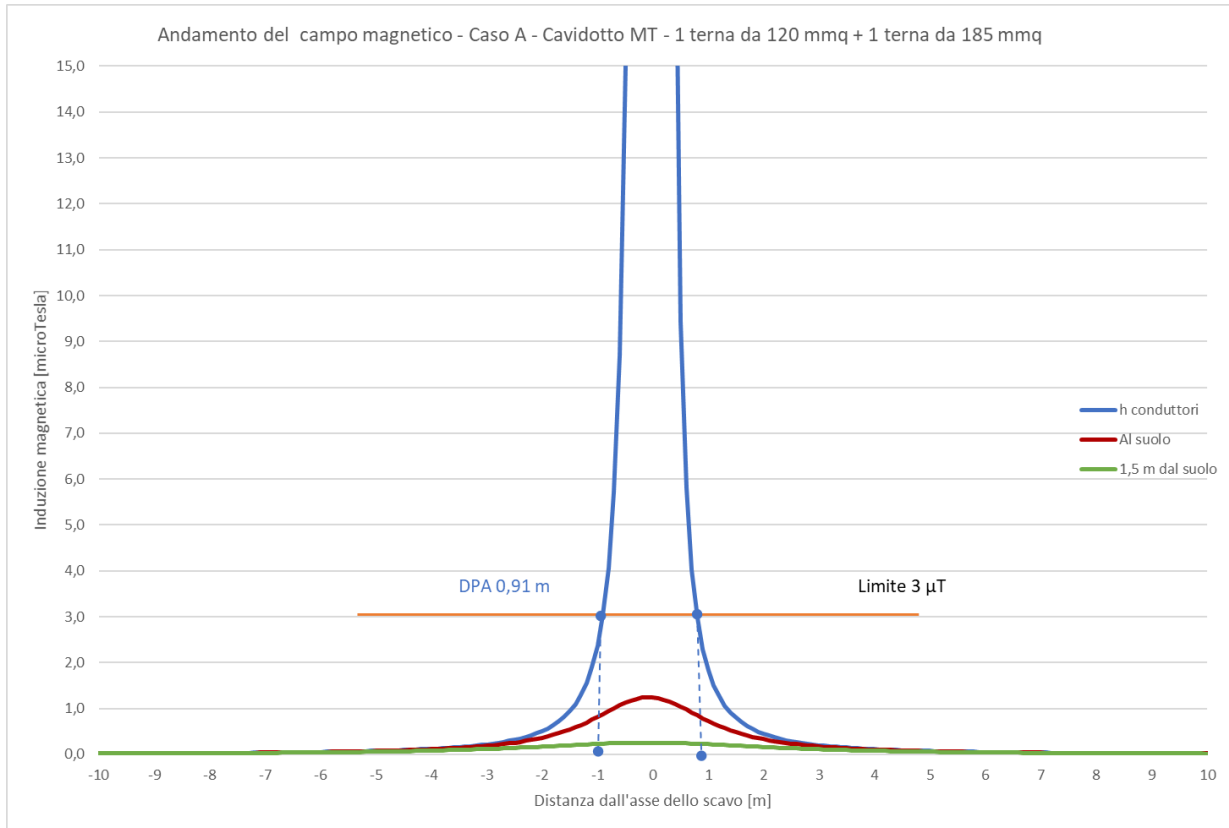
Figura 2 - Andamento del campo magnetico in funzione della distanza dall'asse dei conduttori in forma grafica relativa alla simulazione A.
