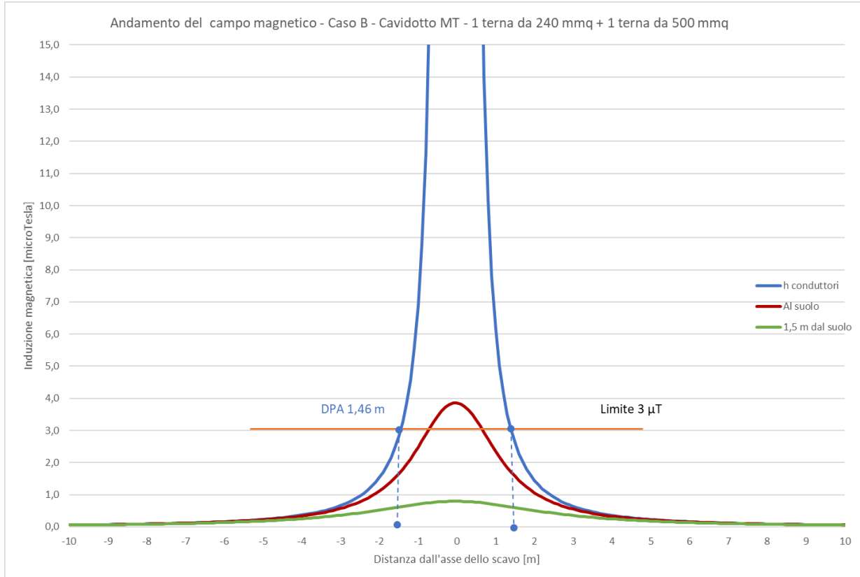
Figura 3 - Andamento del campo magnetico in funzione della distanza dall'asse dei conduttori in forma grafica relativa alla simulazione B.
