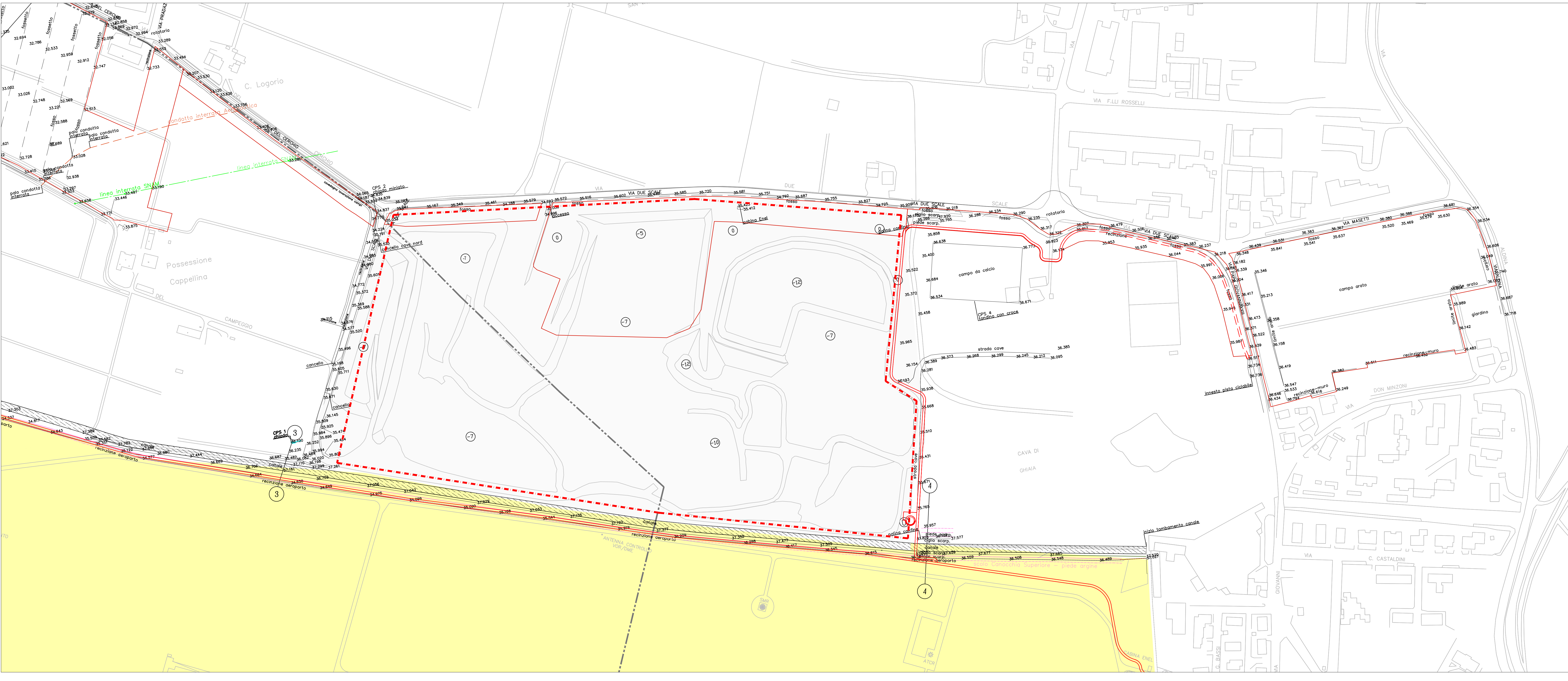
Rilievo dello stato attuale - 02 di 2 scala 1:2.000
