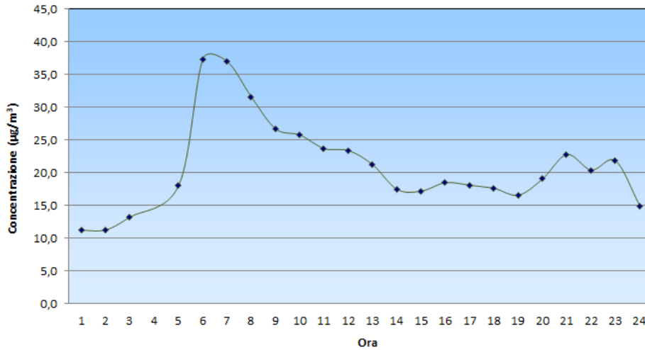
SITO RICETTIVO "MOLINARI" - DAL 21/06/2017 AL 28/07/2017 Biossido di azoto: giorno tipo
