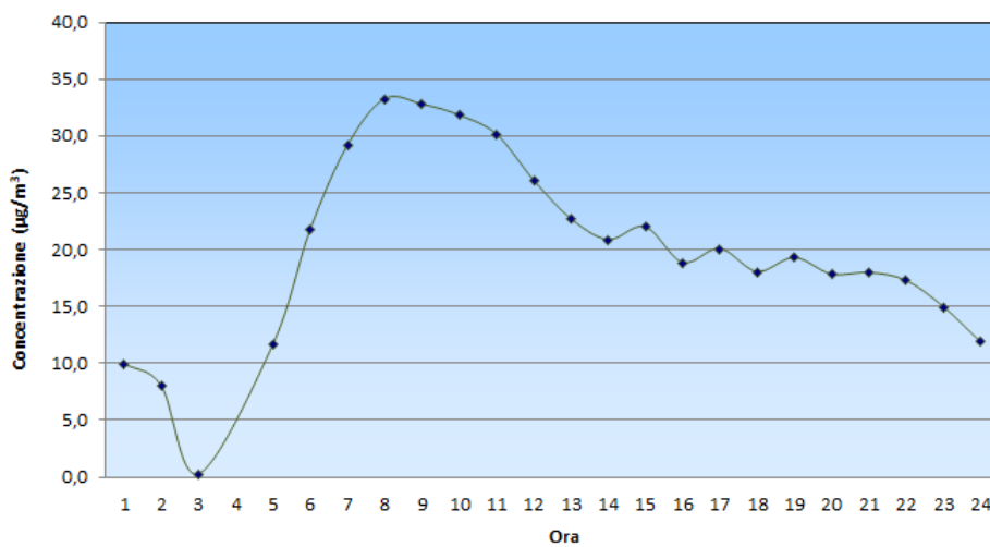
SITO RICETTIVO "SANTA RITA" - DAL 13/07/2017 AL 18/08/2017 Biossido di azoto: giorno tipo
