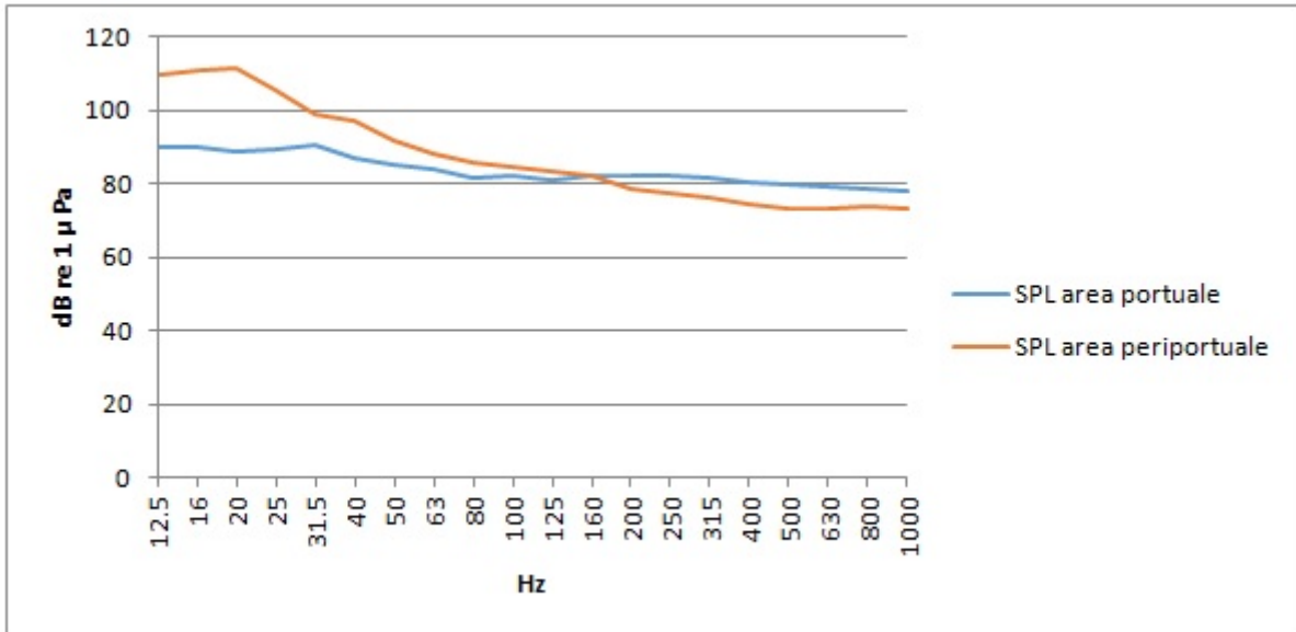
Fig. 3 Sulle ascisse sono rappresentate le bande in 1/3 di ottava comprese tra 10 e 1000 Hz, sulle ordinate il Livello di Pressione Sonora (SPL) in dB re 1 μ Pa
