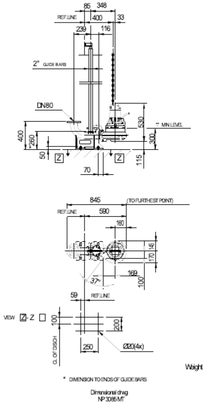
Figura 7.11 – Dimensioni pompa
