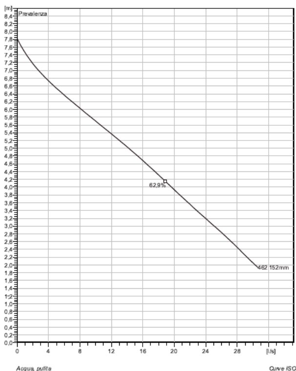
Figura 7.6 – Specifiche tecniche pompa
