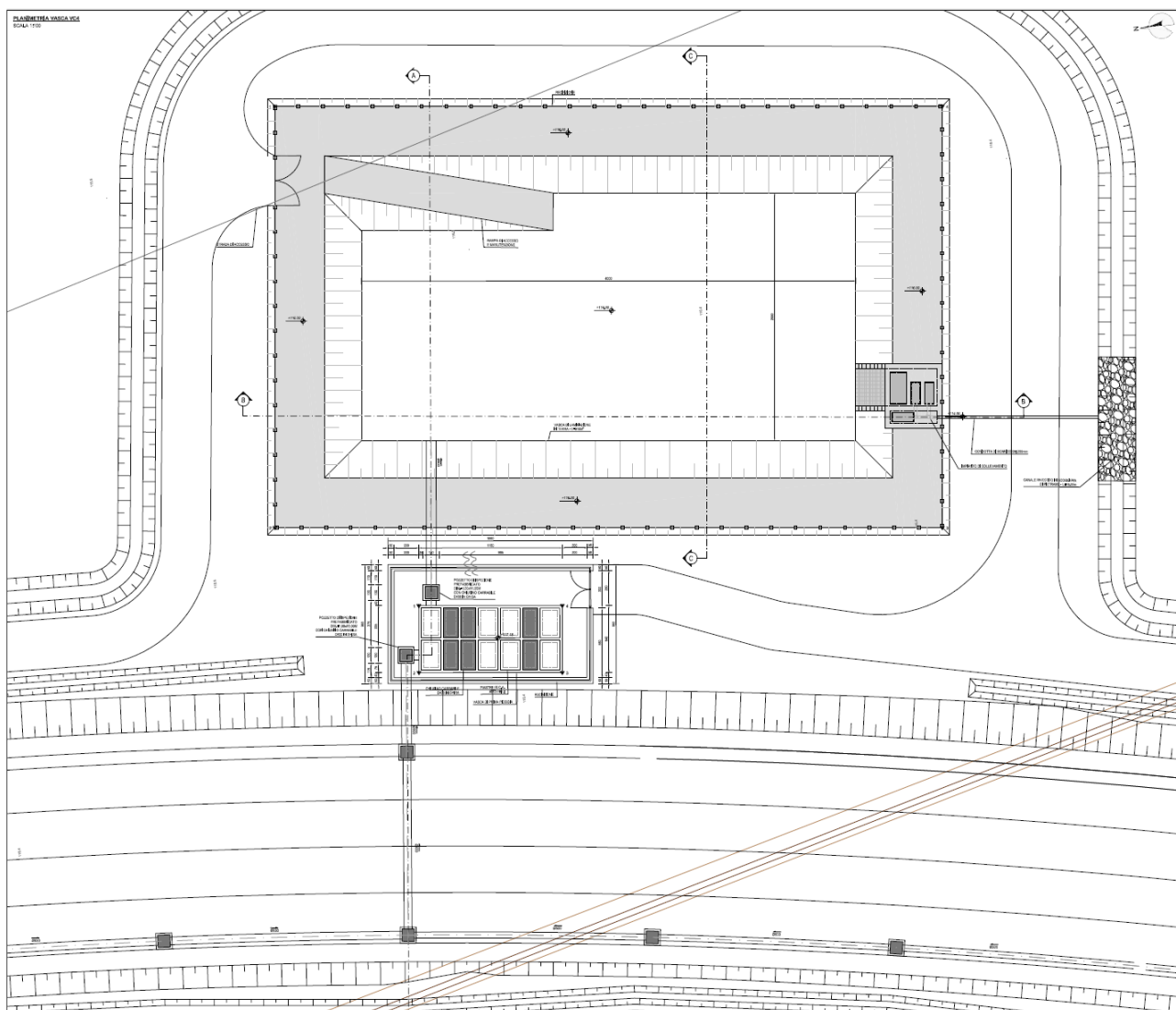
Figura 7.1 - Vasca di laminazione – sistemazione tipologica
