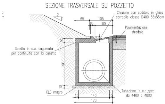
Figura 3-2 - Pozzetto caditoia in cunetta alla francese.
