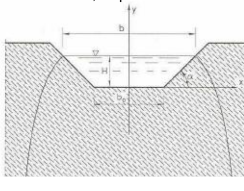
Figura 3-1- Sezione trapezia.
