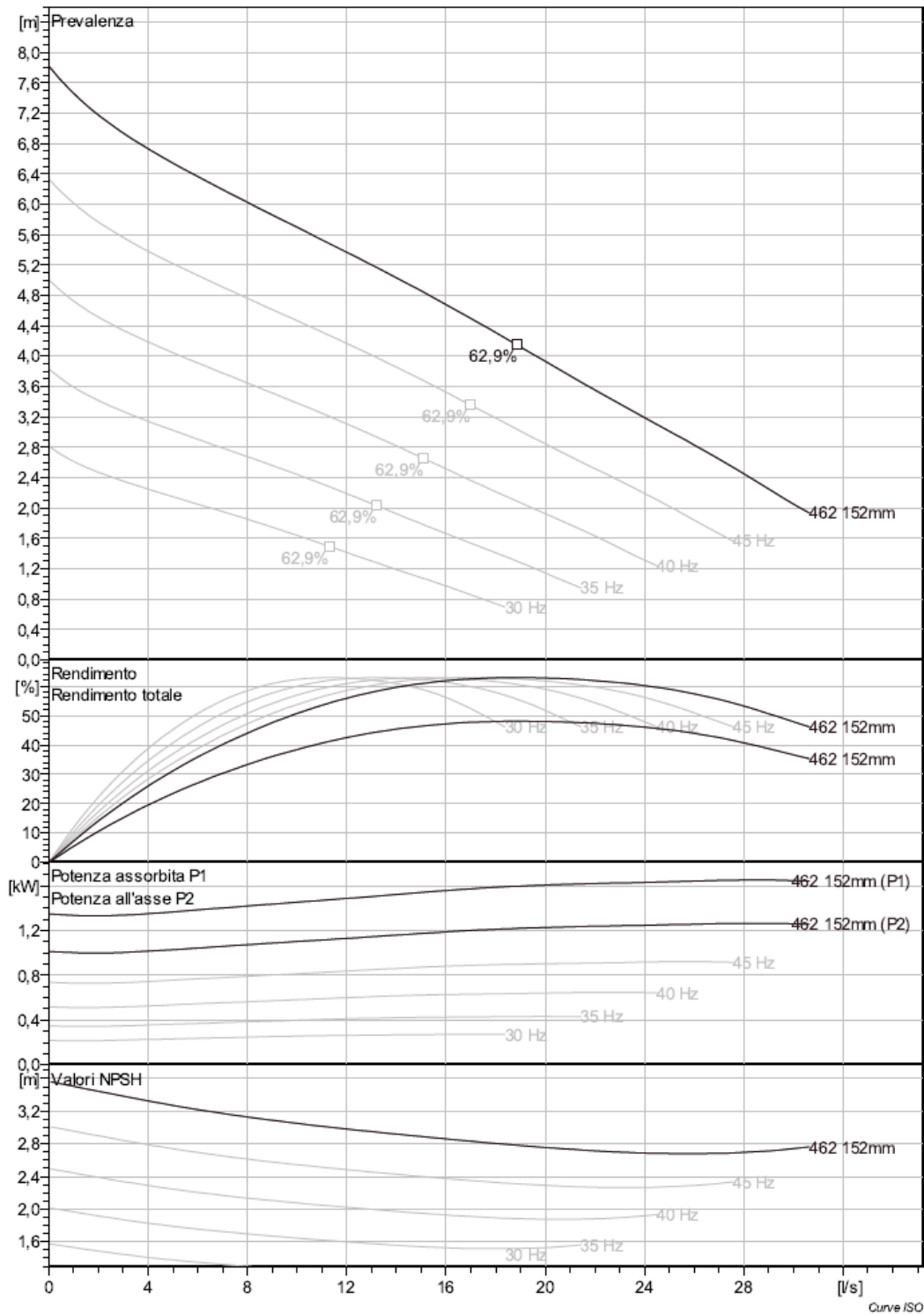
Figura 7.9 – Curva VFD
