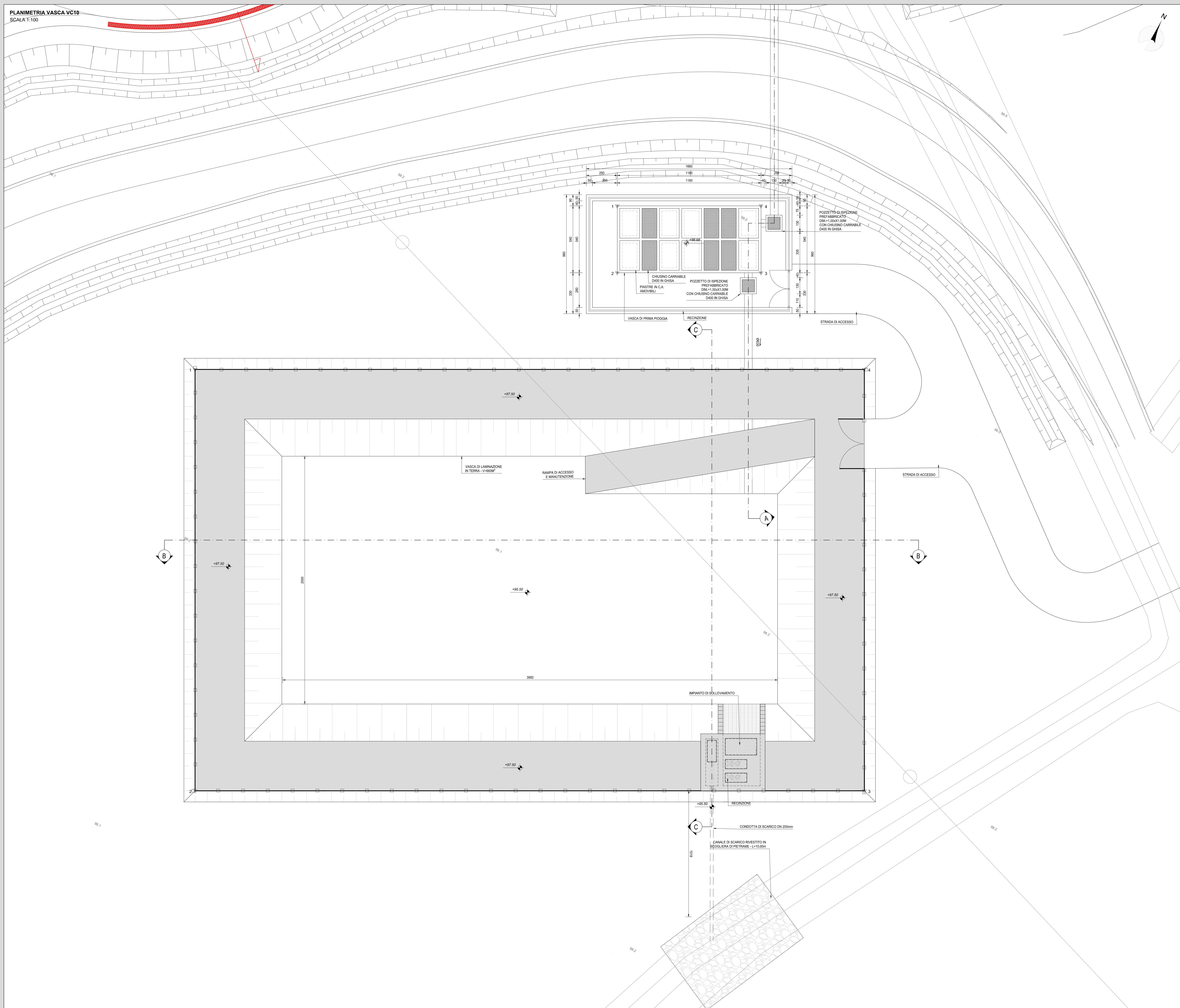
VASCA LAMINAZIONE VC10 E VASCA PRIMA PIOGGIA VPP10
