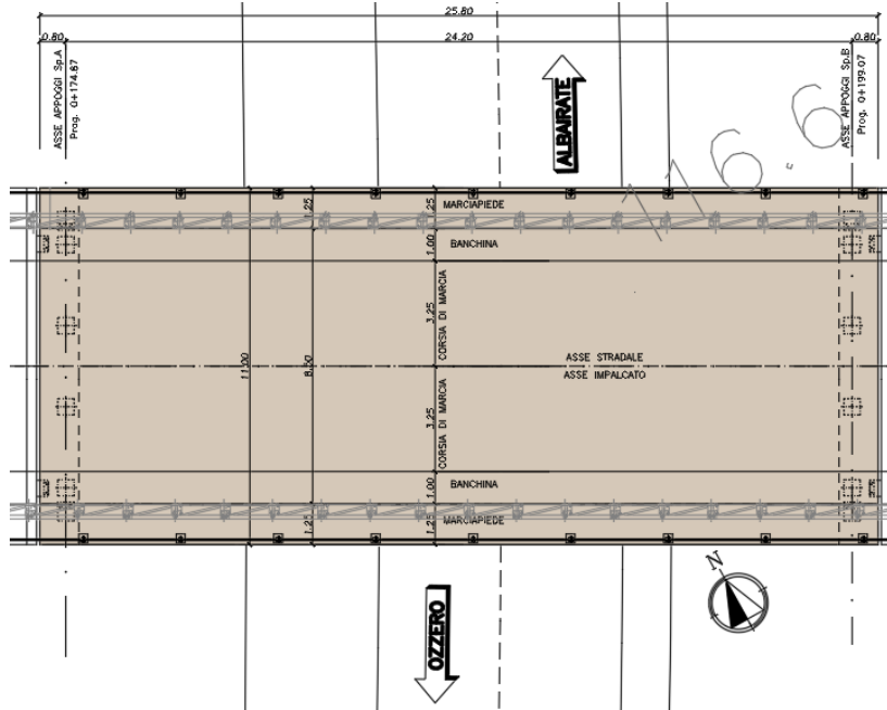
Figura 1: Pianta impalcato
