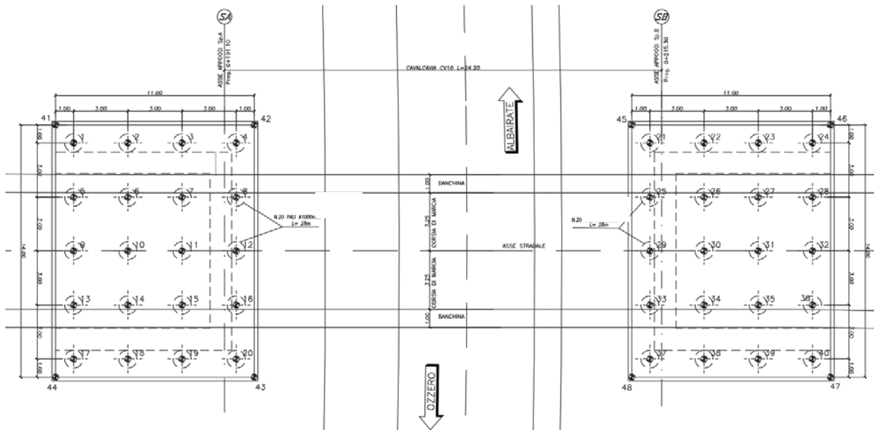
Figura 2: Pianta fondazioni
