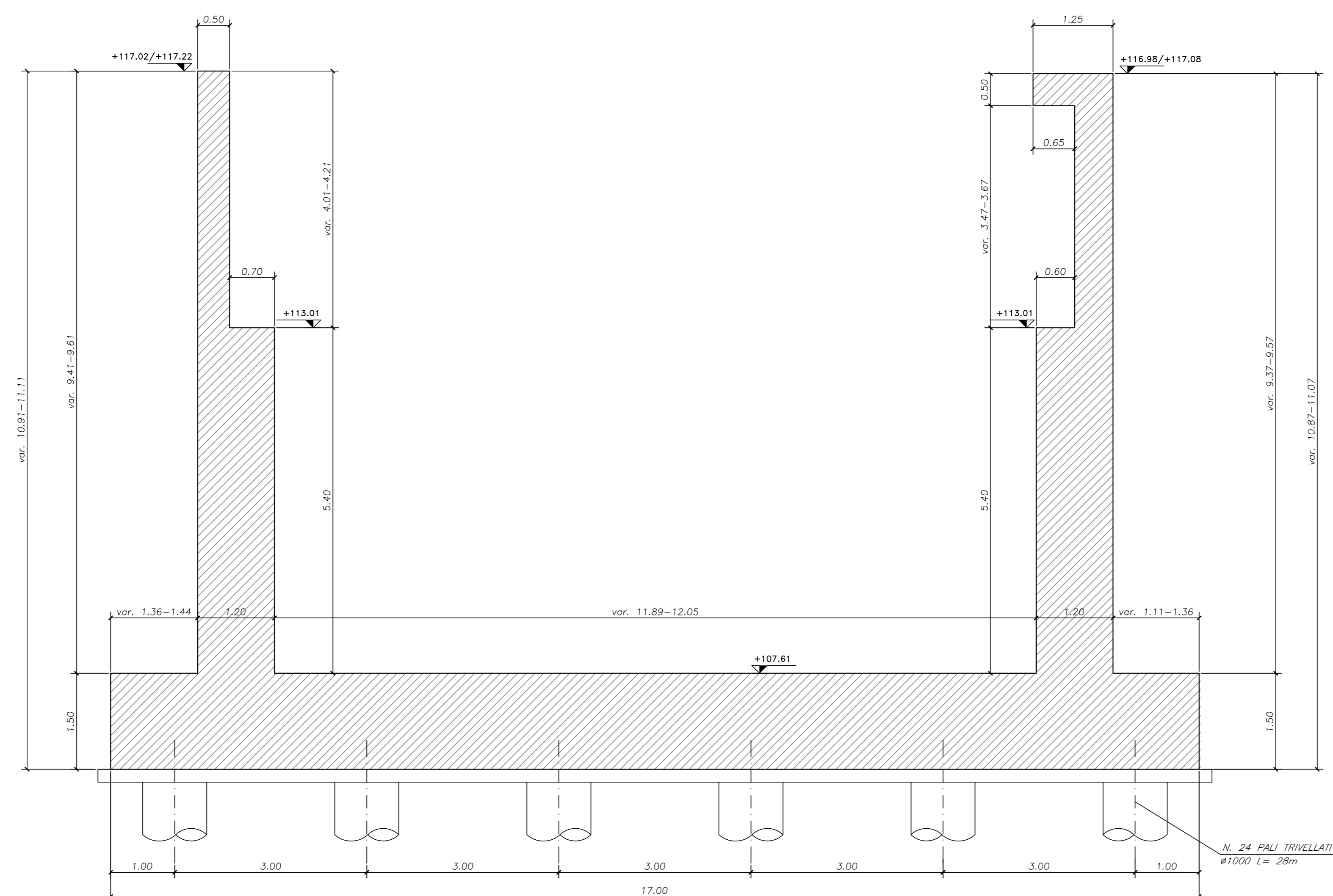
SEZIONE C-C SCALA 1:50
