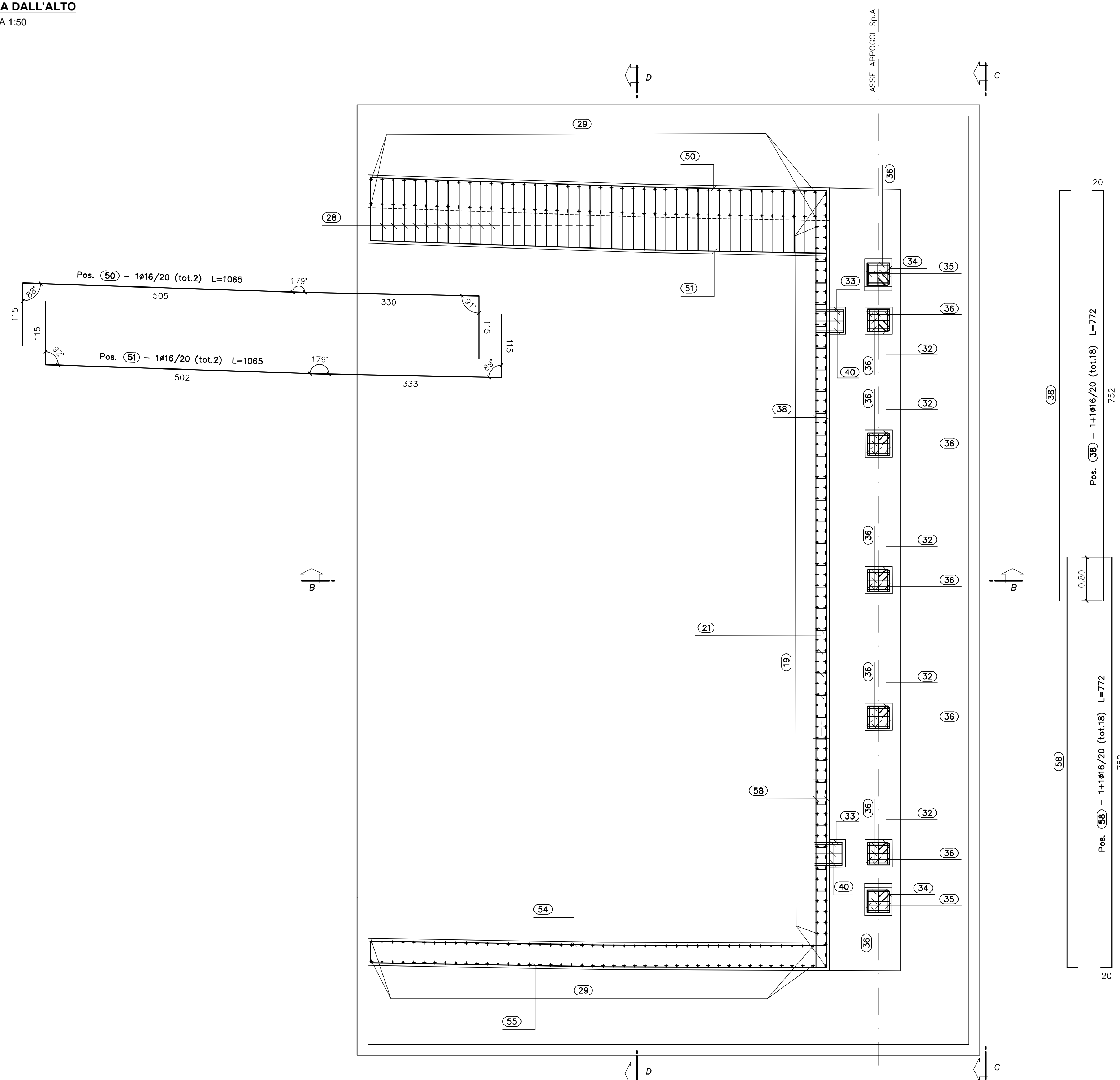
VISTA DALL'ALTO SCALA 1:50
