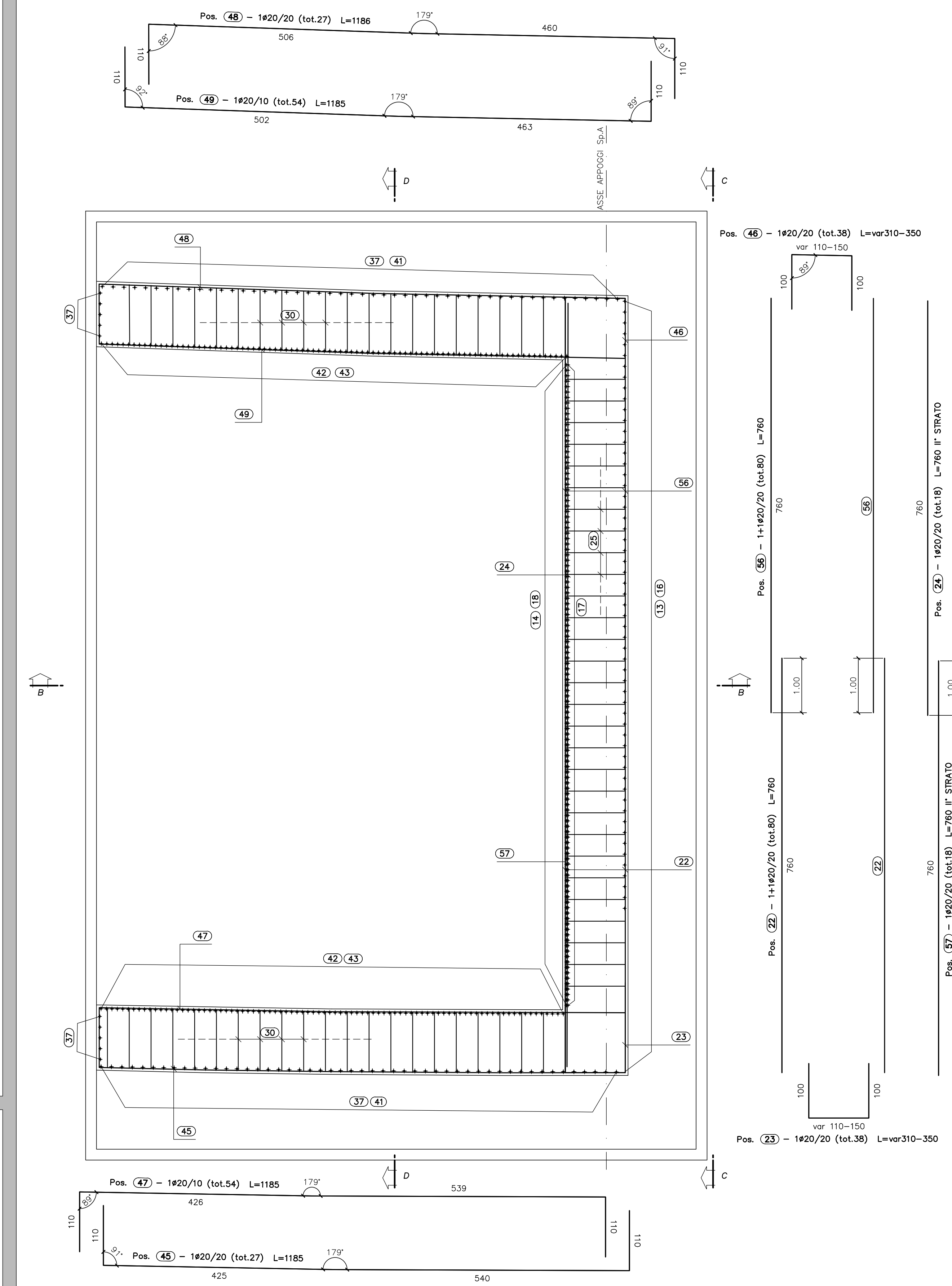
PIANTA SPICCATO SCALA 1:50
