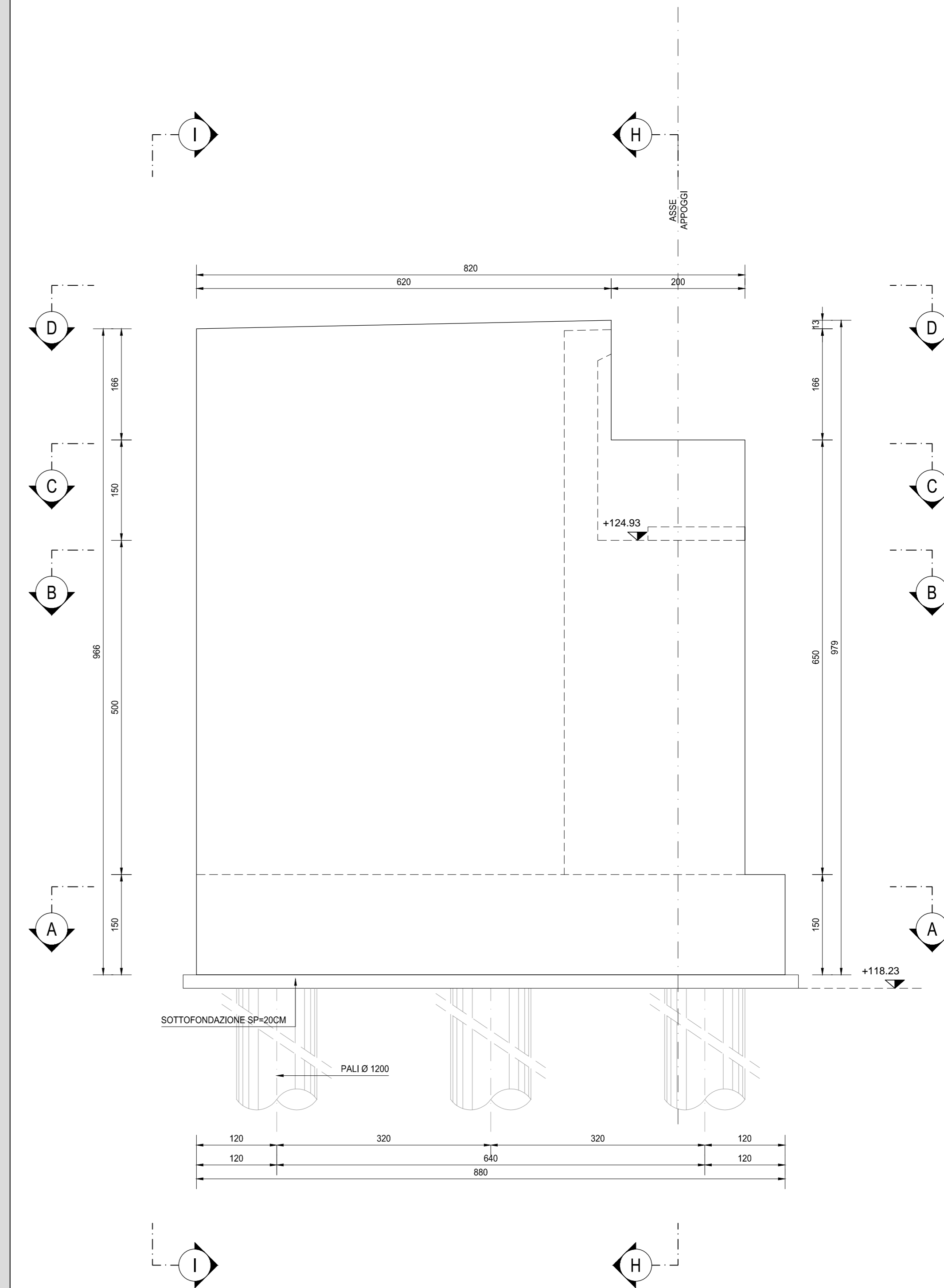
VISTA F-F SCALA 1:50
