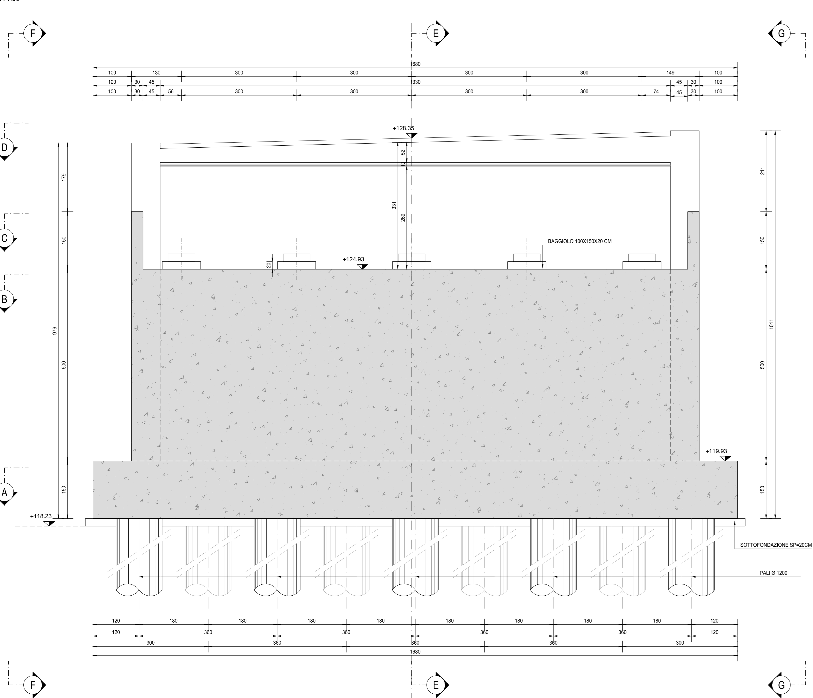
SEZIONE H-H SCALA 1:50
