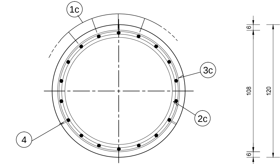
SEZIONE C-C
