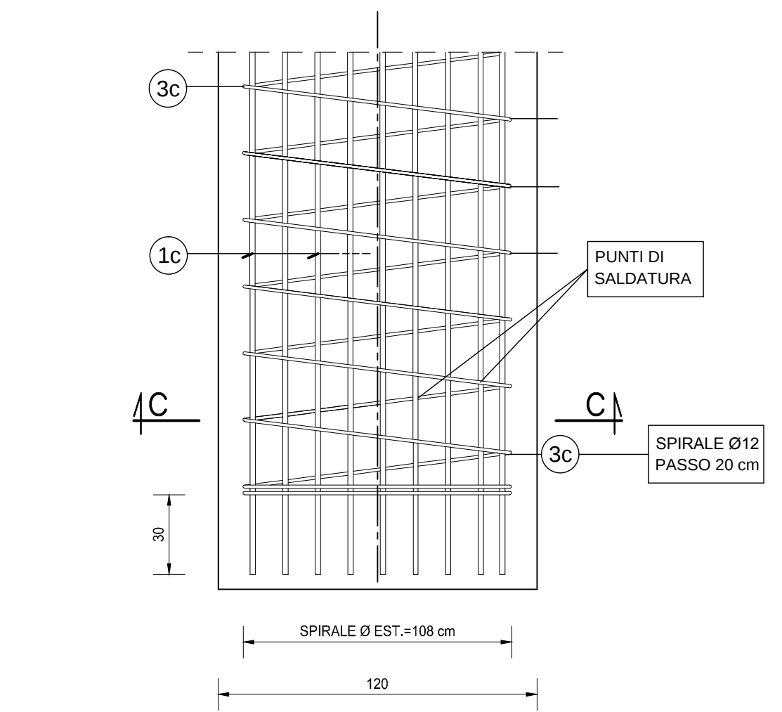
PARTICOLARE 03
