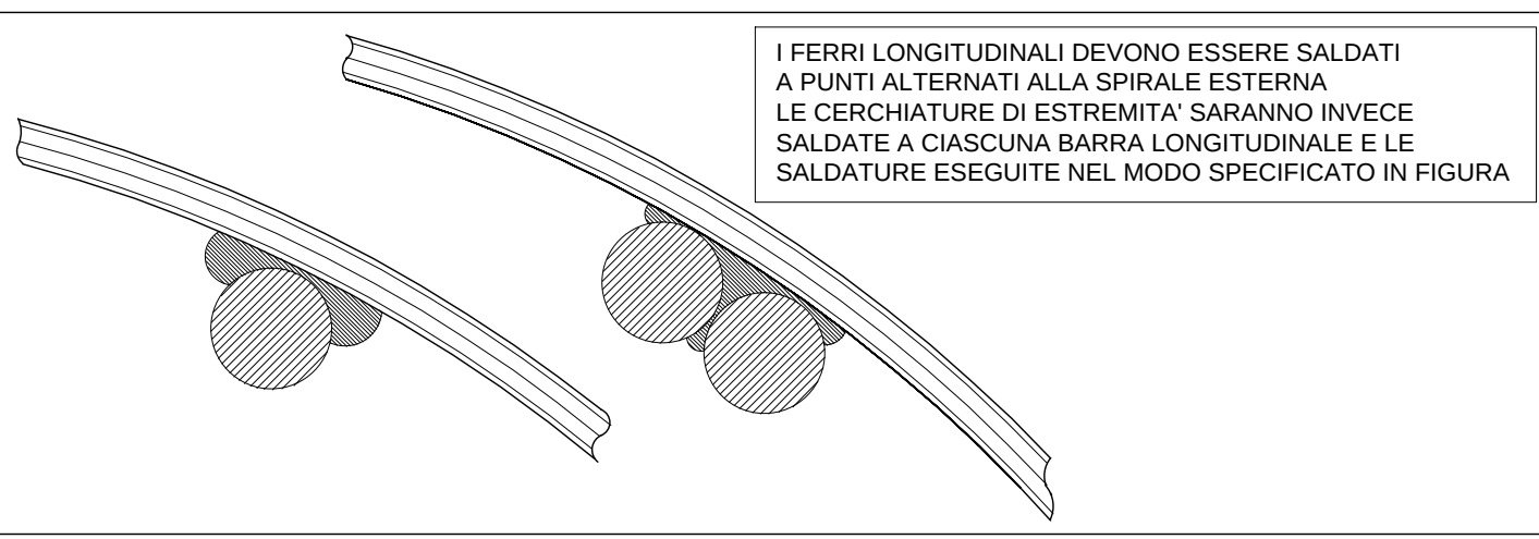
PARTICOLARE SALDATURA
