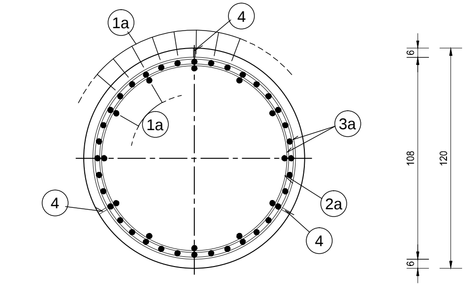
SEZIONE A-A
