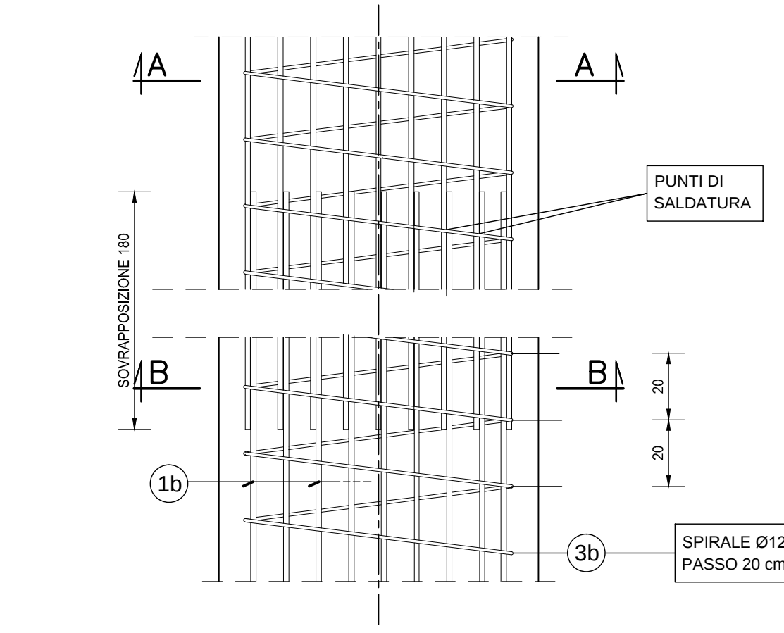
PARTICOLARE 03
