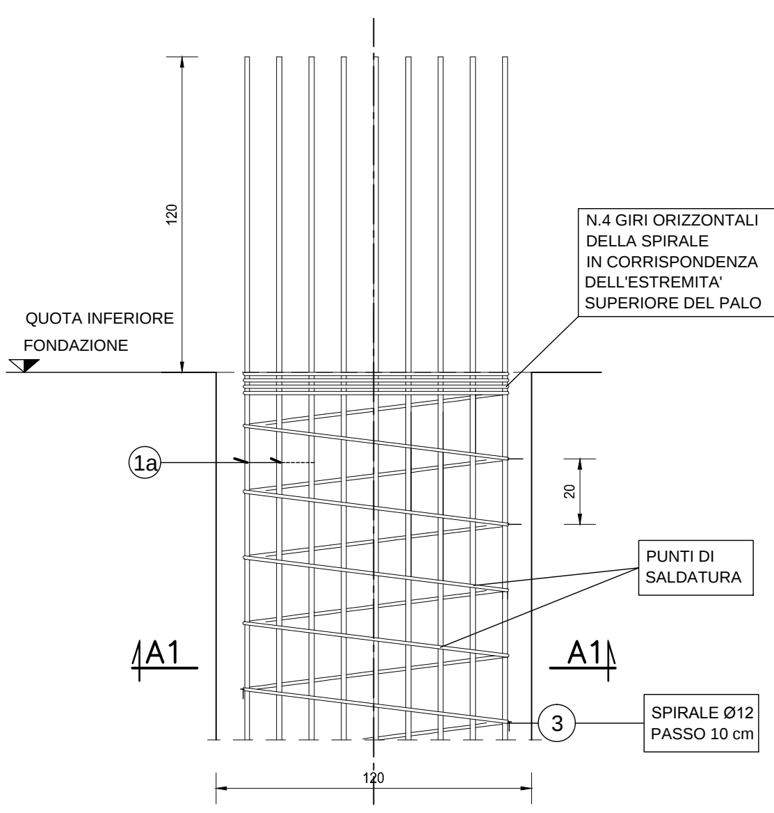
PARTICOLARE 02
