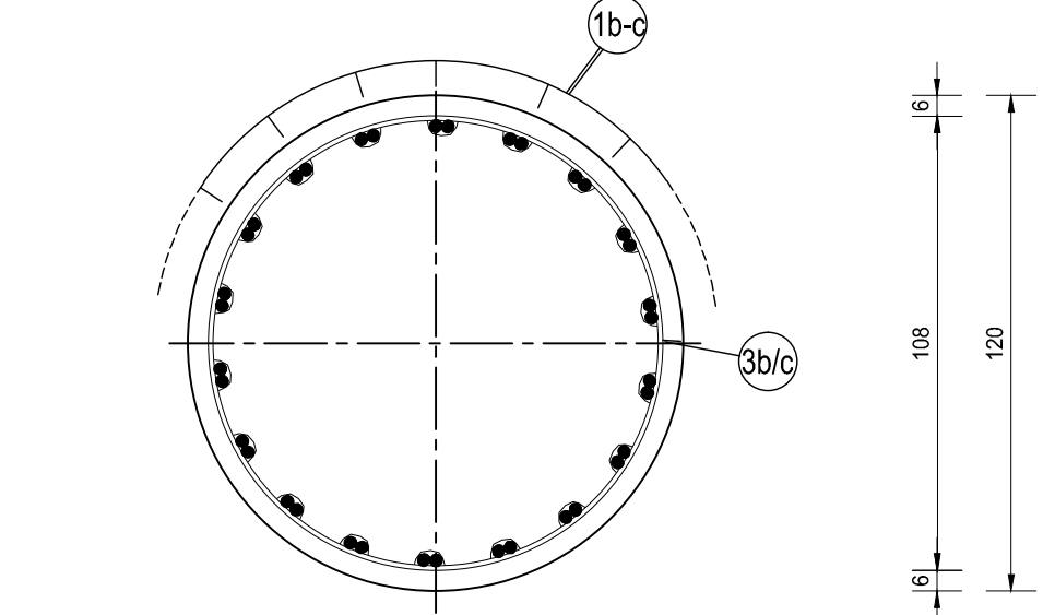
SEZIONE C-C
