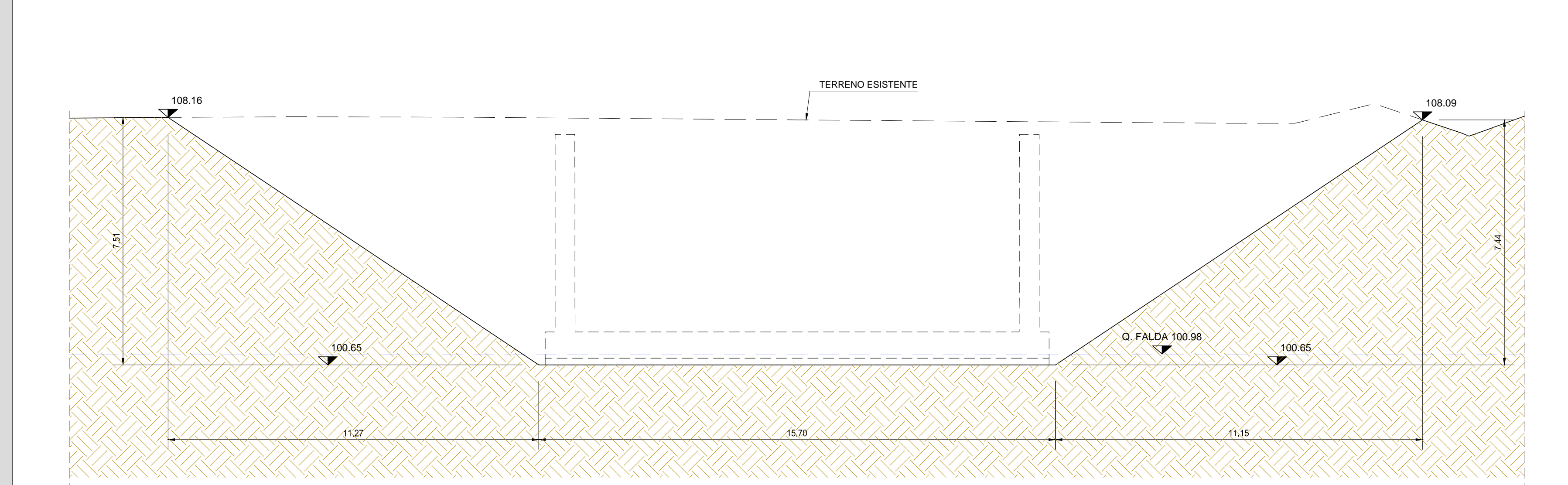
SEZIONE F-F SCALA 1:100
