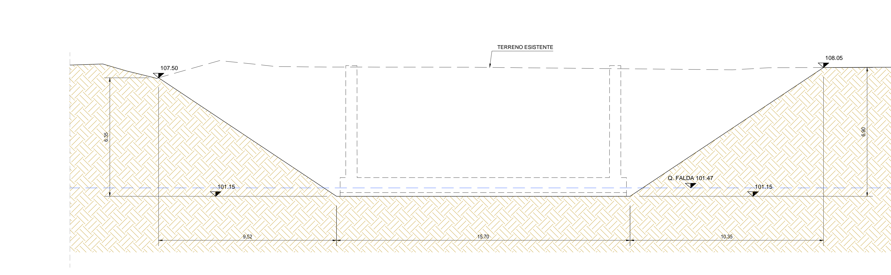
SEZIONE G-G SCALA 1:100
