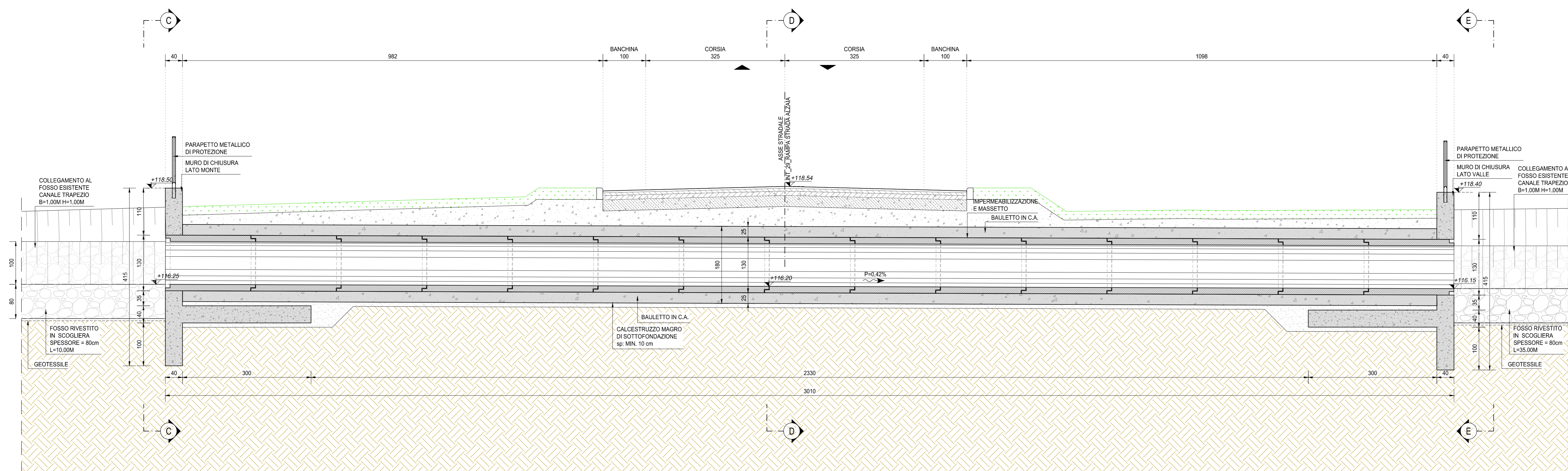
SEZIONE LONGITUDINALE (SEZIONE A-A) SCALA 1:50
