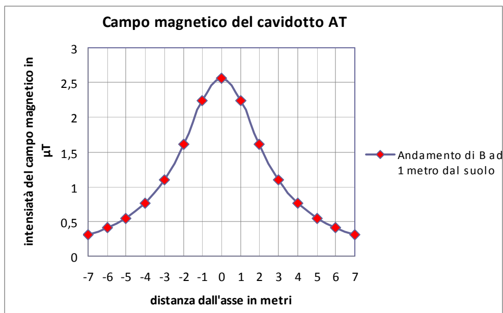
Figura 12 Campo magnetico cavidotto AT ad 1 m dal suolo.
