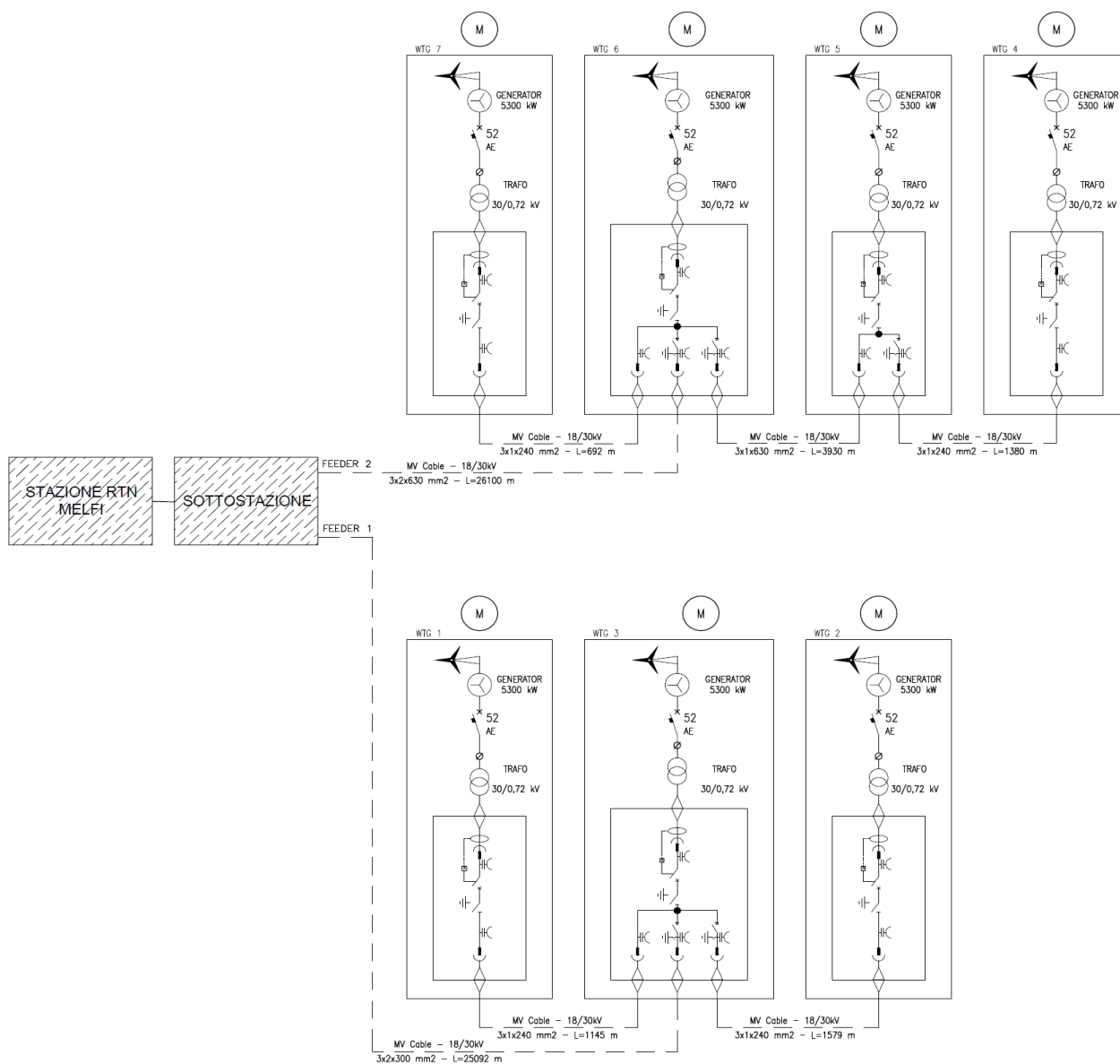
Figura 2 – Schema unifilare
