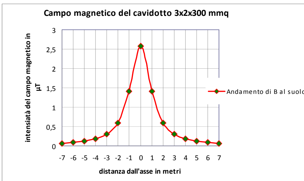
Figura 6 Campo magnetico cavidotto 3x2x300mmq al suolo.
