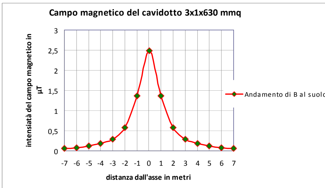
Figura 8 Campo magnetico cavidotto 3x1x630mmq al suolo.
