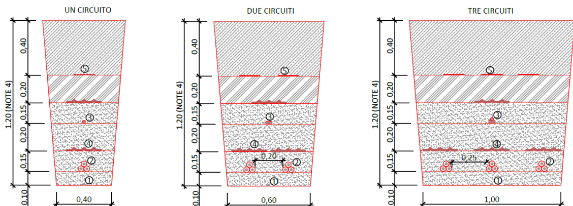
Figura 1 – Tipologico sezione di scavo cavidotto.
