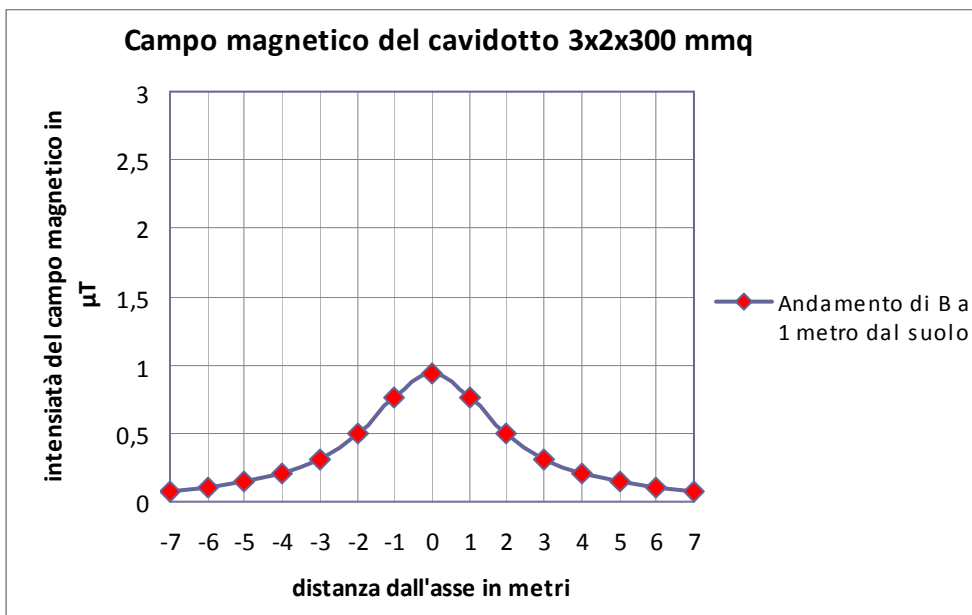
Figura 5 – Campo magnetico cavidotto 3x2x300mmq ad 1 m dal suolo.
