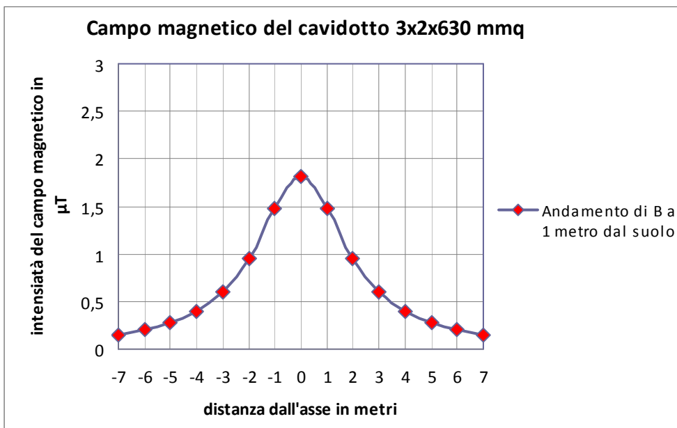
Figura 9 – Campo magnetico cavidotto 3x2x630mmq ad 1 m dal suolo.
