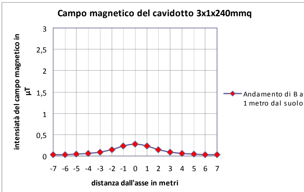
Figura 3 – Campo magnetico cavidotto 3x1x240mmq ad 1m dal suolo.
