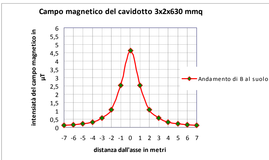
Figura 10 Campo magnetico cavidotto 3x2x630mmq al suolo.
