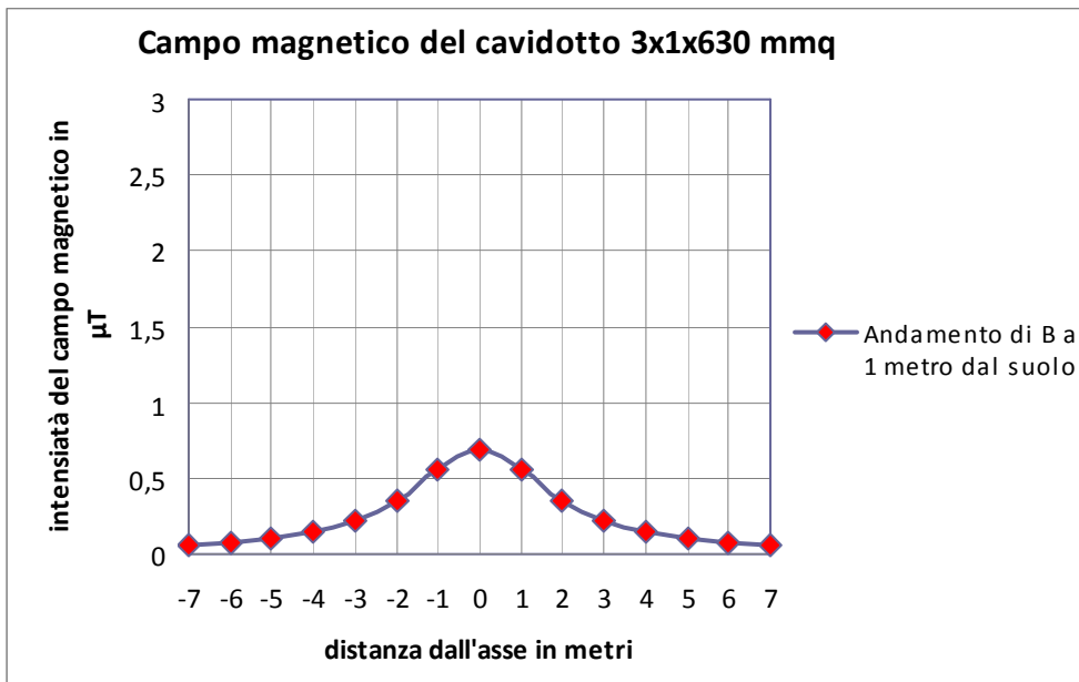
Figura 7 – Campo magnetico cavidotto 3x1x630mmq ad 1 m dal suolo.
