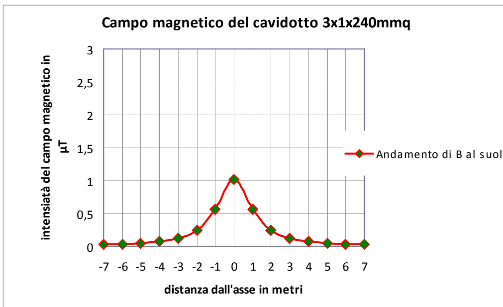
Figura 4 Campo magnetico cavidotto 3x1x240mmq al suolo
