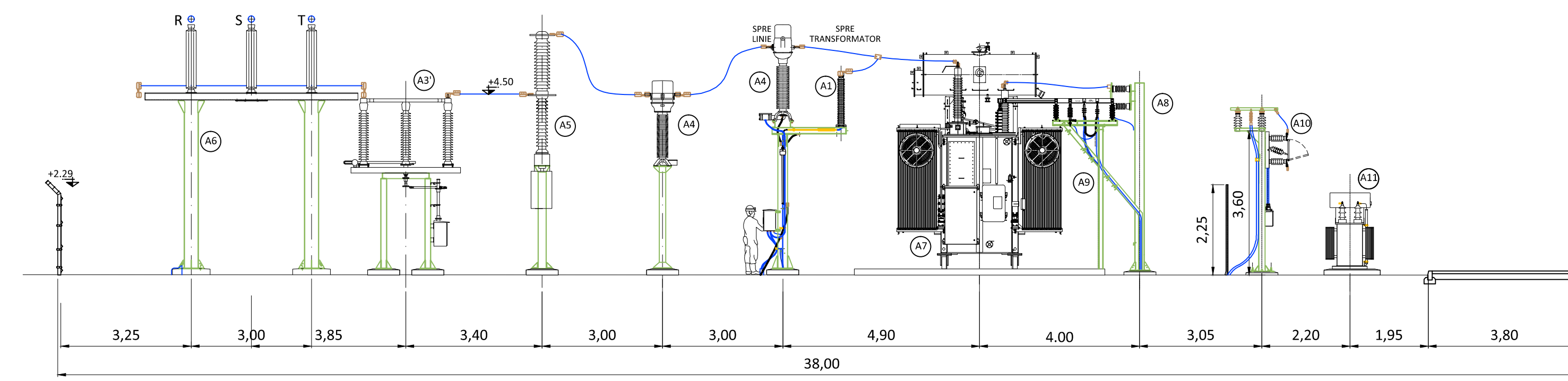
SEZIONE A-A
