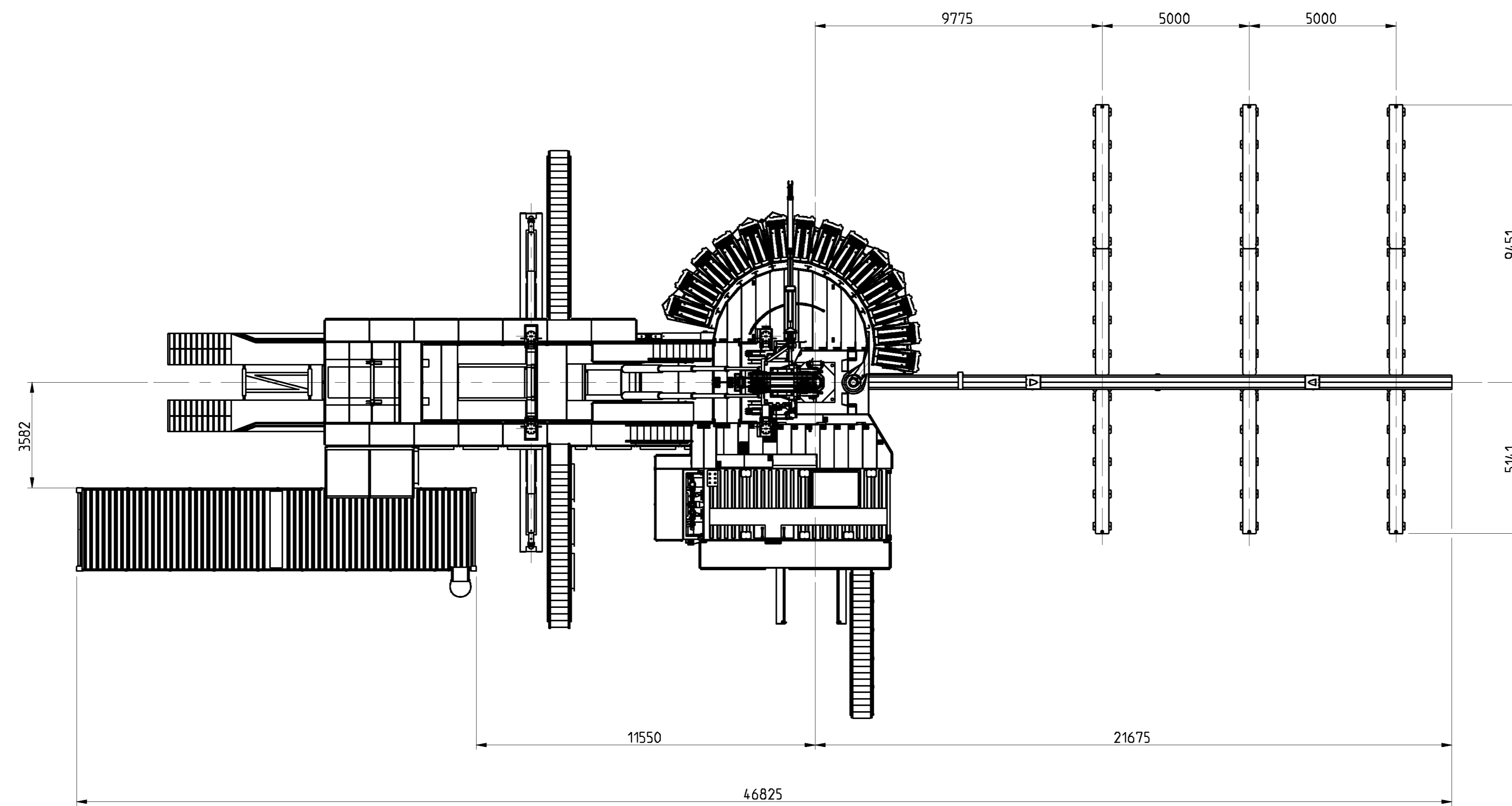
IMPIANTO DI PERFORAZIONE DRILL MEC HH200 MM: VISTA IN PIANTA
