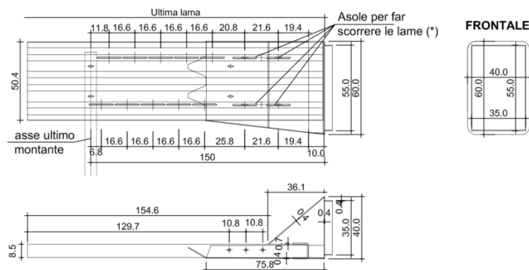
Figura 3: elemento terminale di fine impianto (tradizionale “a manina” non ammesso in progetto a sx e soluzione prevista in PE a dx)
