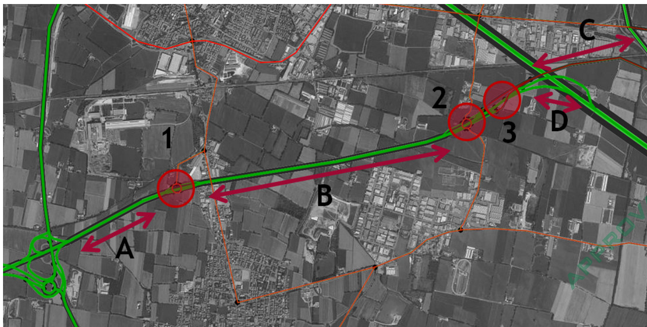
Schema dei Tronchi stradali dello studio di traffico
