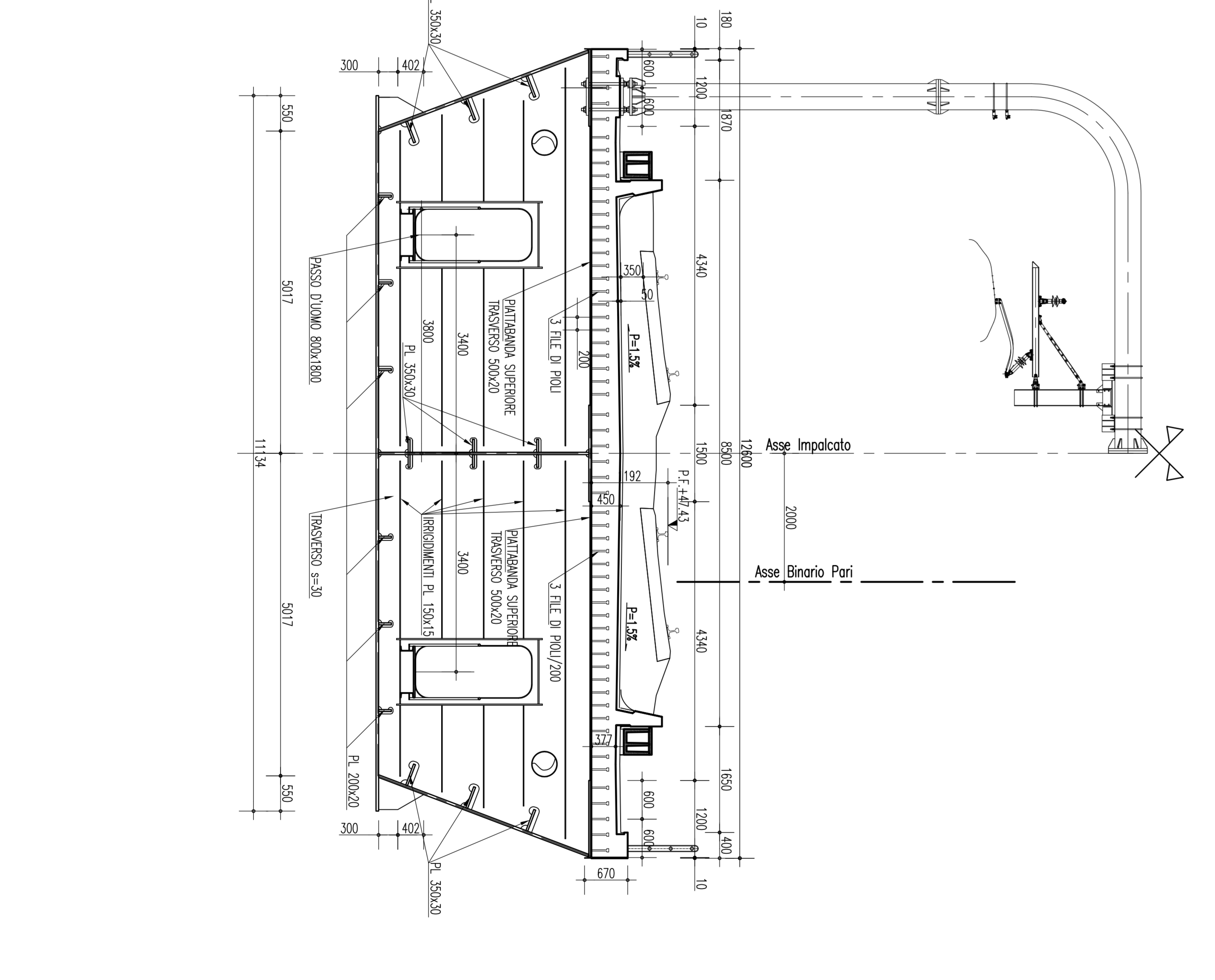
SEZIONE TRASVERSALE SUGLI APPOGGI SPALLA B SCALA 1:50
