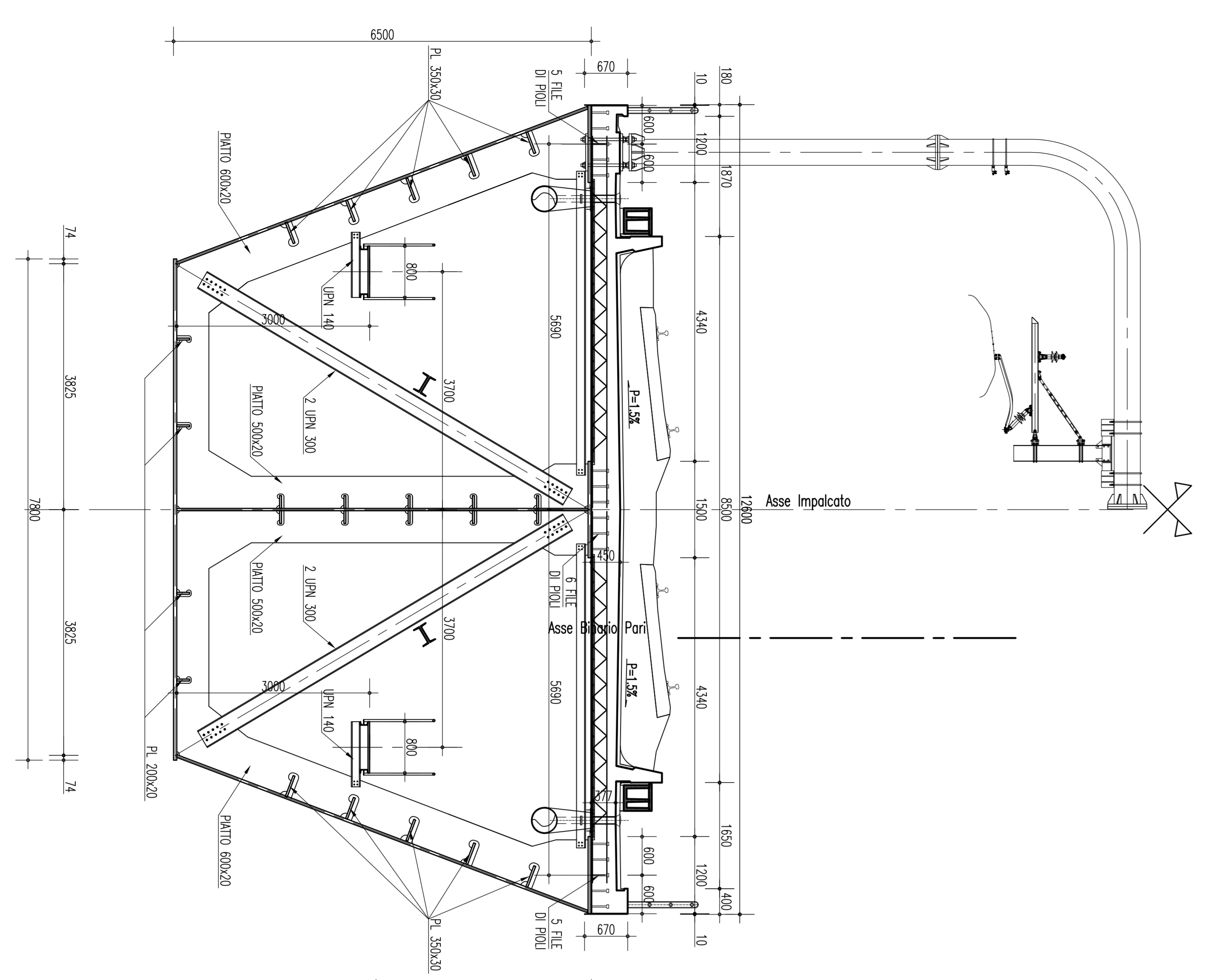
SEZIONE TRASVERSALE IN MEZZERIA SCALA 1:50
