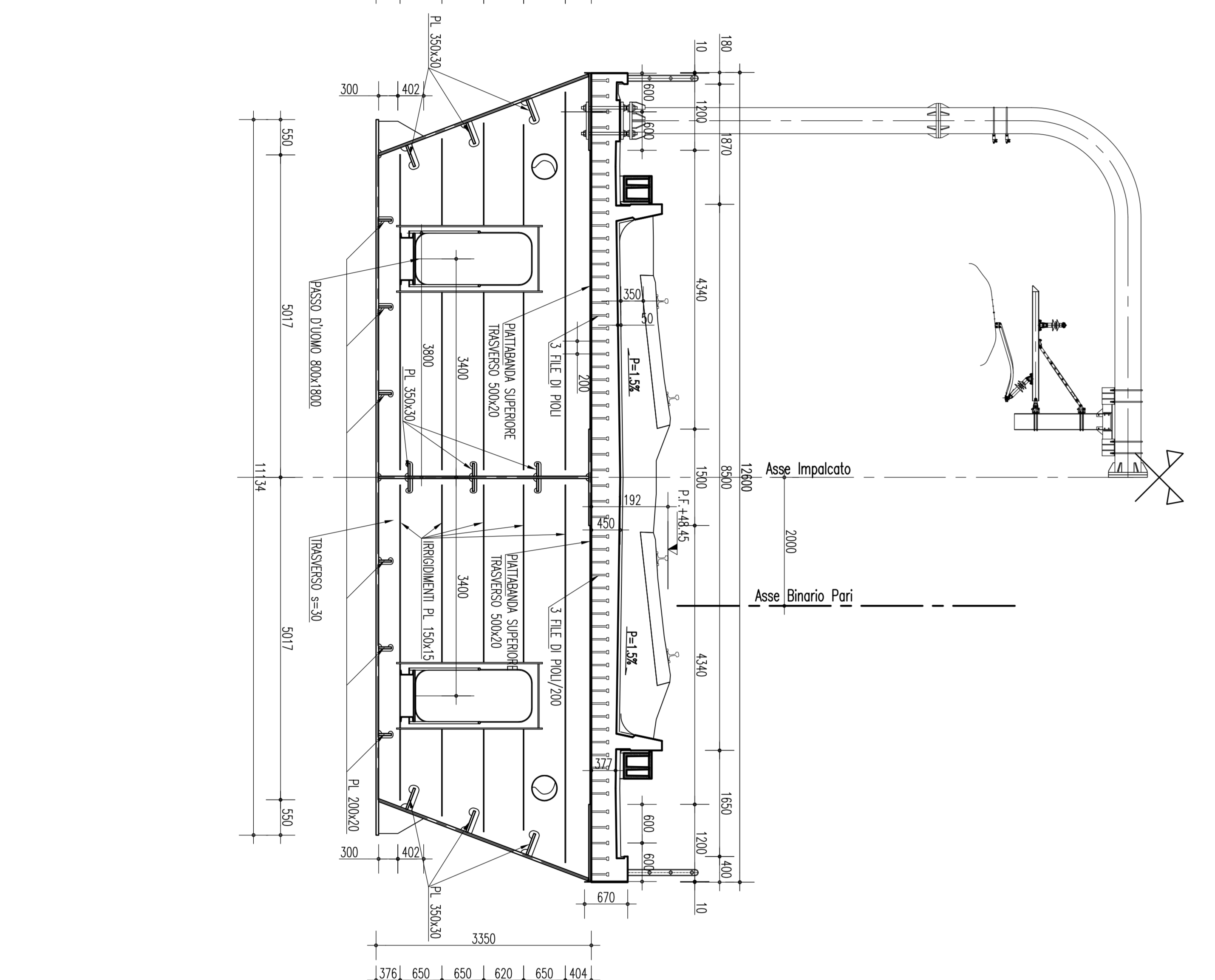
SEZIONE TRASVERSALE SUGLI APPOGGI PILA 5 SCALA 1:50
