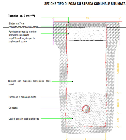
Figura 3.5 – Condotte su strada comunale
