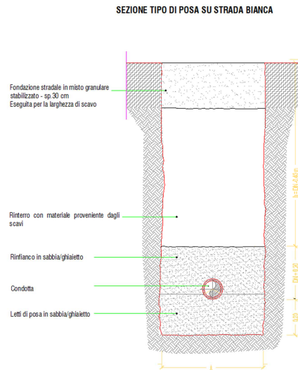
Figura 3.4 – Condotte su strada bianca
