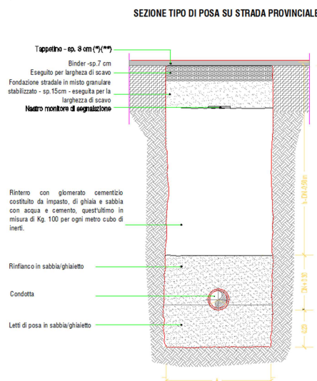
Figura 3.6 – Condotte su strada provinciale
