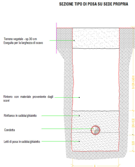
Figura 3.3 – Condotte in sede propria
