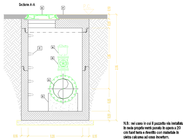
Figura 3.2 – Pozzetti di linea su strada
