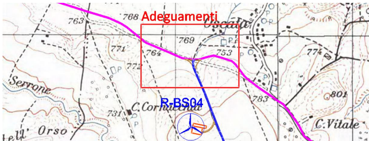
Figura 11: adeguamenti dell'accesso dalla SP 189 da prevedersi sia sul lato destro che sinistro della viabilità imbrecciata esistente.
