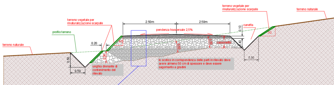
Figura 3: sezione tipo della viabilità da realizzare o adeguare
