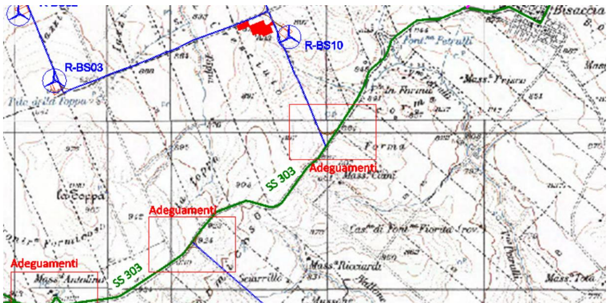
Figura 10: adeguamenti degli accessi dalla SS 303.
