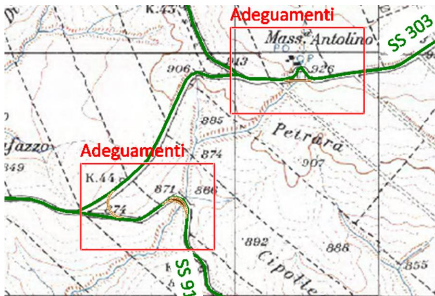
Figura 4: adeguamenti lungo la viabilità principale dell'area (SS 91 e SS 303).
