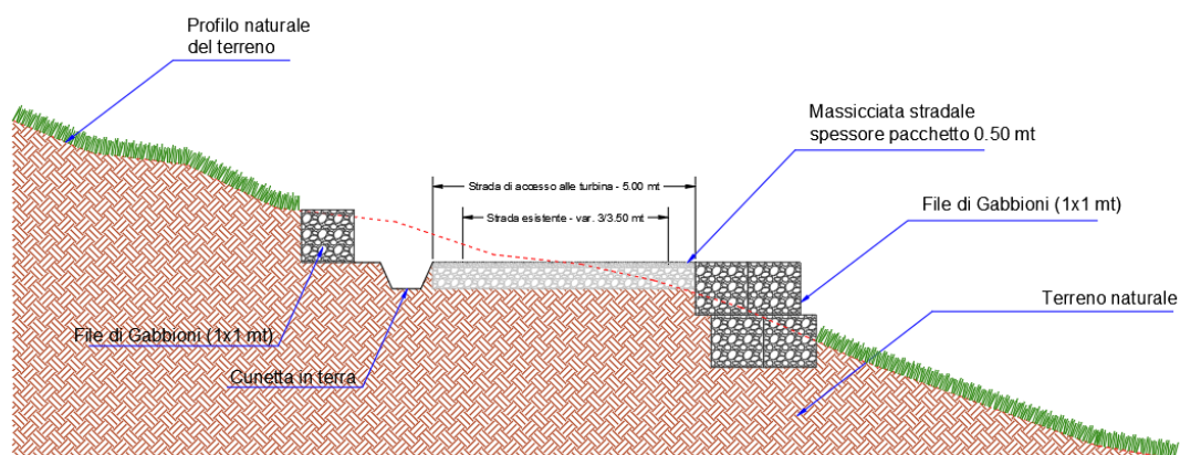
Figura 14: sezione tipo del tratto della strada di collegamento tra dell'aerogeneratore R-BS07 e R-BS08 ove ci sono le pendenze trasversali più elevate
