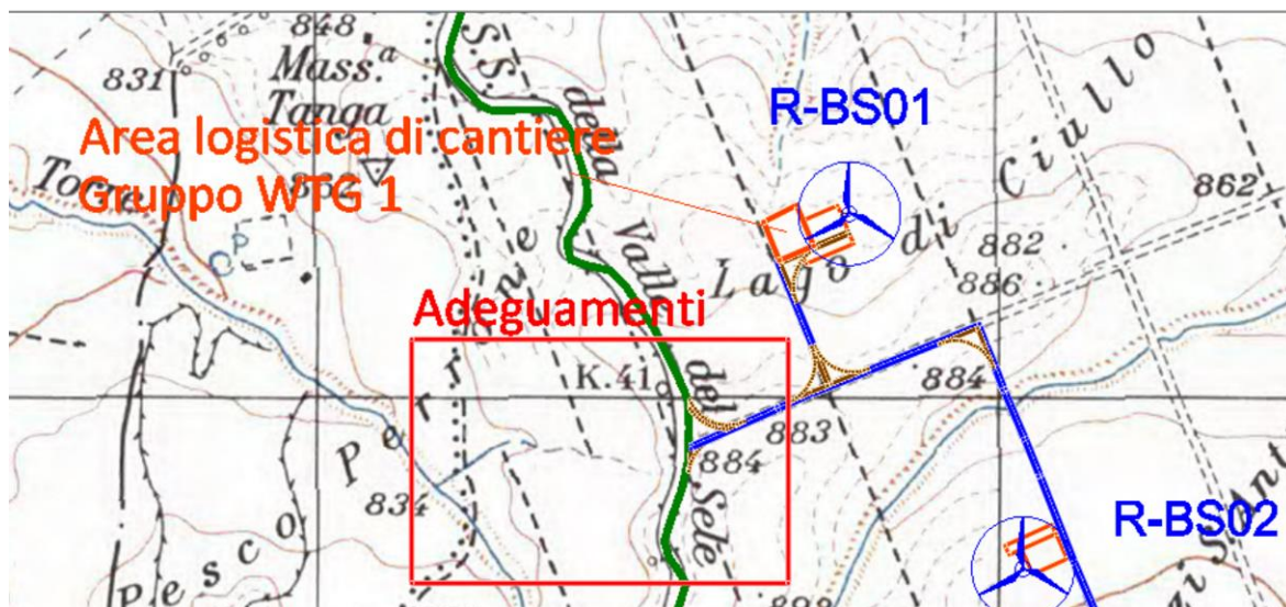
Figura 8: adeguamenti dell'accesso dalla SS 91.
