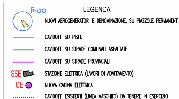
Figura 19: Stralcio planimetrie tracciato cavidotti
