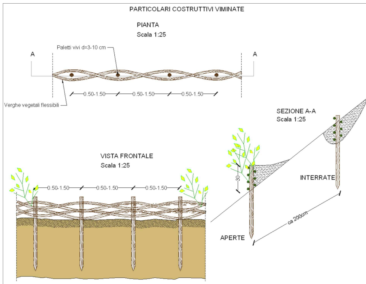
Figura 15: Esempio di vimate per stabilizzazione superficiale.
