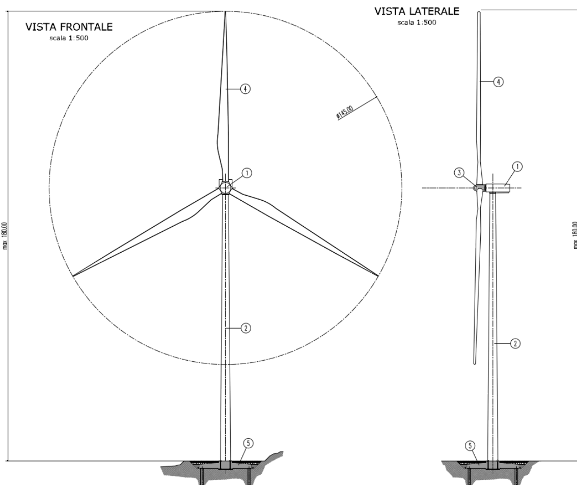
Figura 5: Schema tipo aerogeneratore
