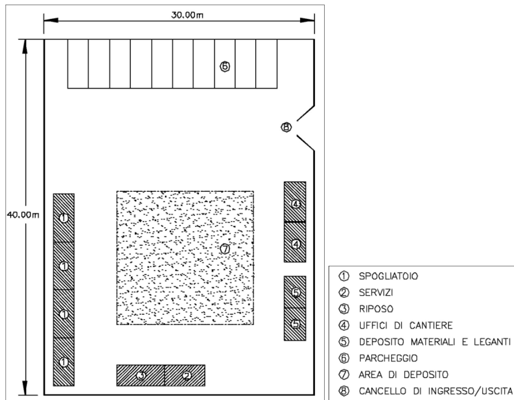
Figura 24: Planimetria area di cantiere.
