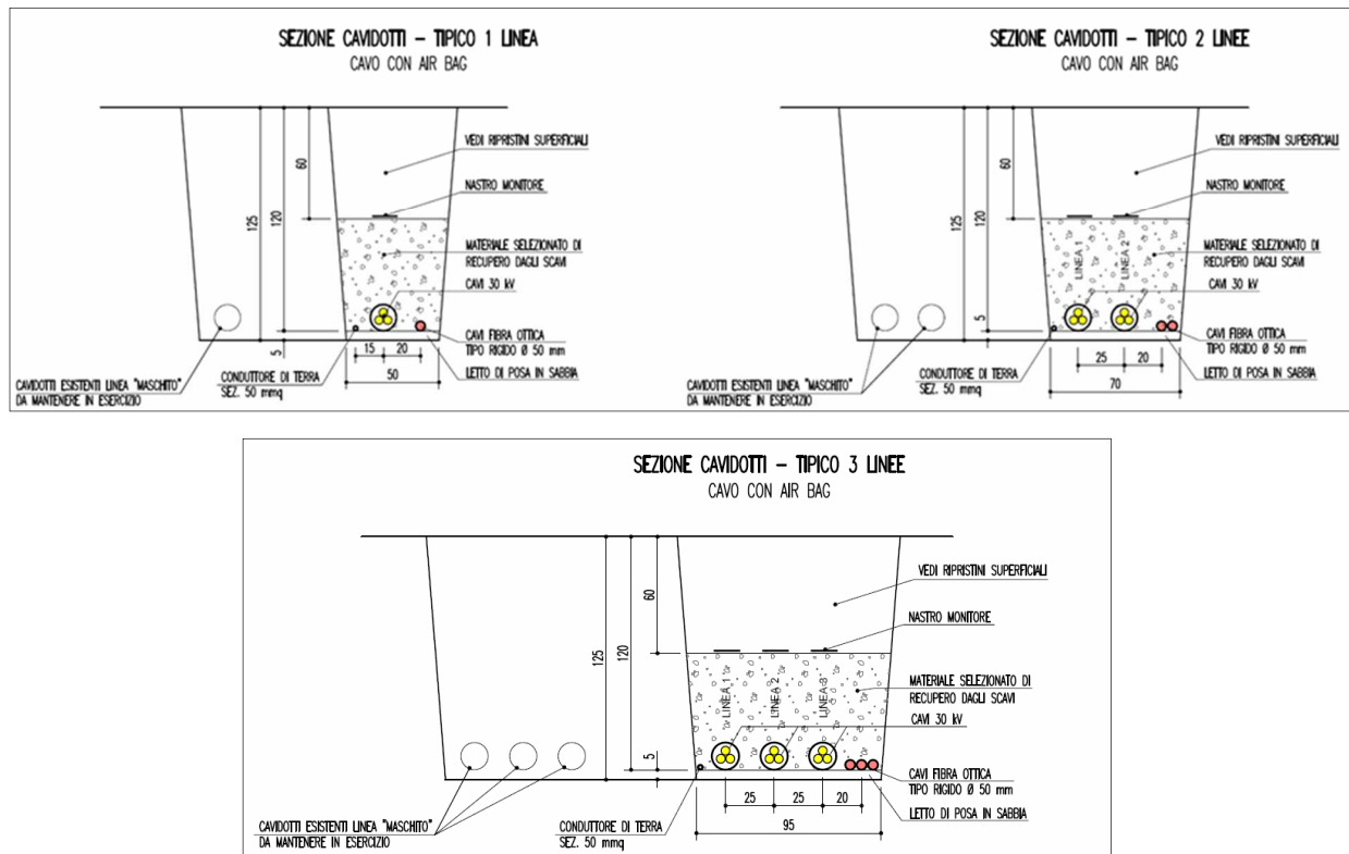
Figura 20: Sezioni tipo cavidotti.
