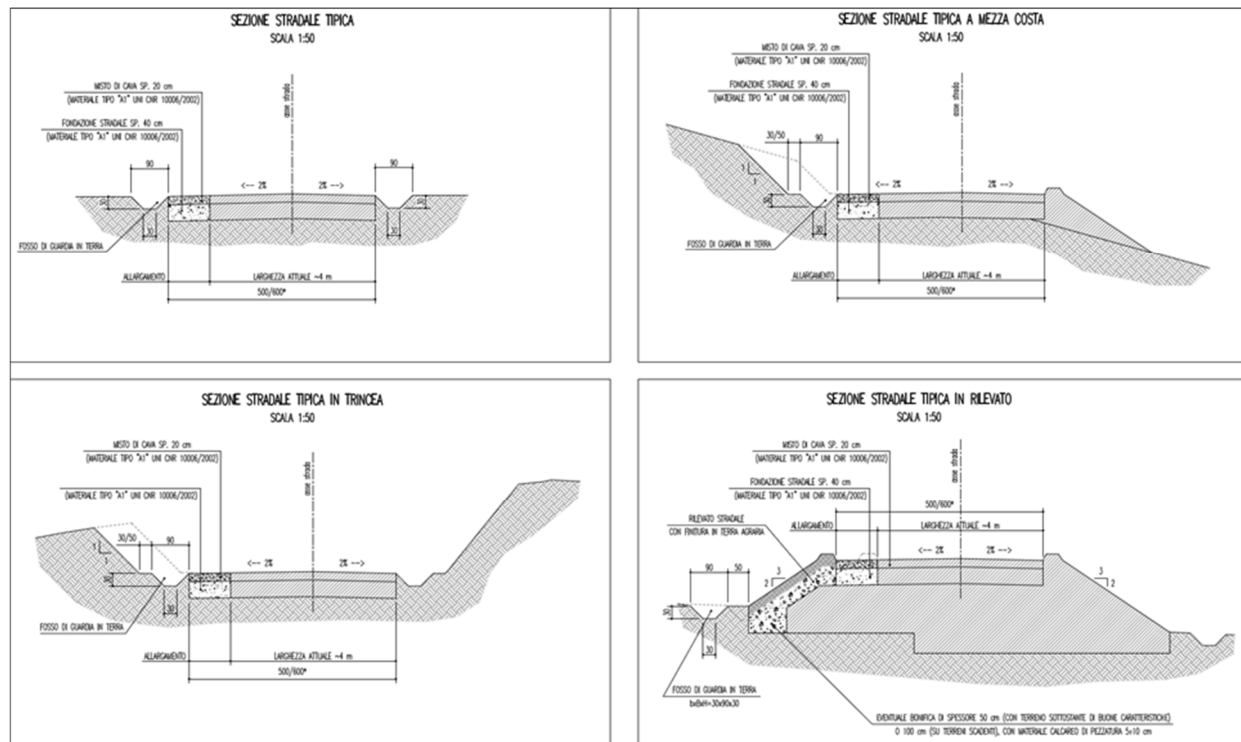
Figura 12: Sezioni stradali.
