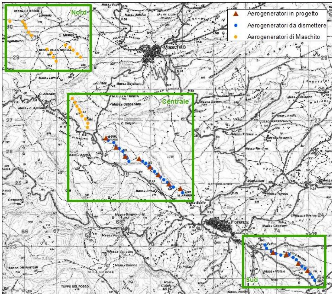
Figura 2-1 – Layout dell'impianto esistente (blu per Foreza e giallo per Maschito) e di quello in progetto (rosso)
