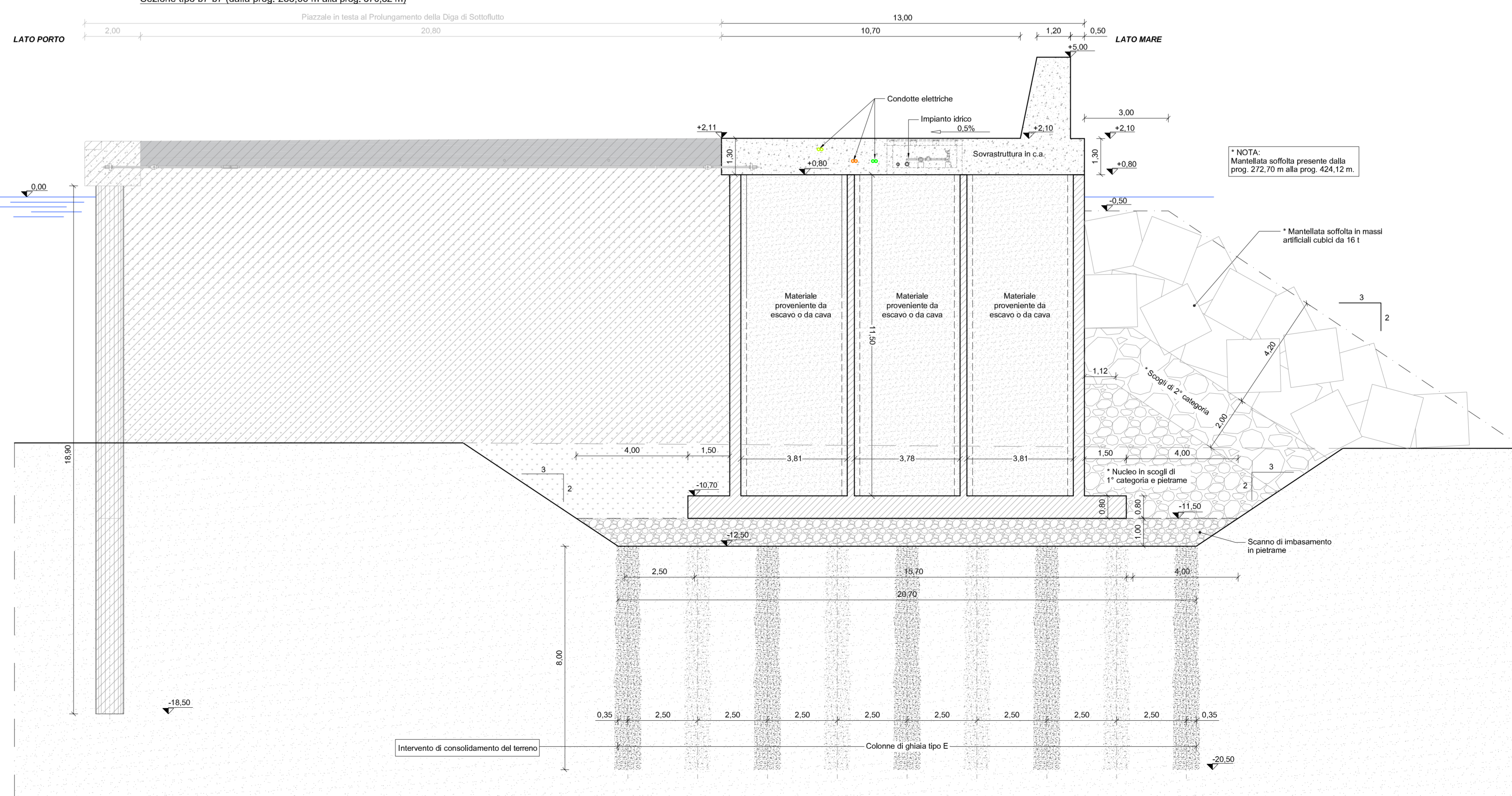
Sezione tipo b7-b7 (dalla prog. 283,86 m alla prog. 370,32 m)
