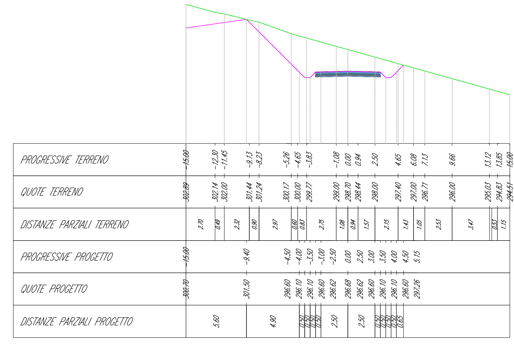
Tracciato BC - Sez. 35 - Progr. 1+700.00 Scala 1:200 Q.Rit. 290.00m
