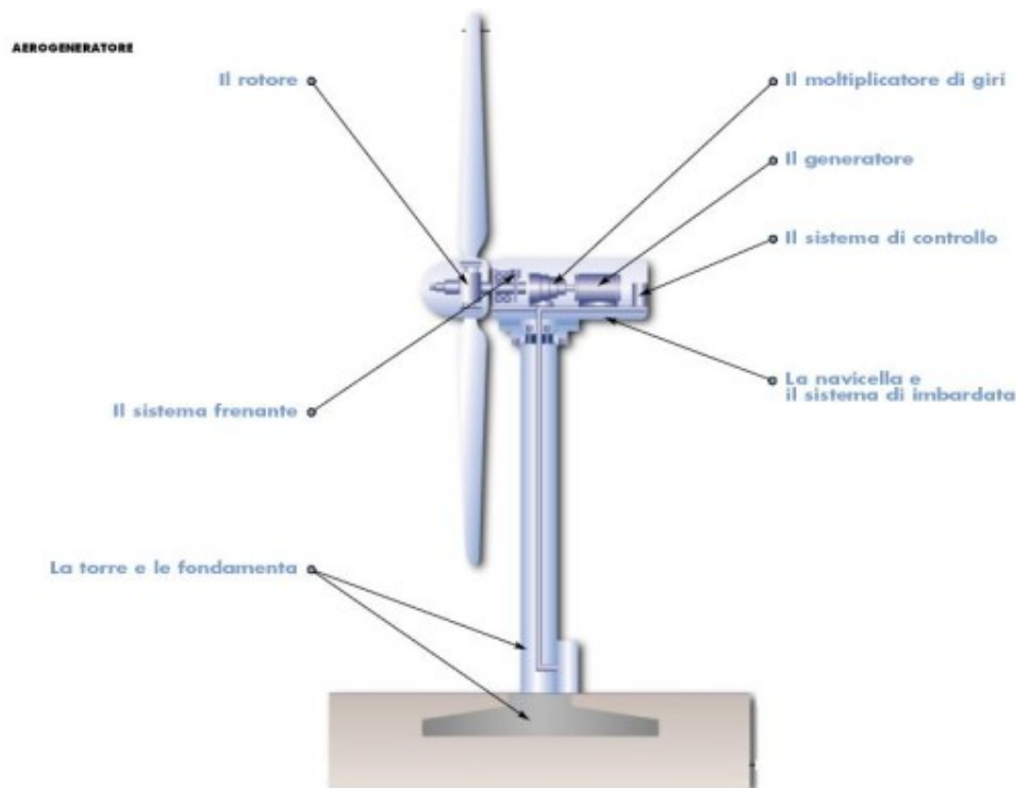
Figura 1 – Schematizzazione aerogeneratore
