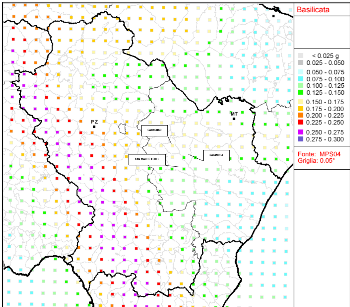
Figura 1 – Stralcio della mappa di pericolosità sismica del territorio nazionale
