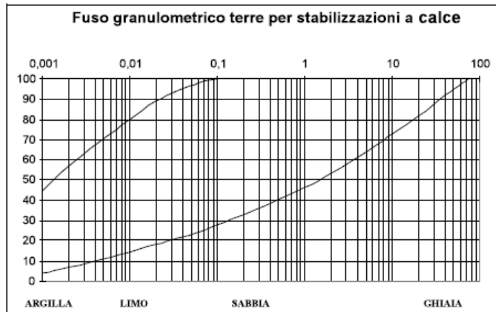
Figura 1 - Fuso granulometrico di riferimento (CNR-UNI 10006:2002).
