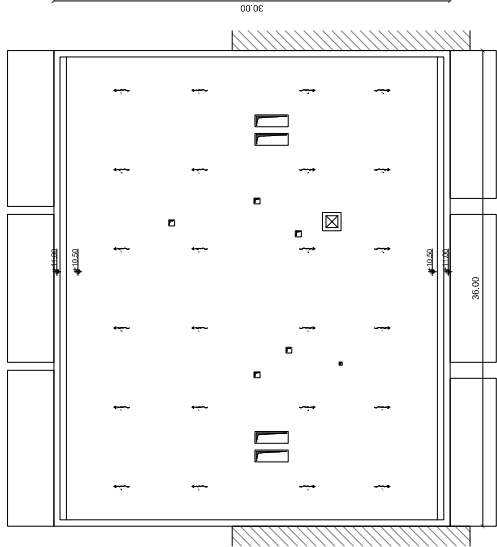
PIANTA COPERTURA
