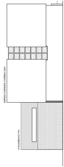
PROSPETTO SUD
