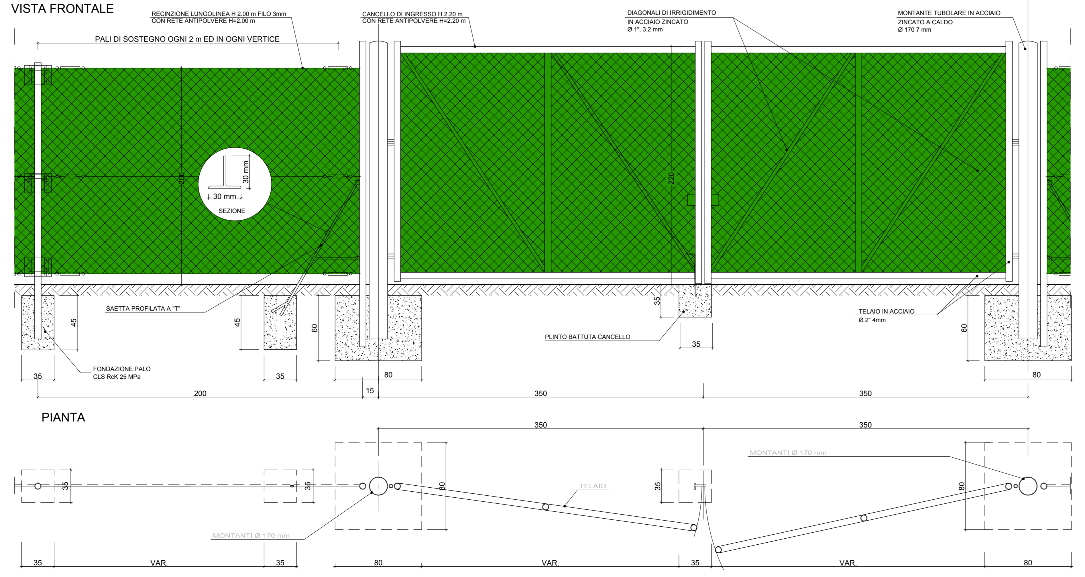
RECINZIONE A MAGLIA SCIOLTA E CANCELLO PASSO CARRABILE scala 1:20
