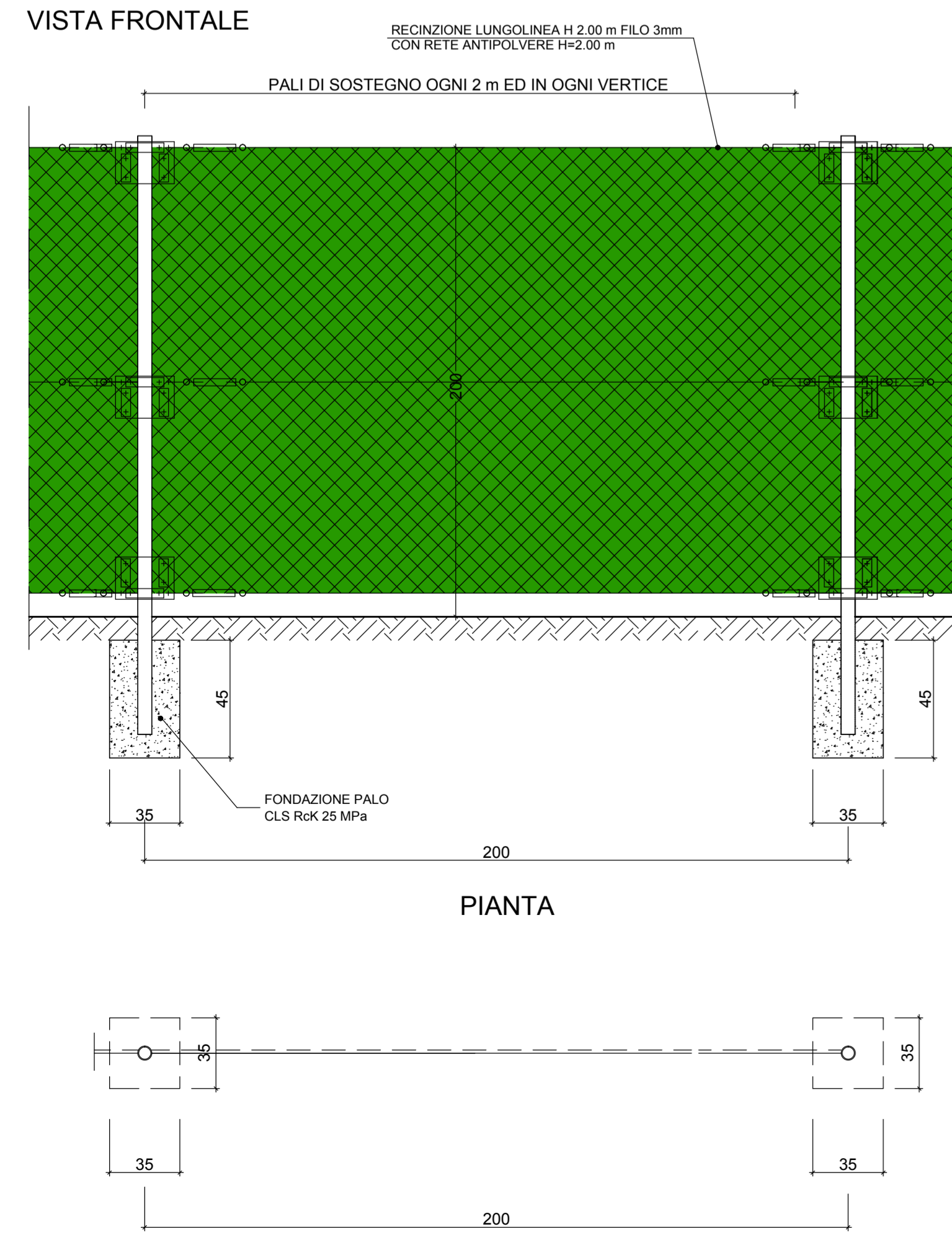
RECINZIONE A MAGLIA SCIOLTA scala 1:20
