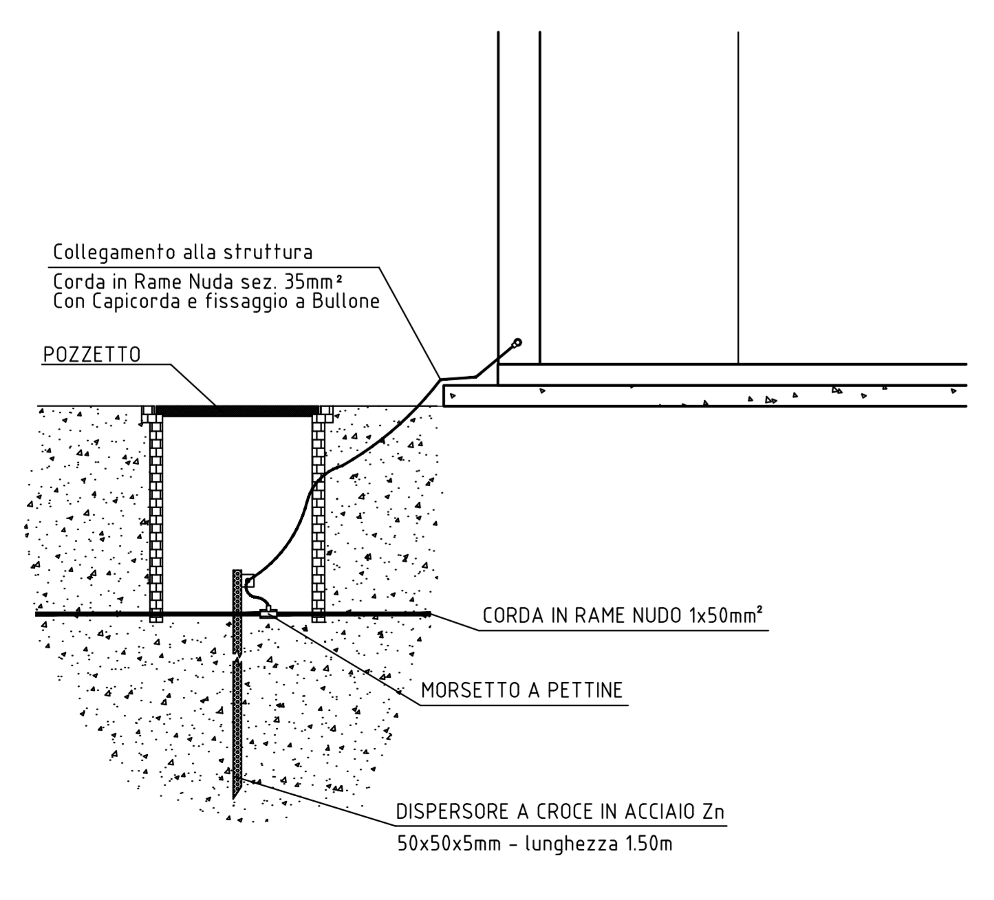
TIPICO COLLEGAMENTO A TERRA DELLE STRUTTURE
