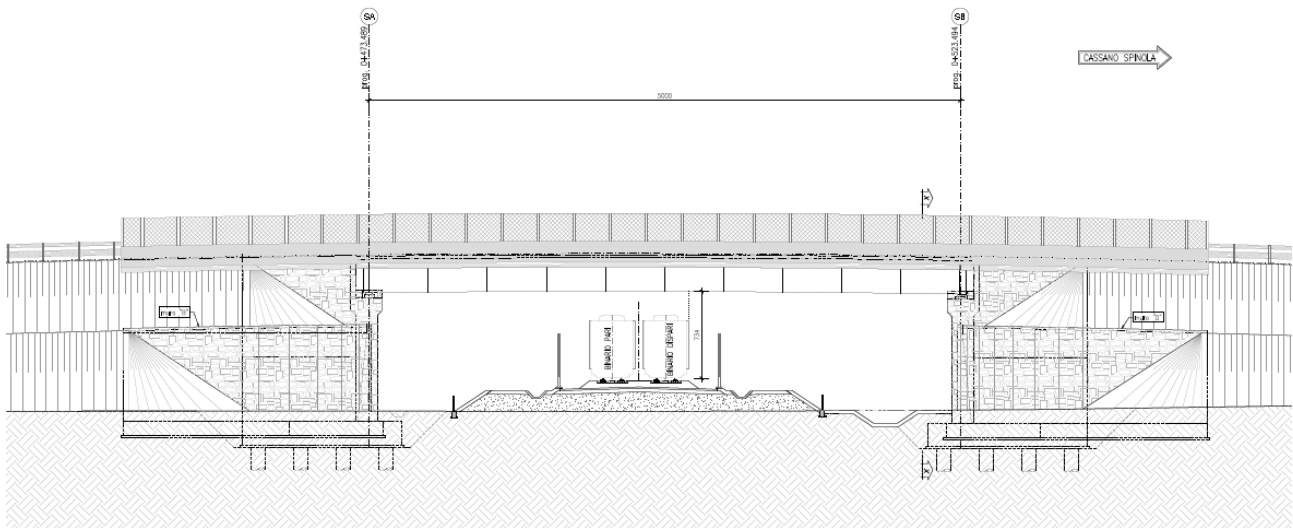
Figura 5 – sezione longitudinale opera
