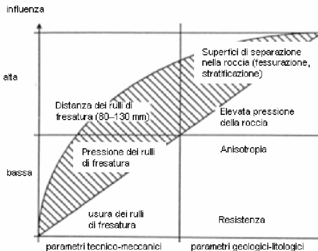
Figura 20 - Influenza sulla pezzatura del materiale di scavo nel caso di avanzamento con fresa TBM
