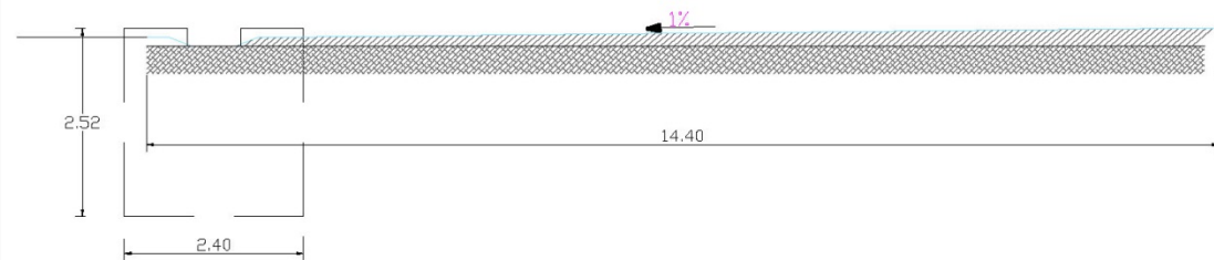
SEZIONE A-A
