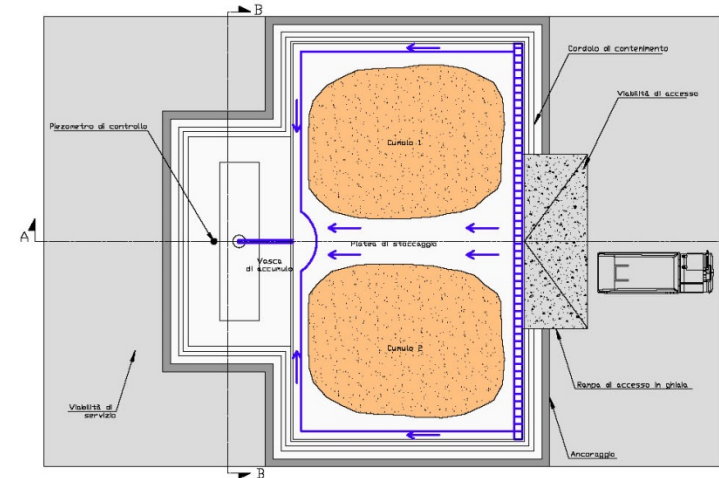
PLANIMETRIA PLATEA SINGOLA (scala 1:200)
