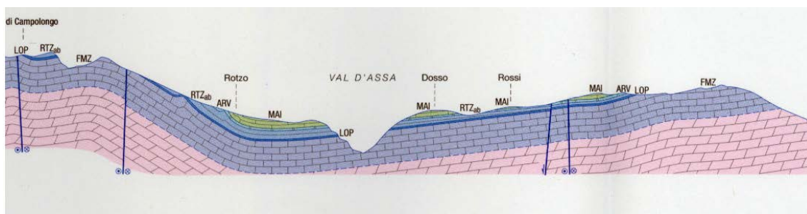
Figura 2 - Morfologia a plateau dell'altopiano della Valdastico e sequenza litologica caratteristica (tratto da "Carta Geologica d'Italia 1:50000, Regione Veneto, foglio 082 Asiago
