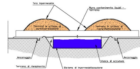
SEZIONE B - B Serbatoio interrato (scala 1:200)
