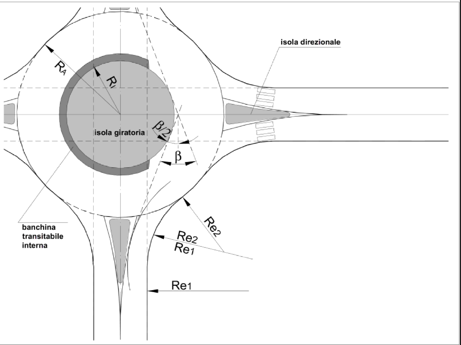
SCHEMA ANGOLO DI DEVIAZIONE DELLE TRAIETTORIE IN ROTATORIA (ANGOLO 8)
