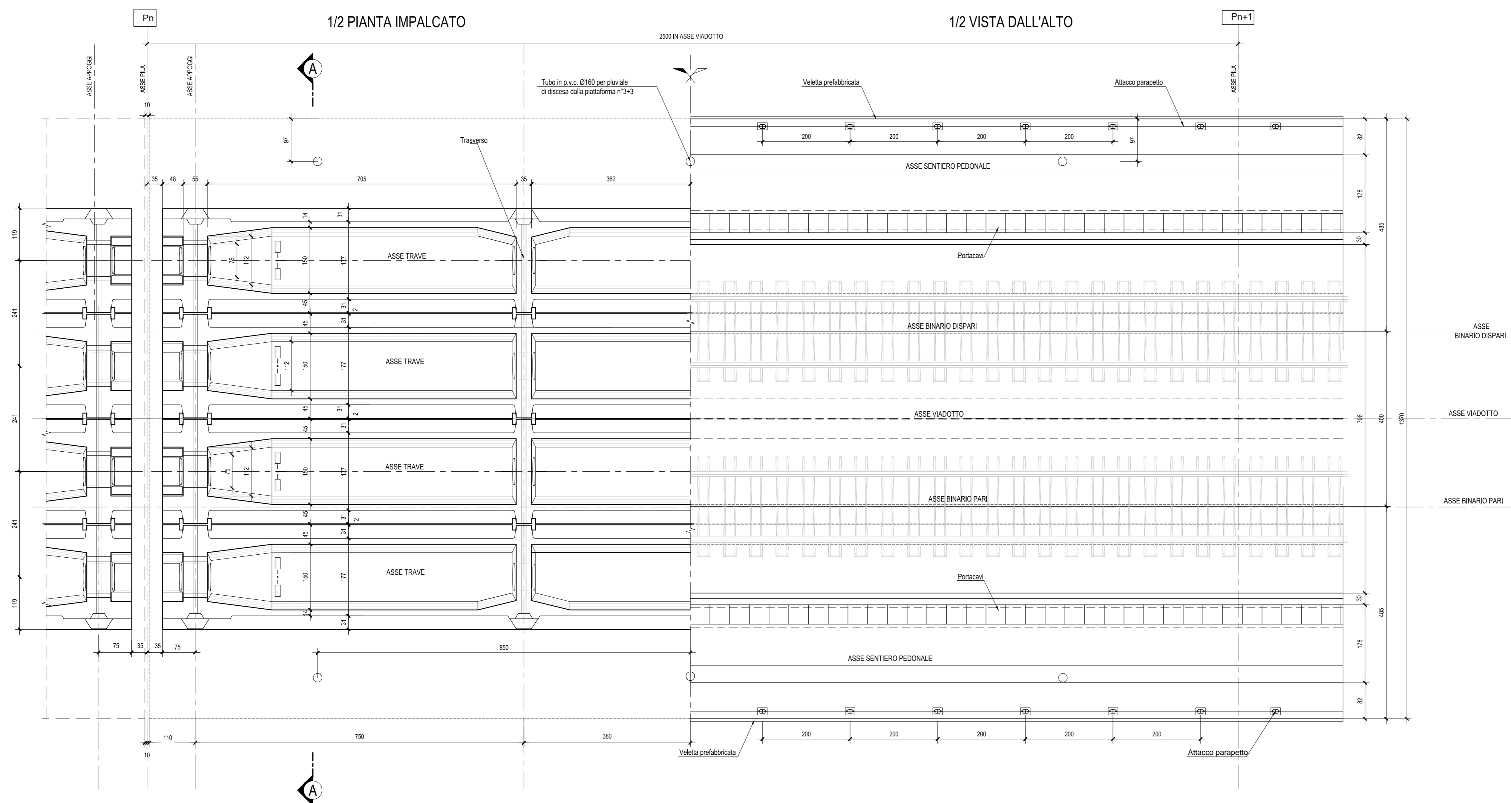
PIANTA IMPALCATO-Scala 1:50
