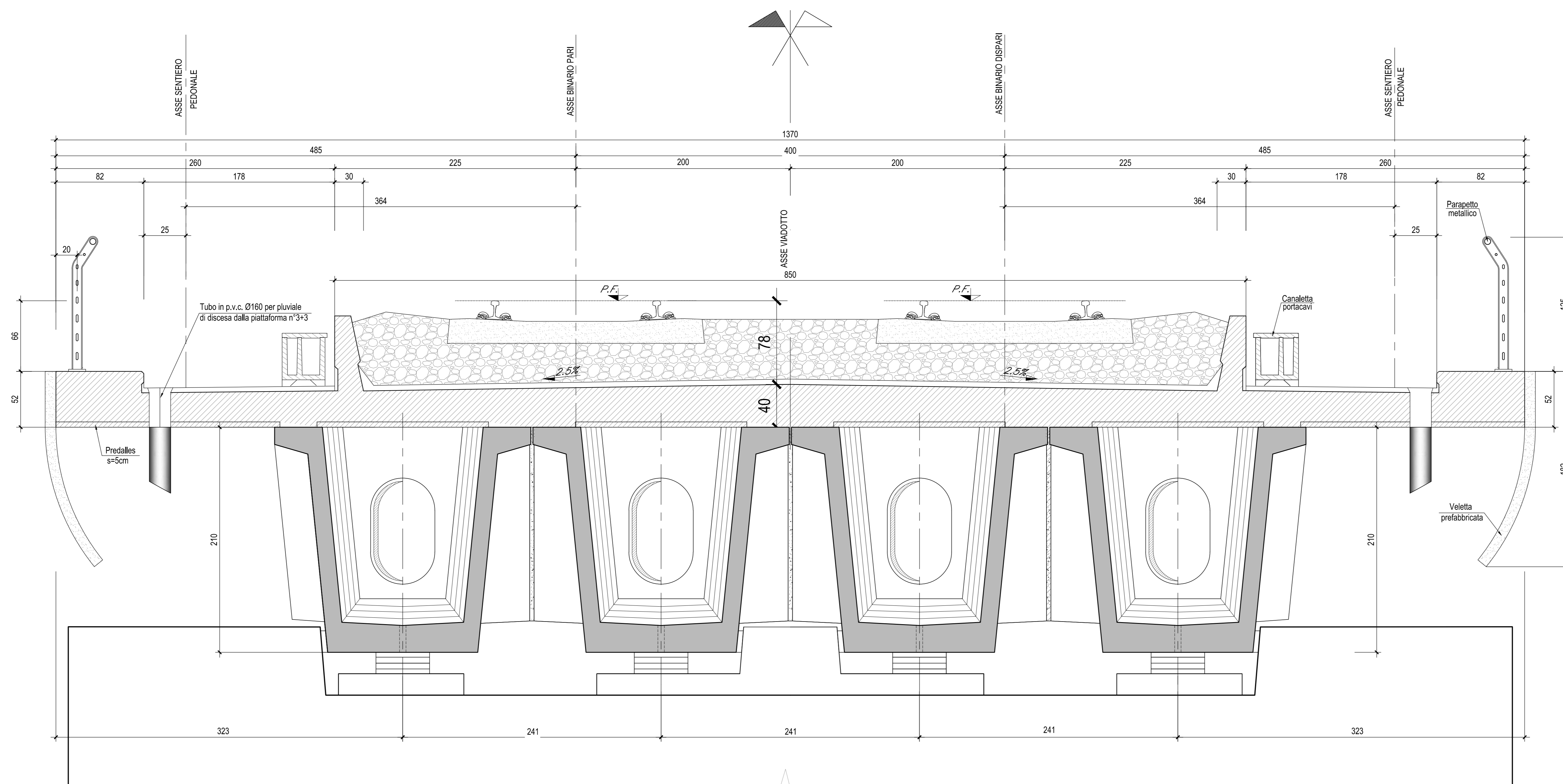
SEZIONE TRASVERSALE A-A-Scala 1:20
