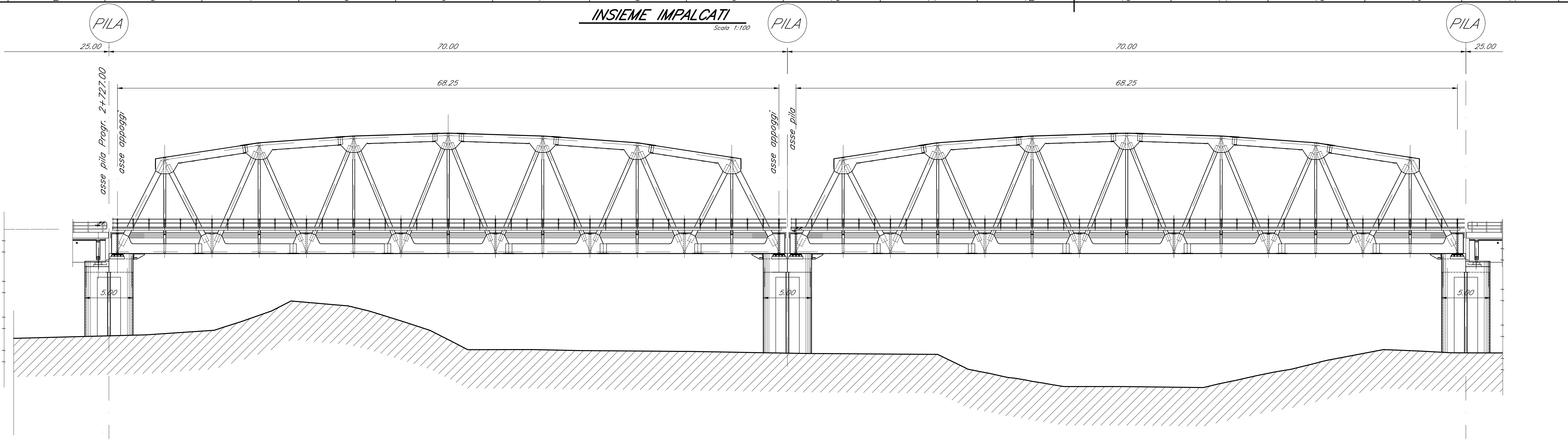
PROSPETTO IMPALCATO Scala 1:100
