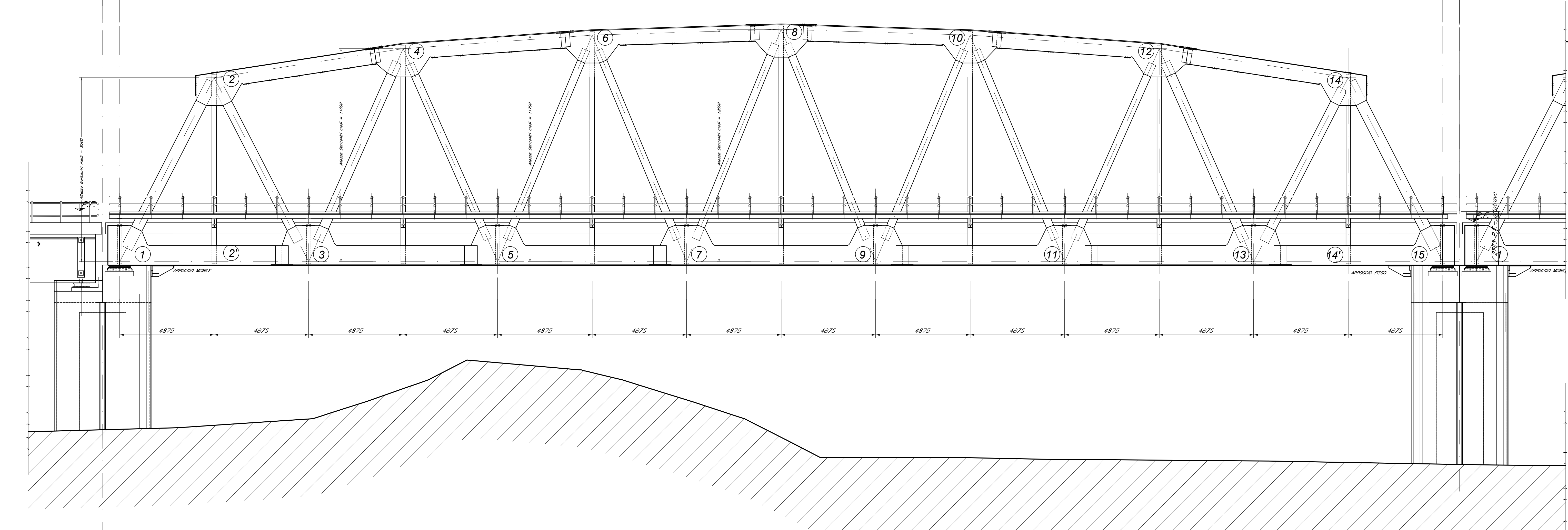
PROSPETTO IMPALCATO Scala 1:100
