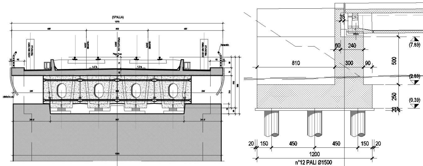
Figura 2 – Sezioni in direzione longitudinale e trasversale
