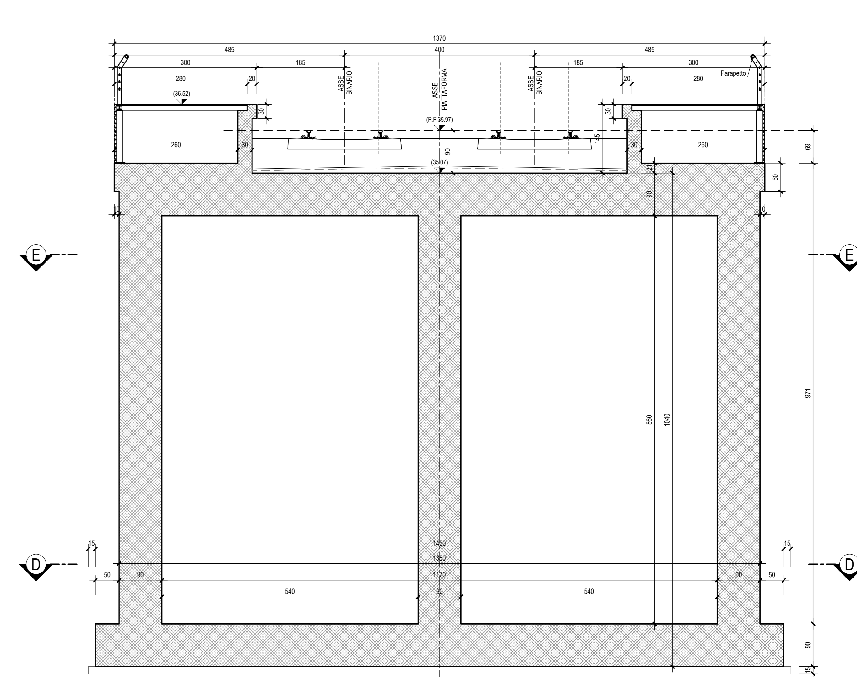
SEZIONE C-C-Scala 1:50
