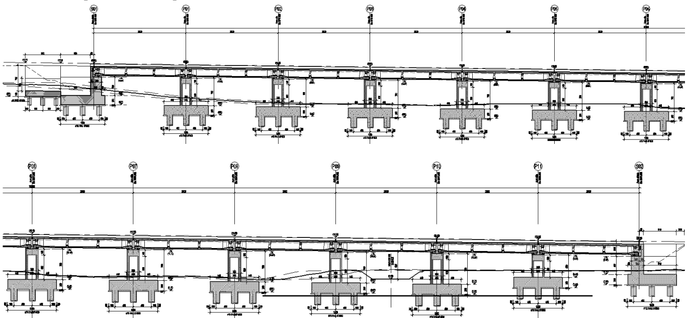
Figura 1 – Profilo longitudinale VI05
