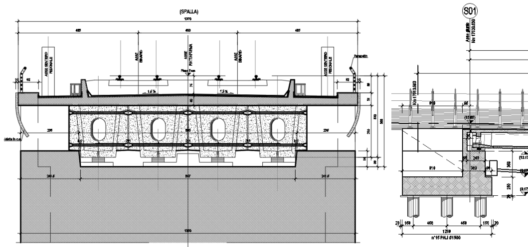
Figura 3 – Sezioni in direzione longitudinale e trasversale
