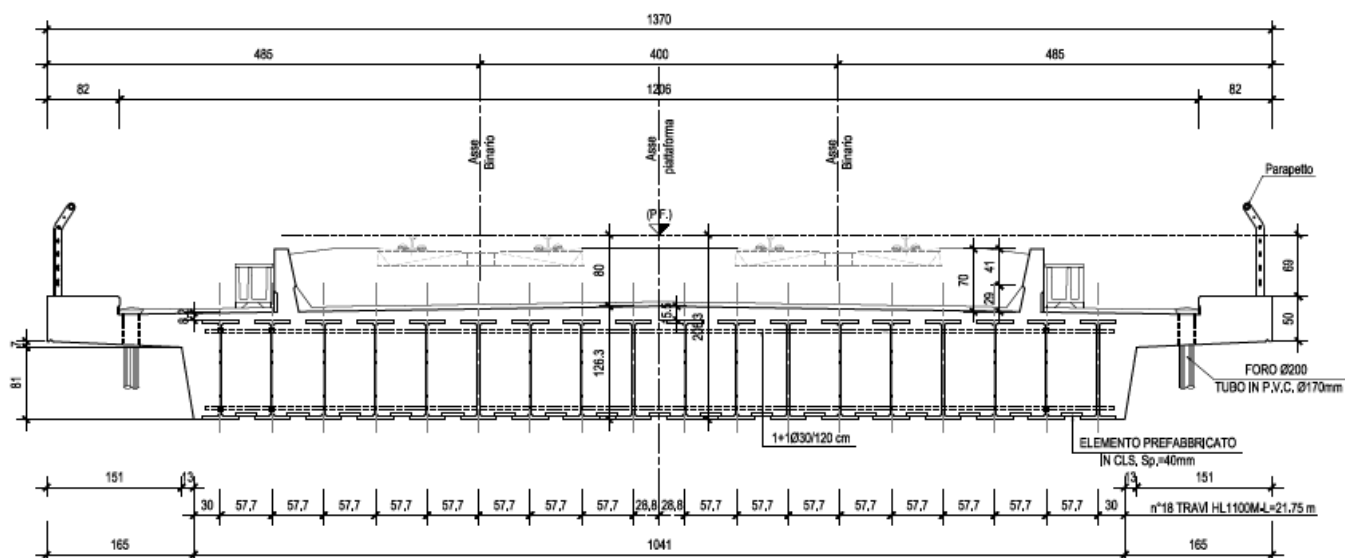
Figura 2 - Sezione trasversale impalcato
