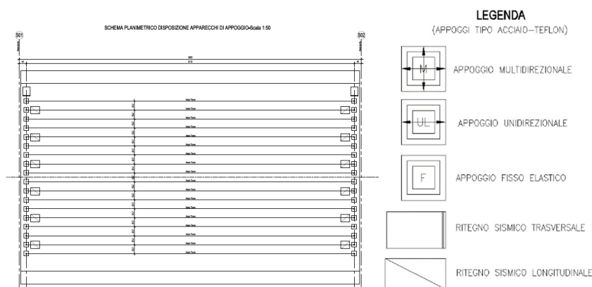
Figura 11 – Schema di appoggi travi incorporate
