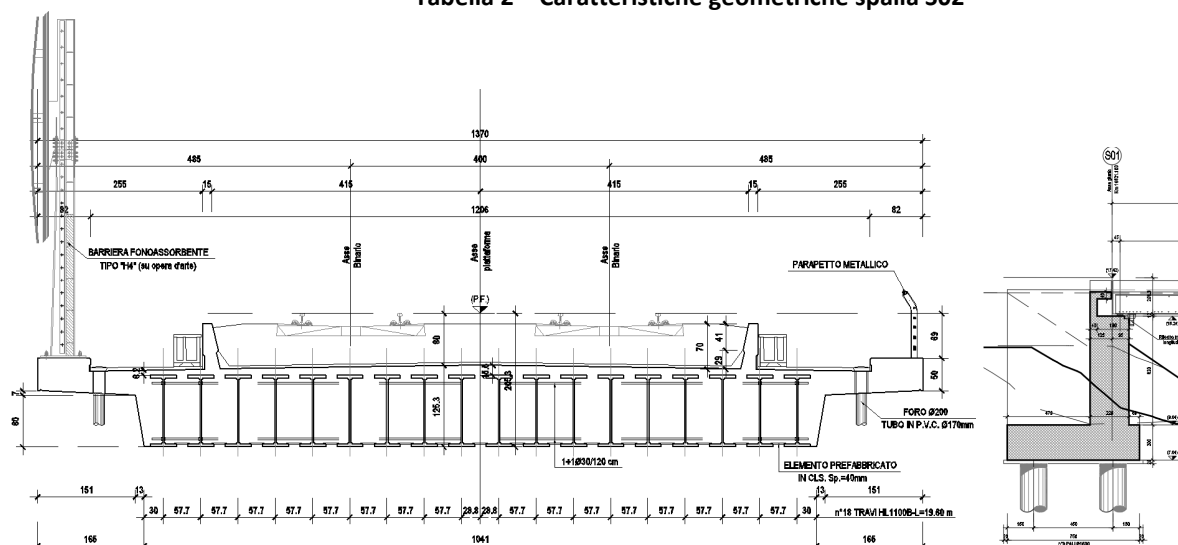
Figura 3 – Sezioni in direzione longitudinale e trasversale
