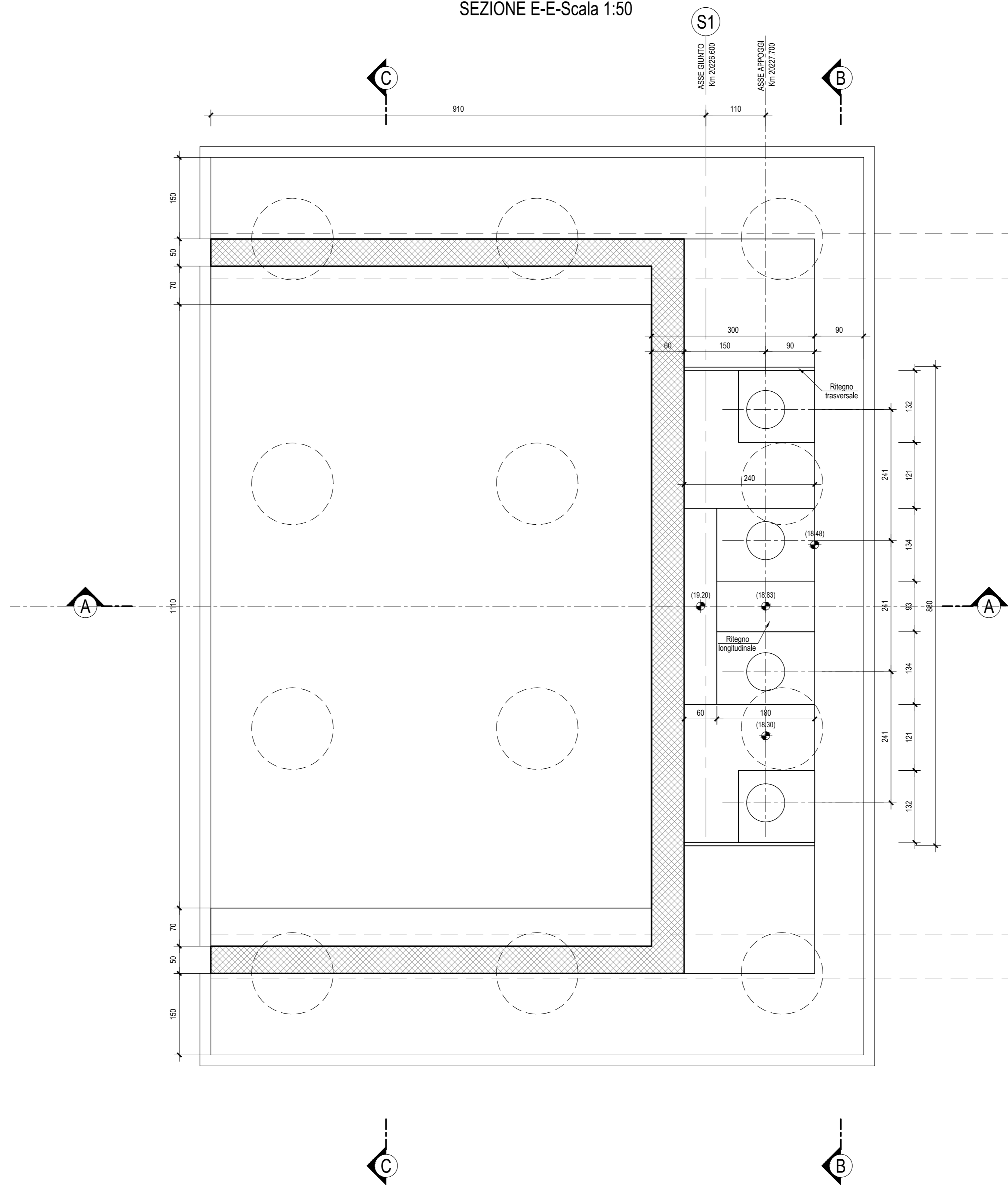
SEZIONE E-E-Scala 1:50
