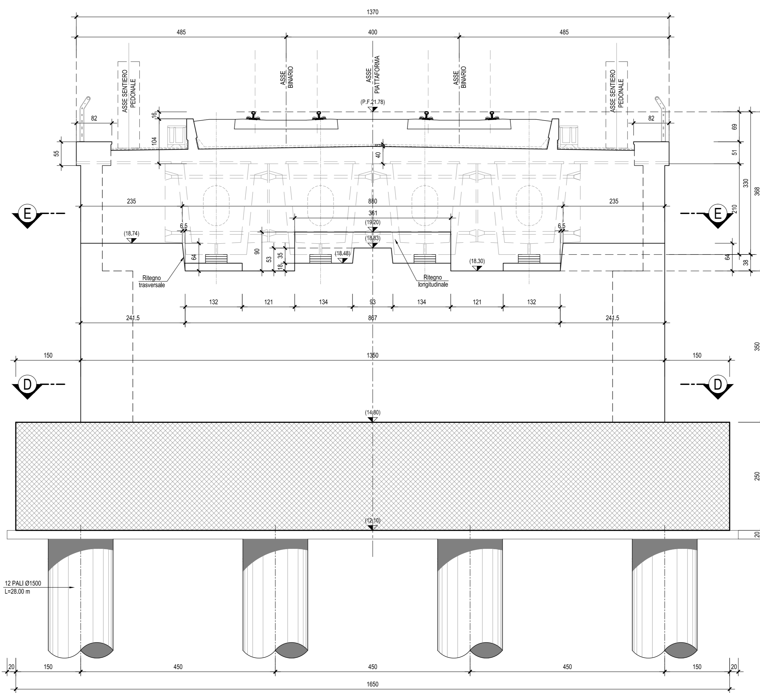
SEZIONE B-B-Scala 1:50
