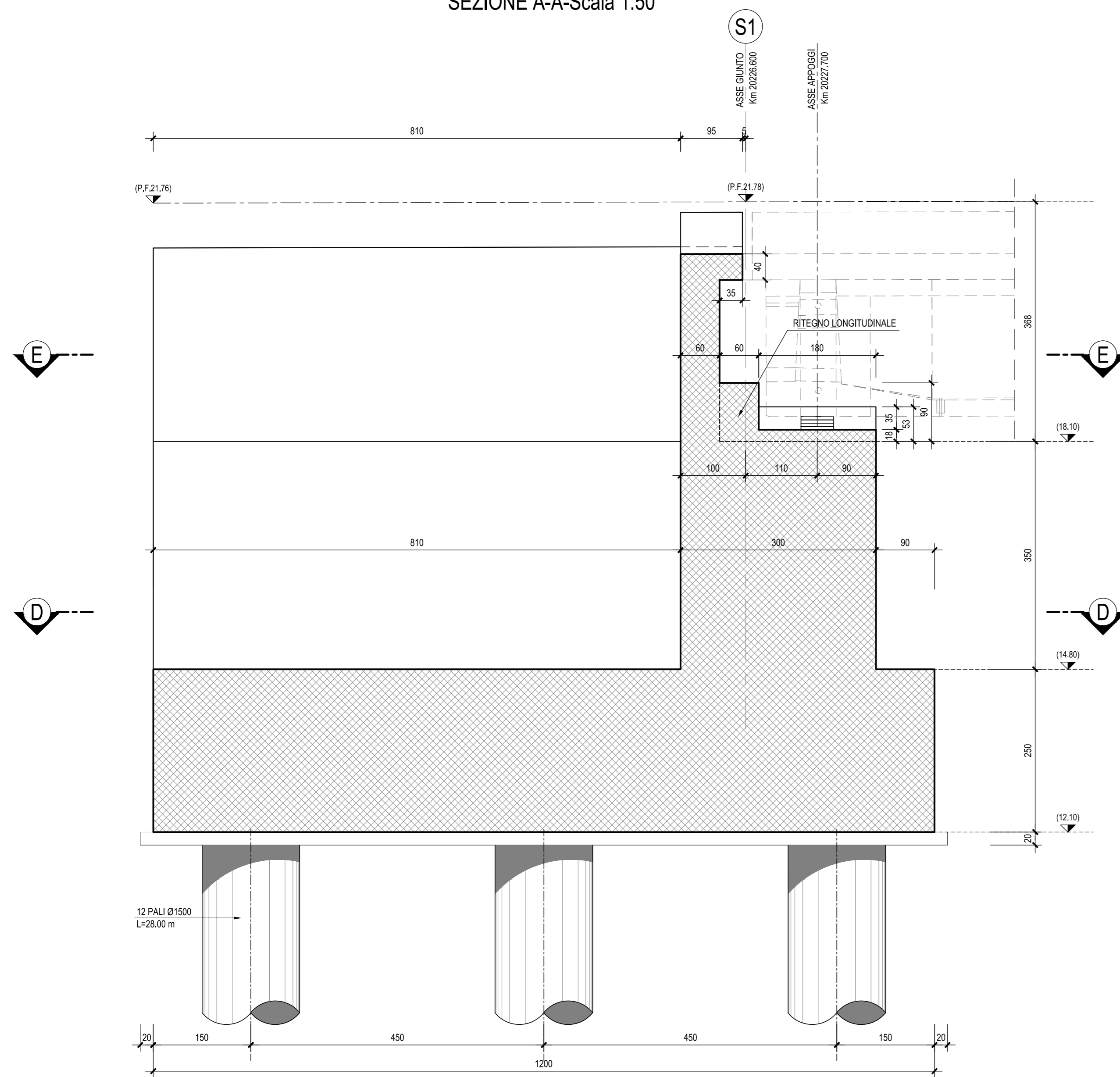
SEZIONE A-A-Scala 1:50
