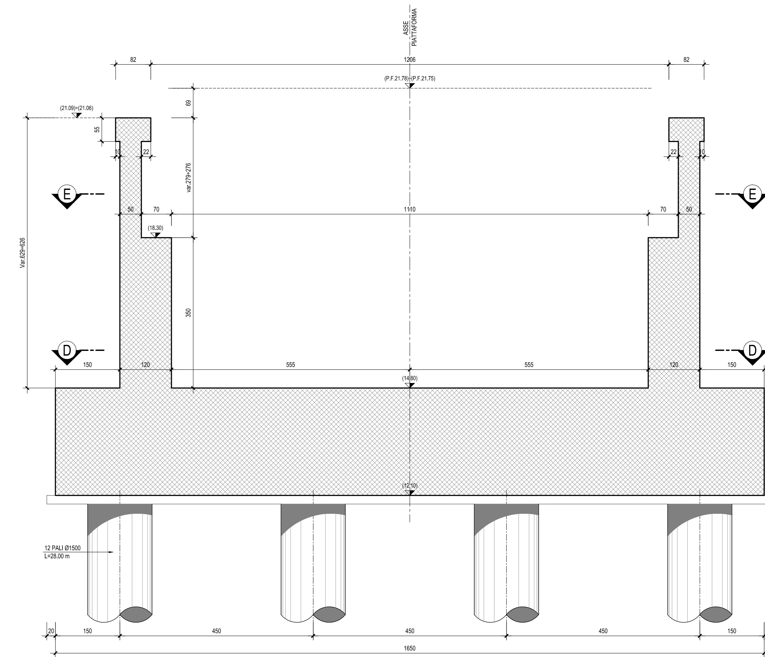
SEZIONE C-C-Scala 1:50
