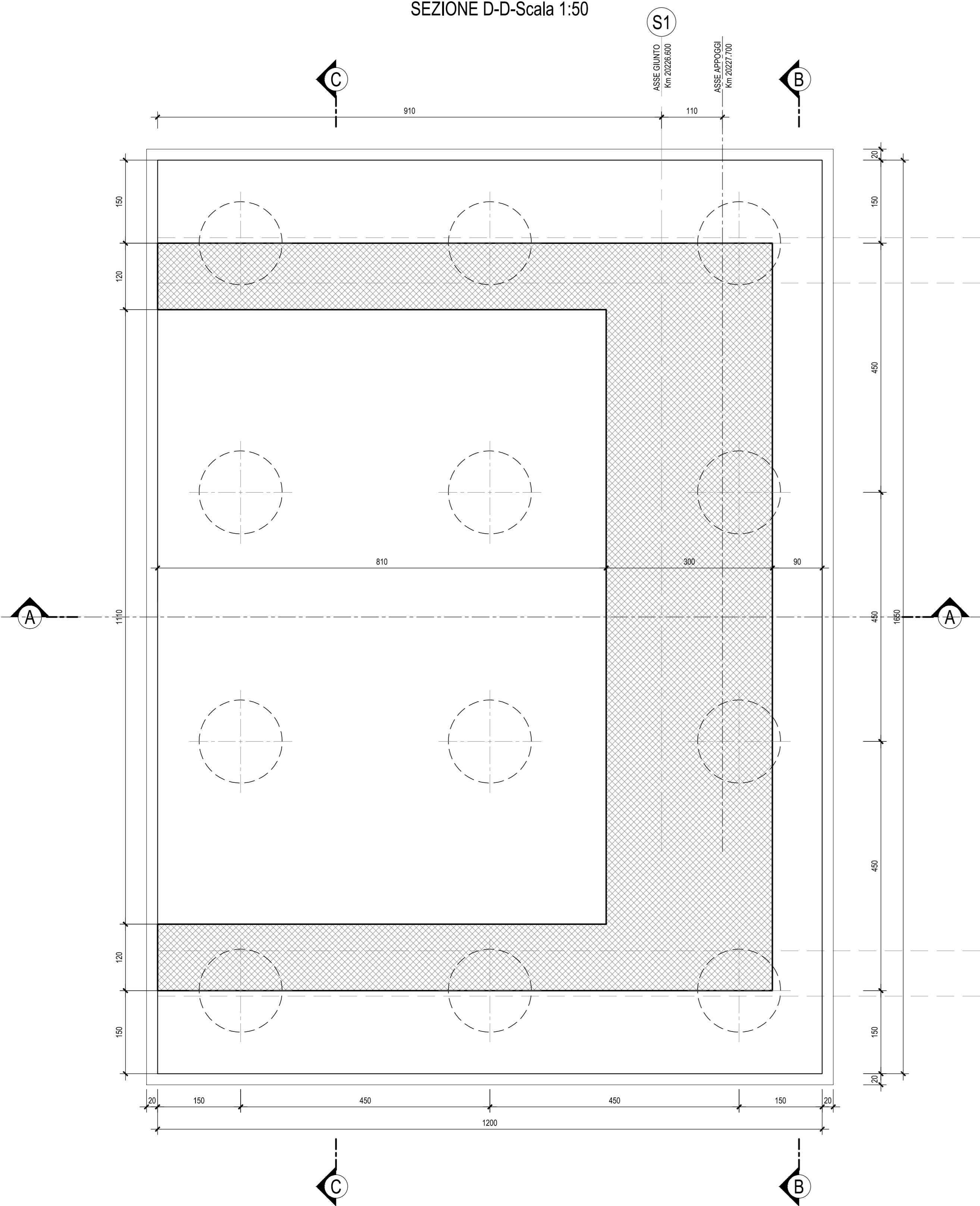
SEZIONE D-D-Scala 1:50
