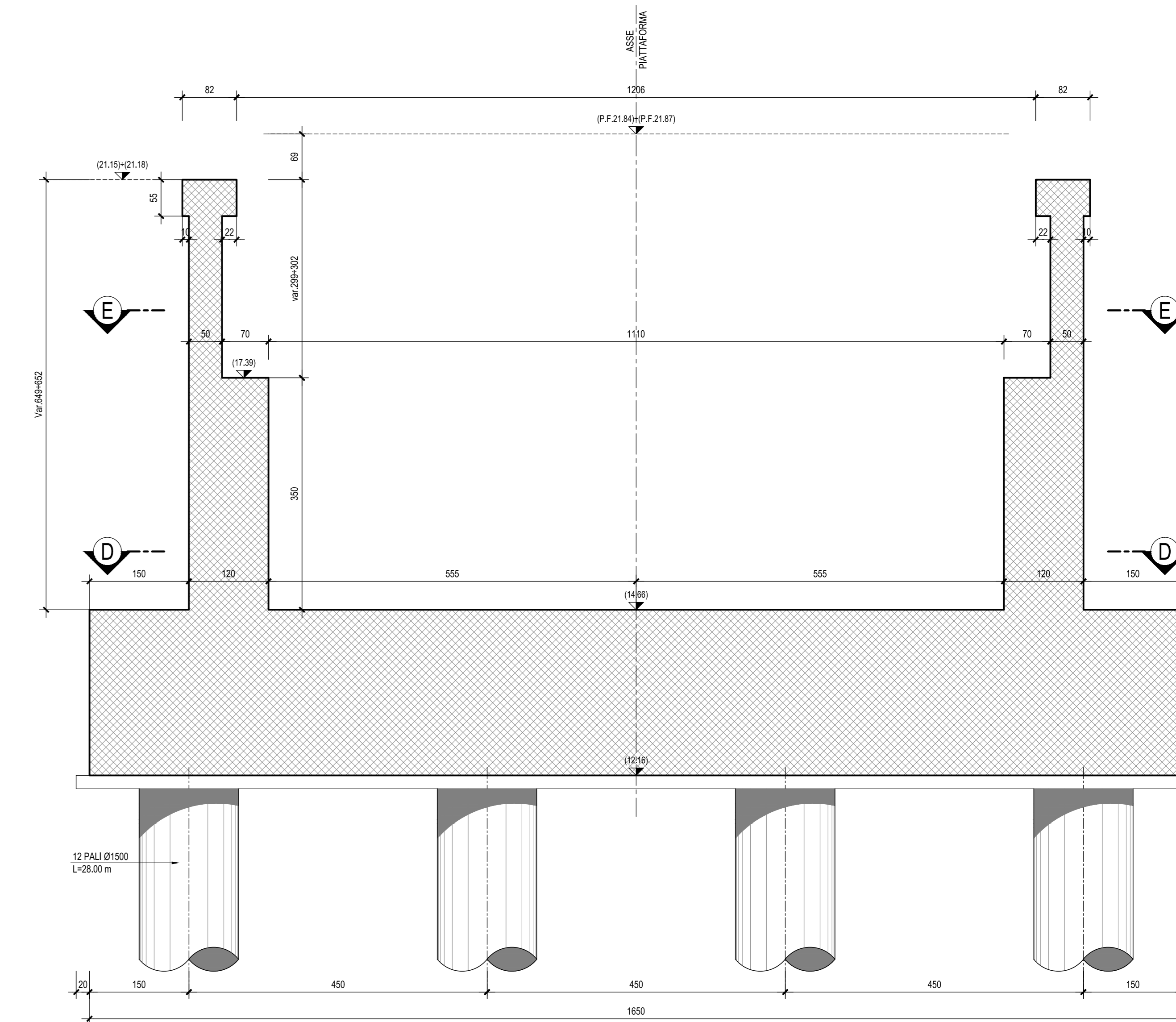
SEZIONE C-C-Scala 1:50
