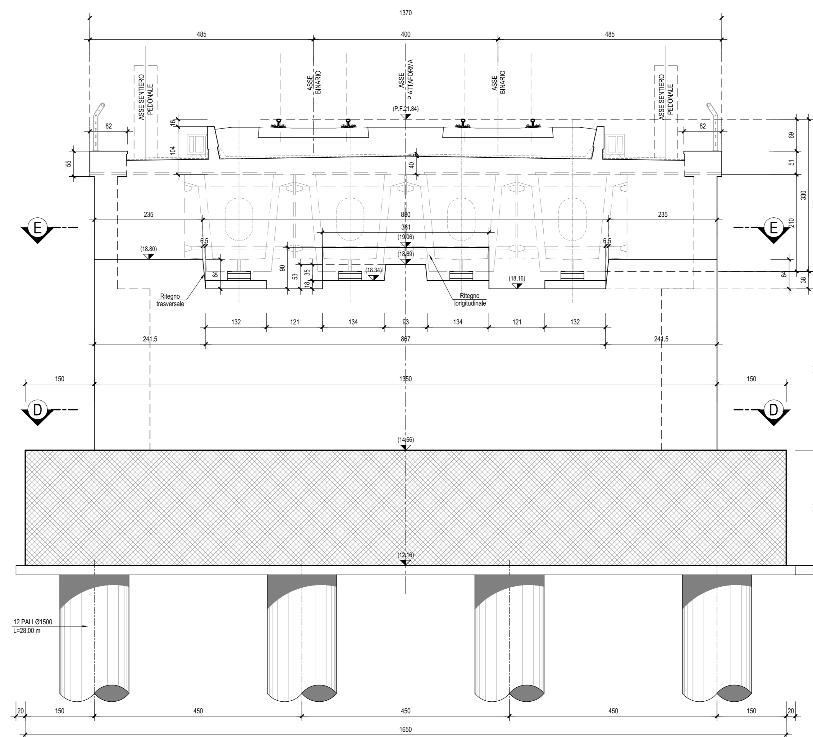
SEZIONE B-B-Scala 1:50
