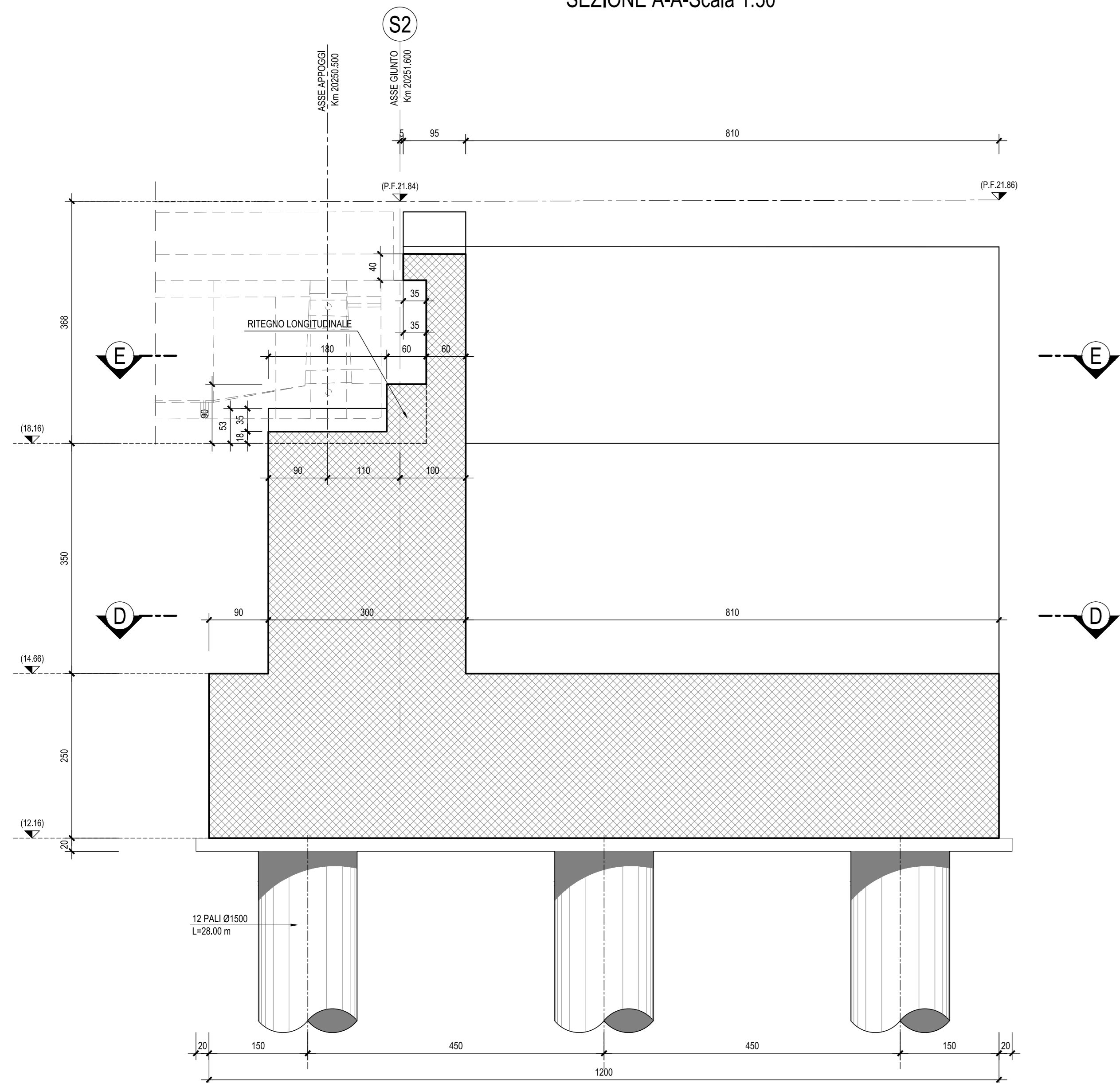
SEZIONE A-A-Scala 1:50
