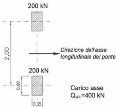
Figura 8: Schema di carico 2 per verifiche locali
