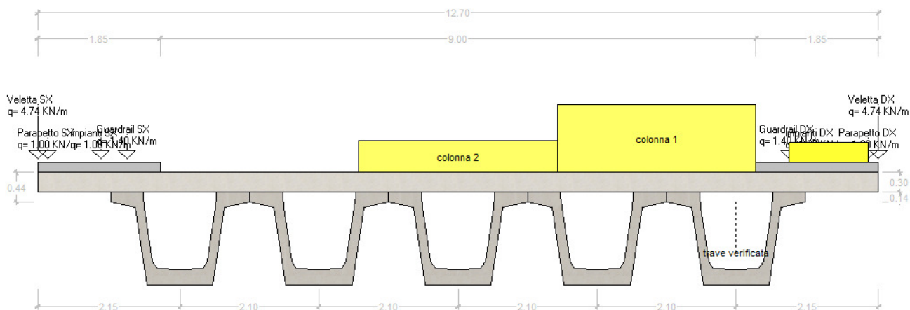
Figura 10 - Disposizione per calcolo trave di bordo
