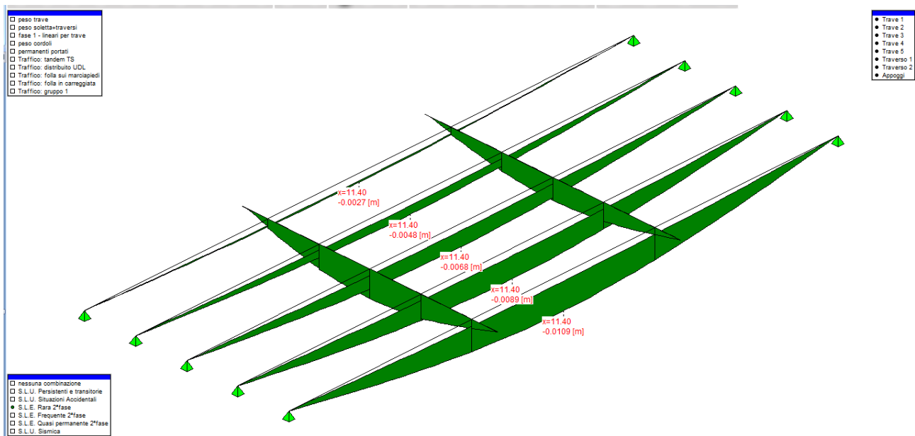
Figura 14 - Freccie SLE rara
