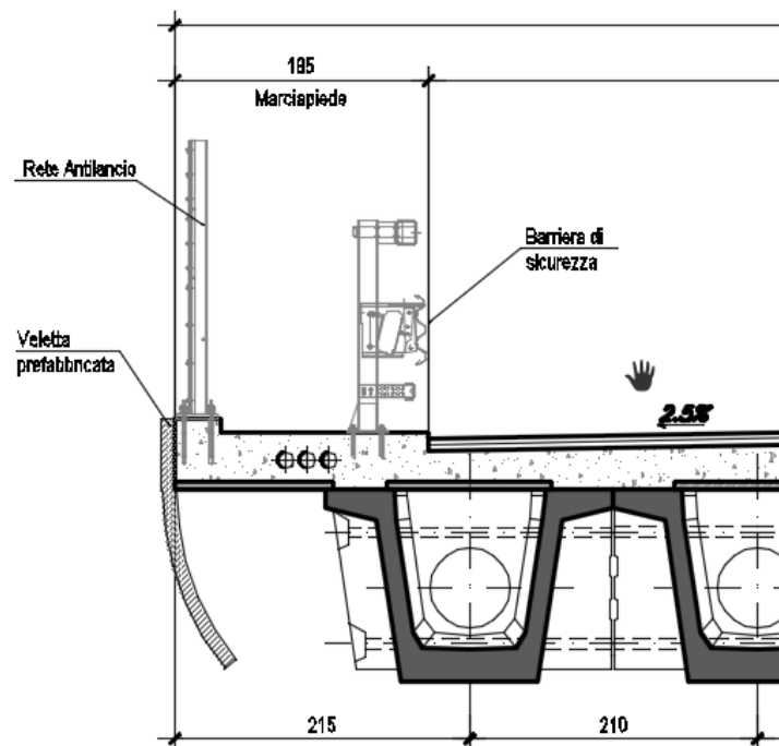
Figura 6 – Marciapiede gettato in seconda fase
