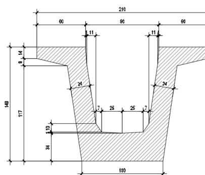
Figura 3 – Sezione della trave in c.a.p.
