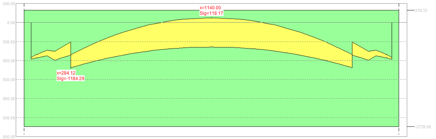
Figura 18 - Momento flettente - RARA - t inf.
