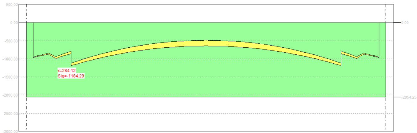
Figura 20 – Momento flettente – QUASI PERMANENTE - t inf.
