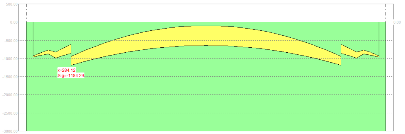
Figura 19 - Momento flettente - FREQUENTE - t inf.
