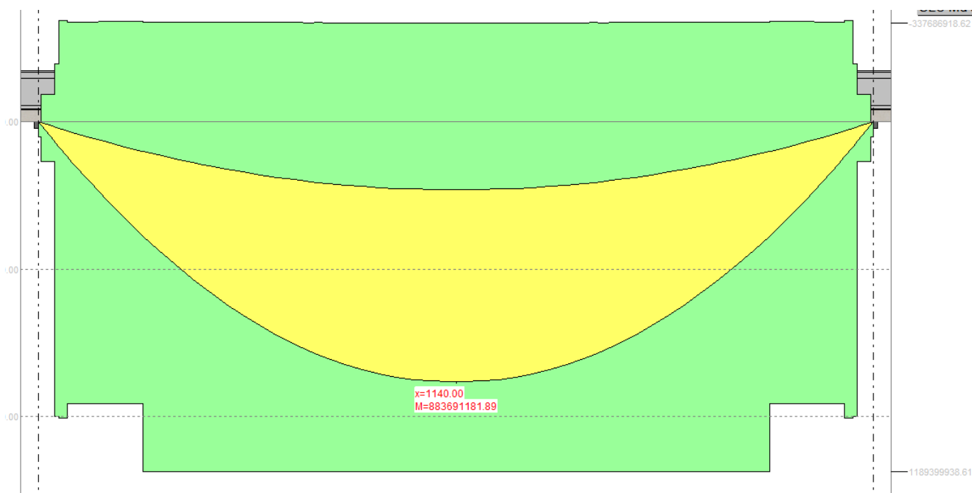
Figura 15 - Momento flettente a t inf.
