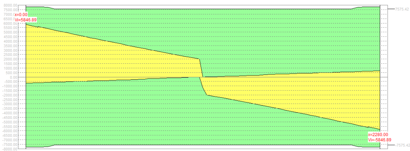
Figura 17 - Scorrimento interfaccia trave-soletta
