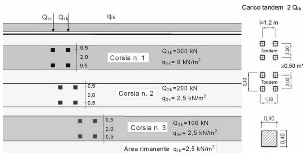
Figura 7 – Corsie: Corsia n°1, corsia n°2 e corsia n°3– Colonne di carico
