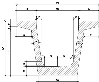
Figura 5 – Sezioni trave in c.a.p.
