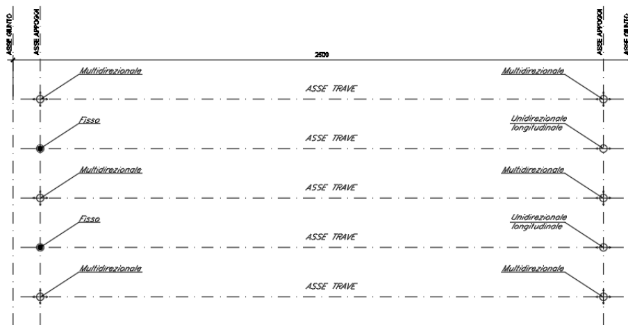
Figura 4 – Schema degli apparecchi di appoggio
