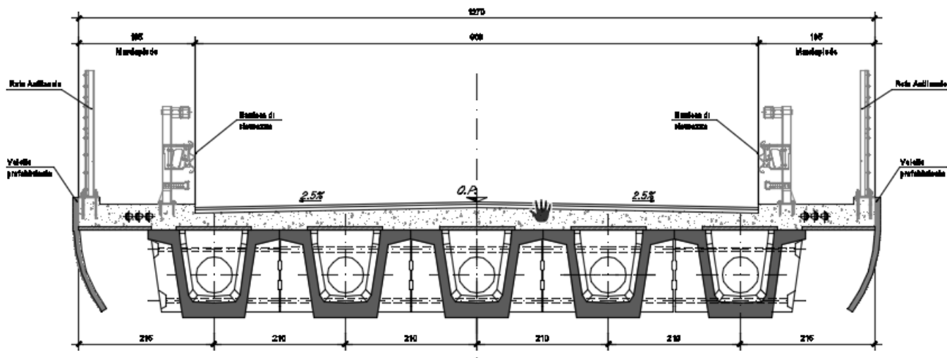
Figura 2 – Sezione tipica trasversale dell'impalcato
