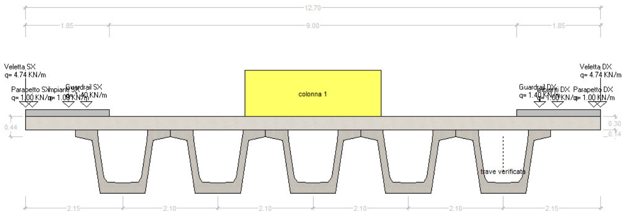
Figura 11 - Disposizione per calcolo M max su trasverso
