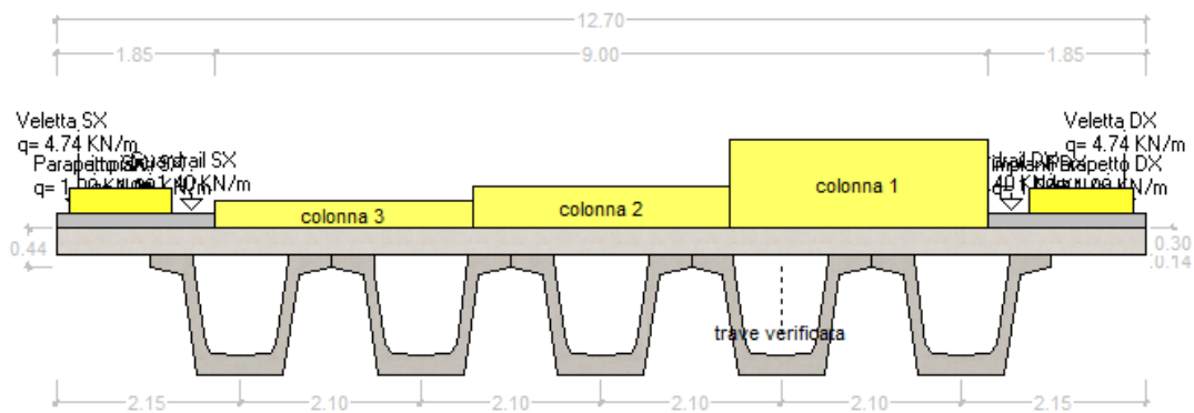
Figura 13 - Disposizione per N max su sottostrutture
