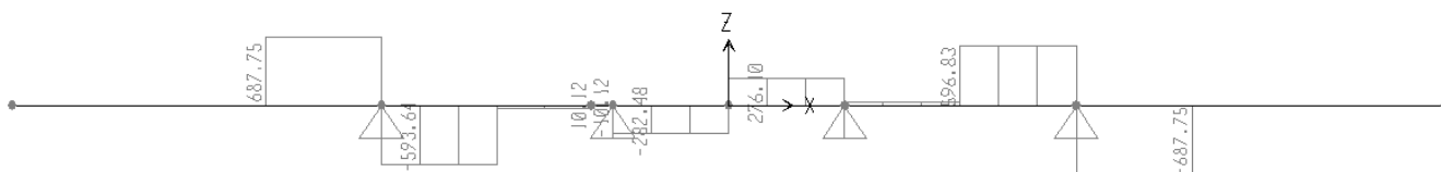
Figura 22 - Momento flettente
