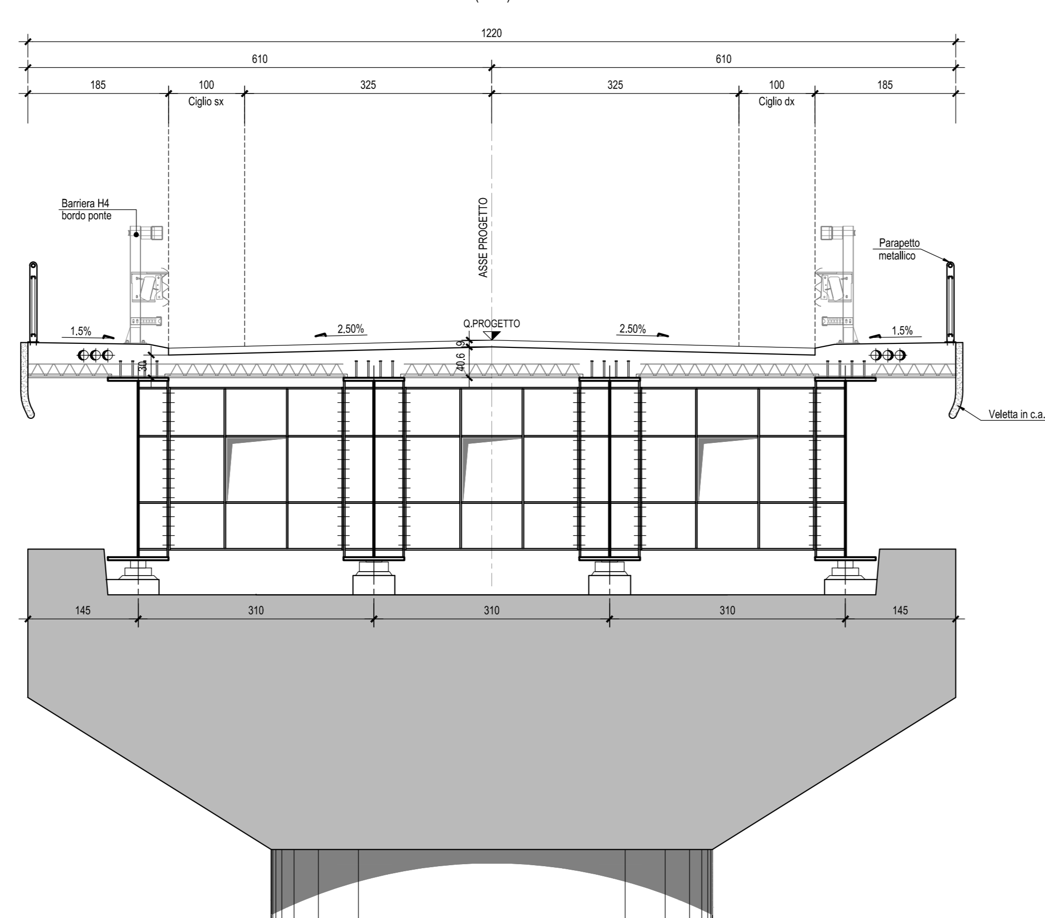
PROSPETTO TIPO APPOGGIO (PILA)-Scala 1:50
