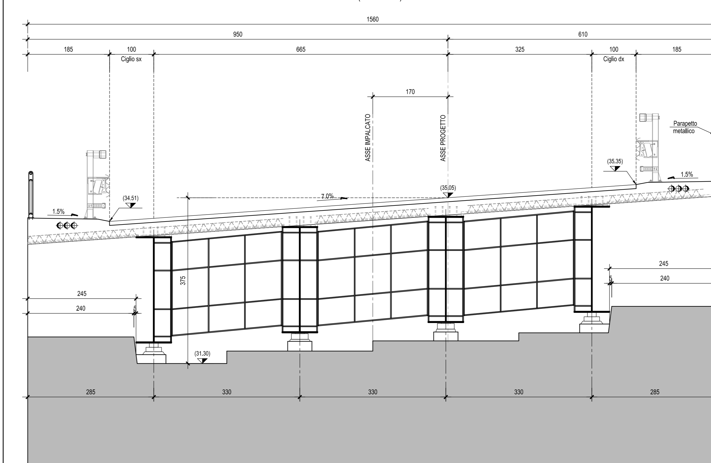
PROSPETTO TIPO APPOGGIO (SPALLA S2)-Scala 1:50
