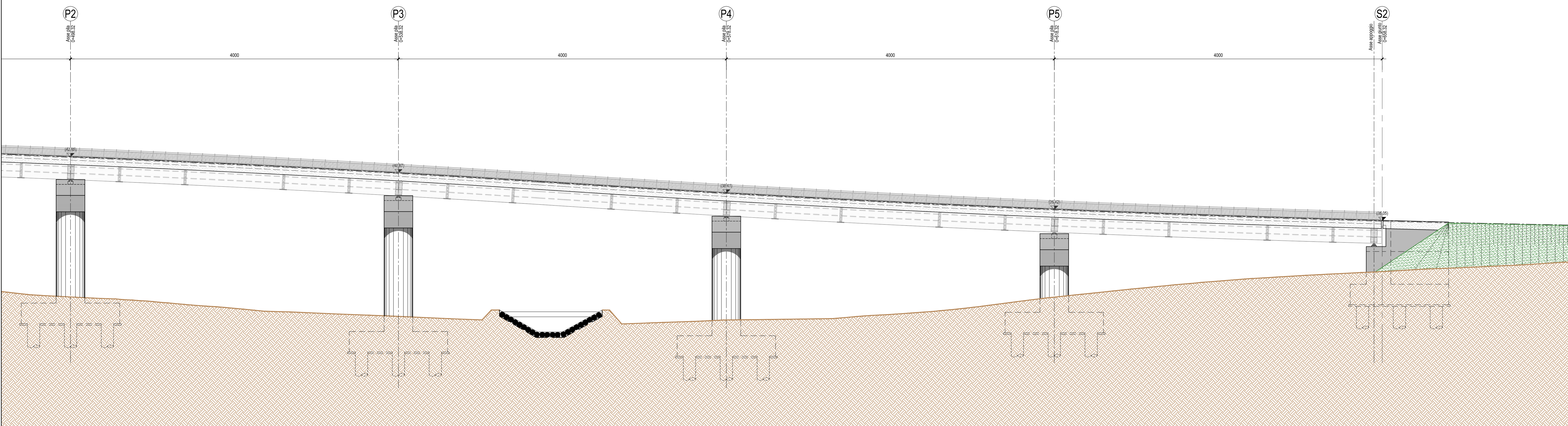
PIANTA IMPALCATO-Scala 1:200
