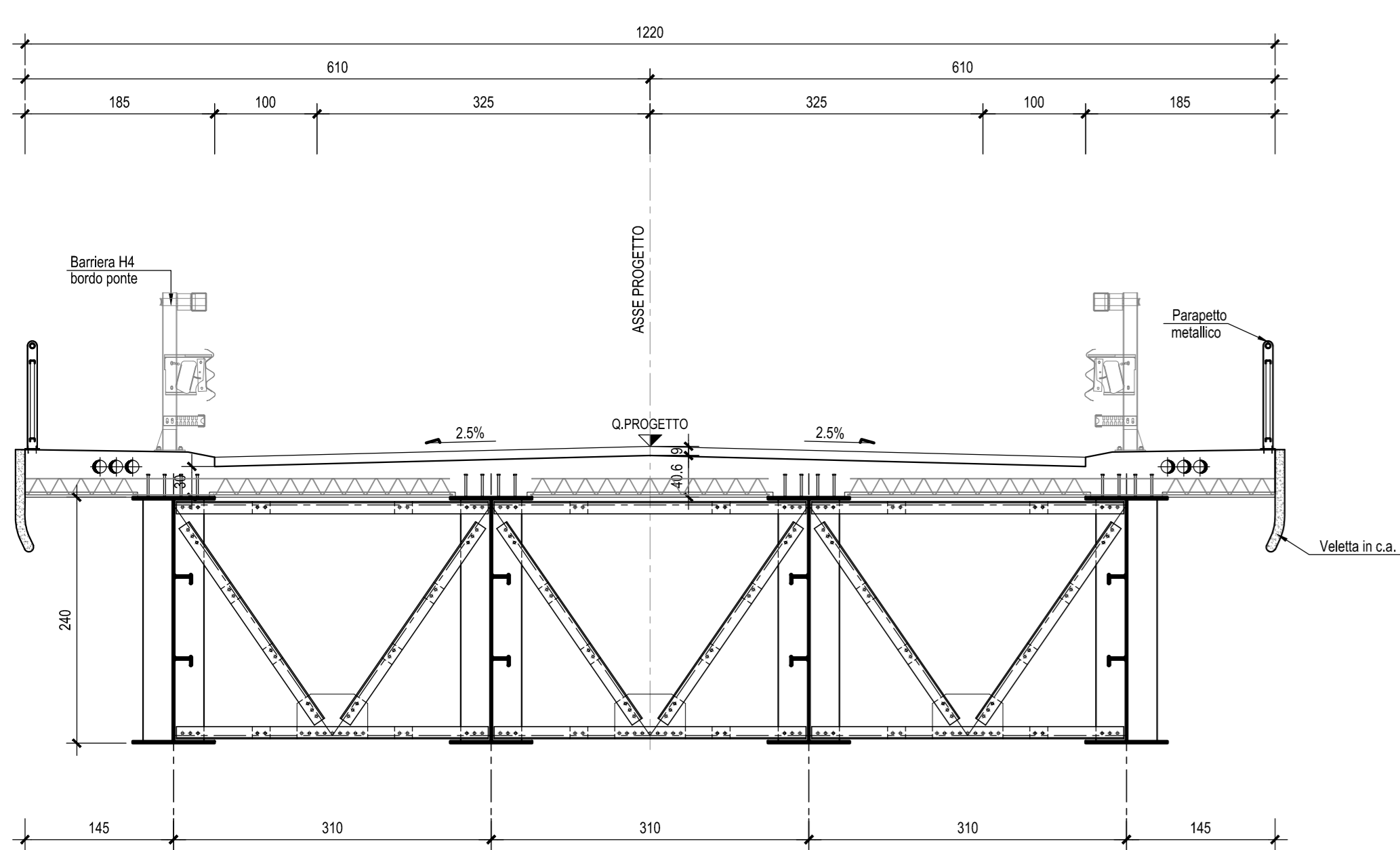
SEZIONE TRASVERSALE TIPO CORRENTE-Scala 1:50
