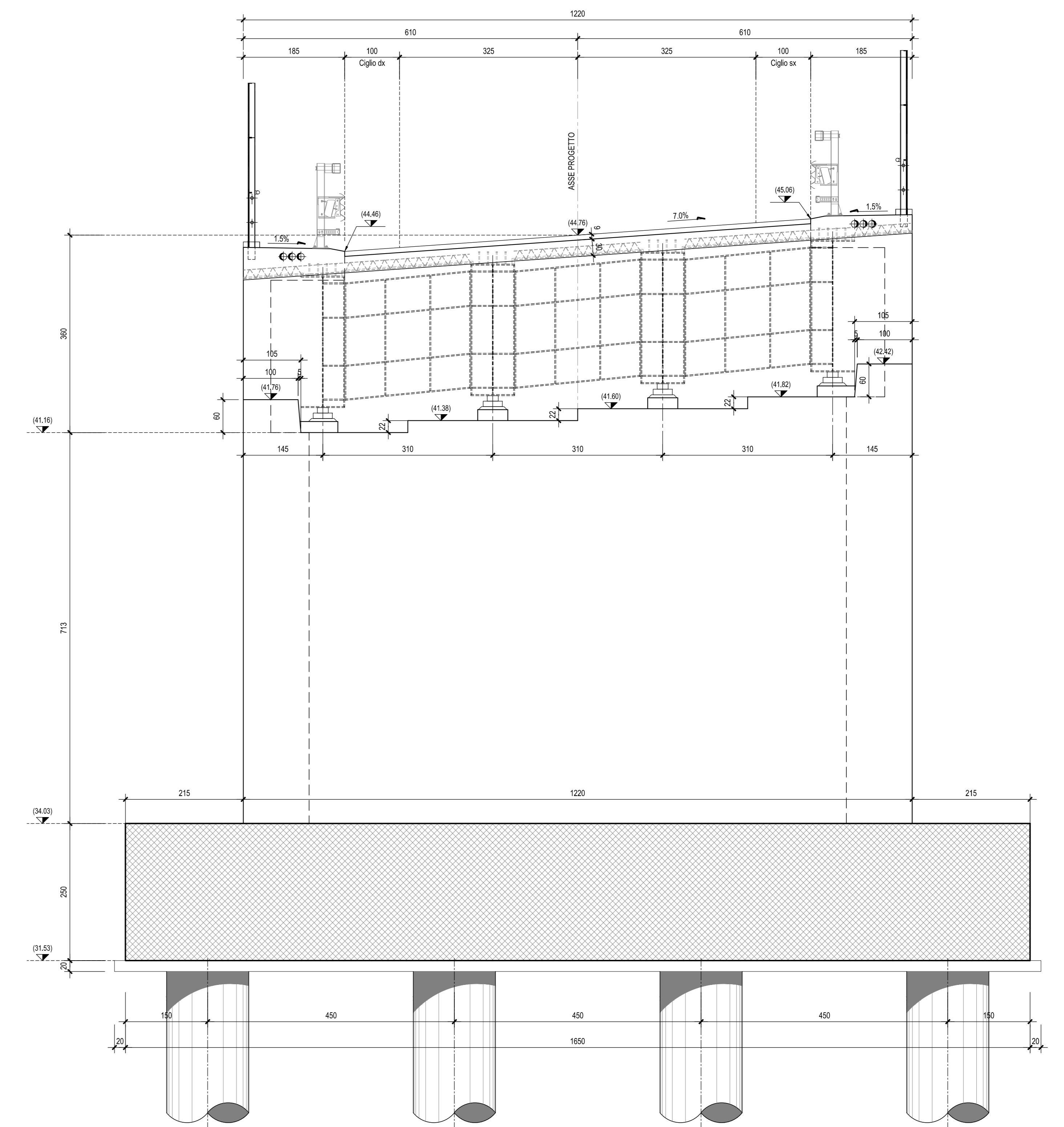
SEZIONE B-B-Scala 1:50
