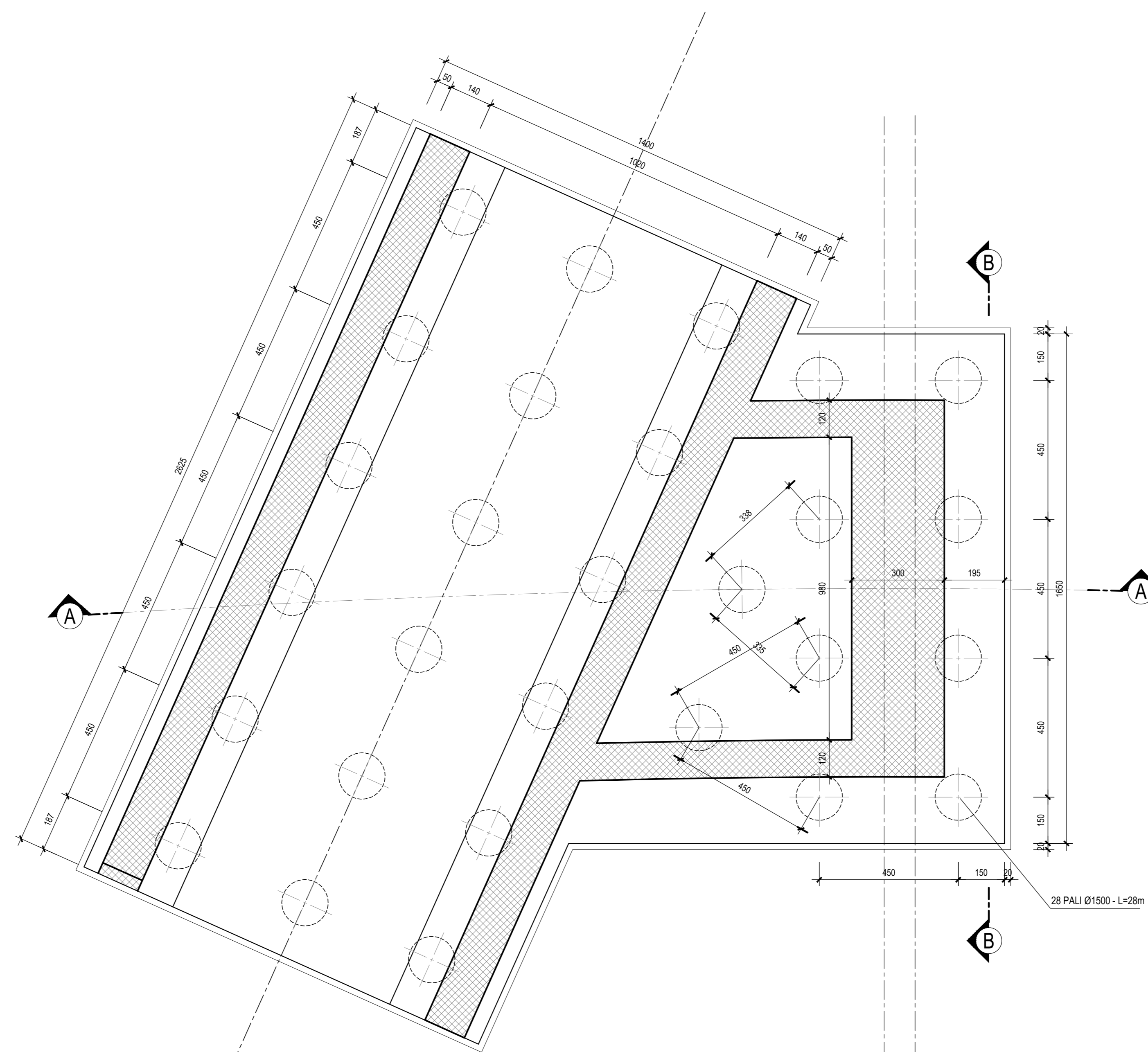
PIANTA FONDAZIONI-Scala 1:100
