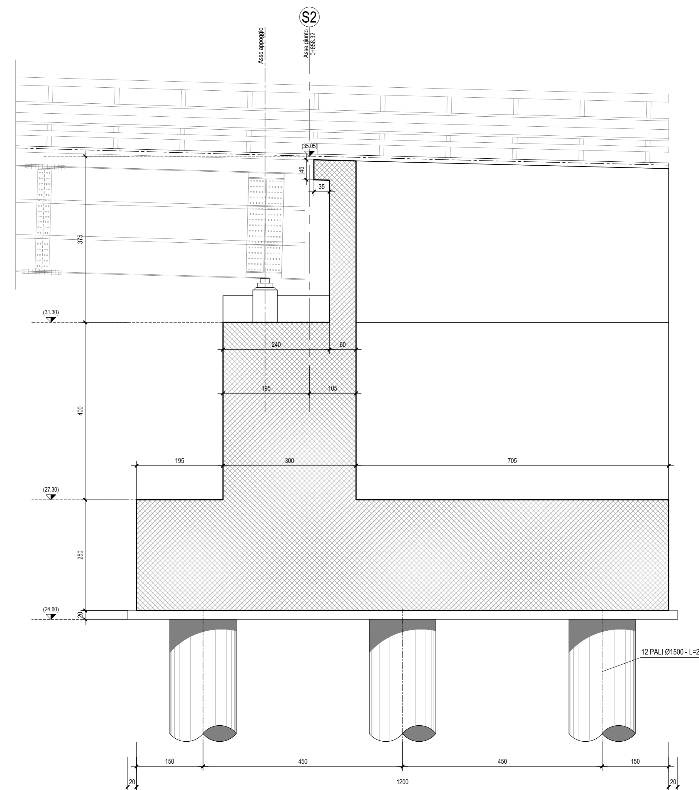
SEZIONE B-B-Scala 1:50
