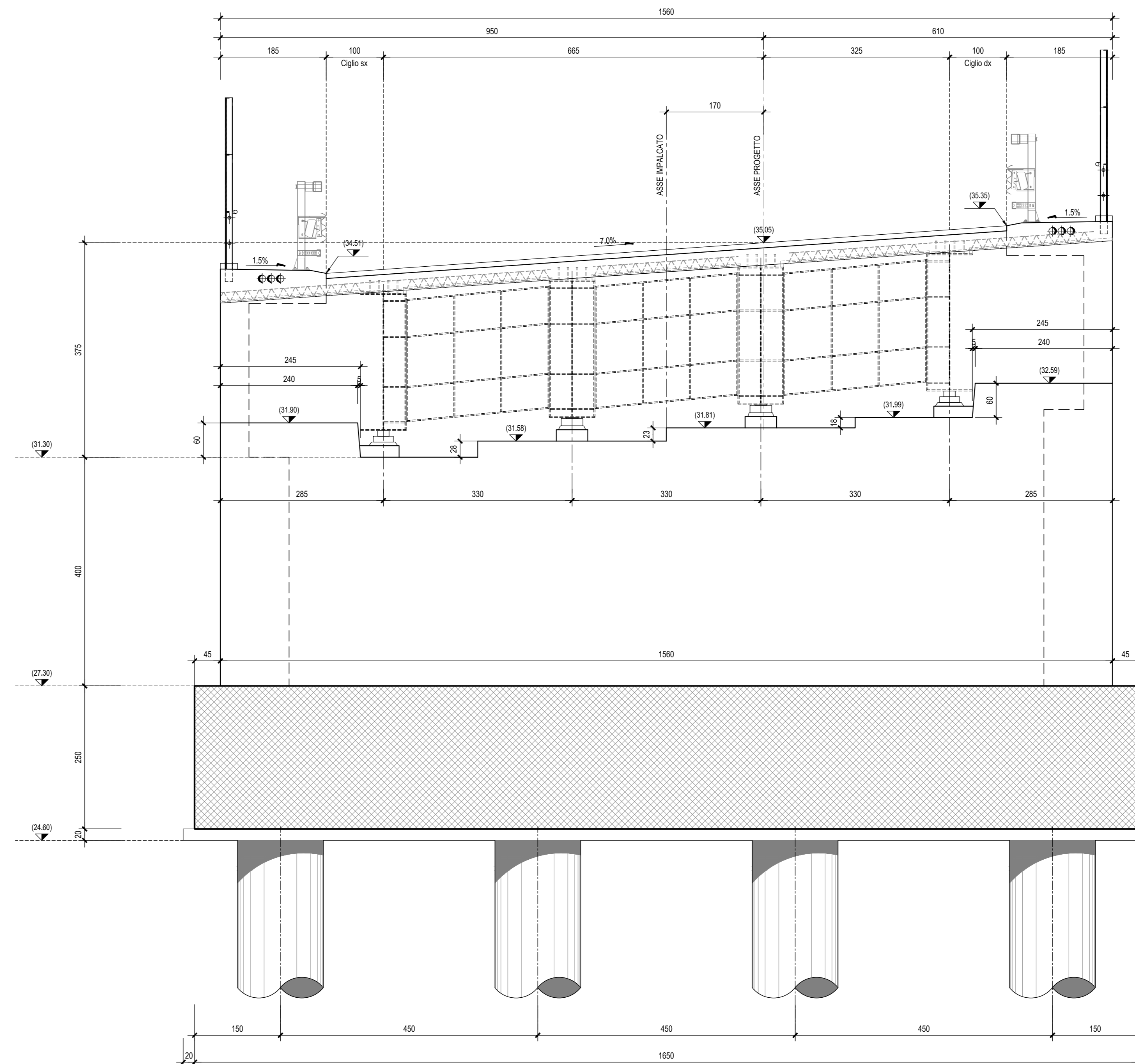
SEZIONE B-B-Scala 1:50
