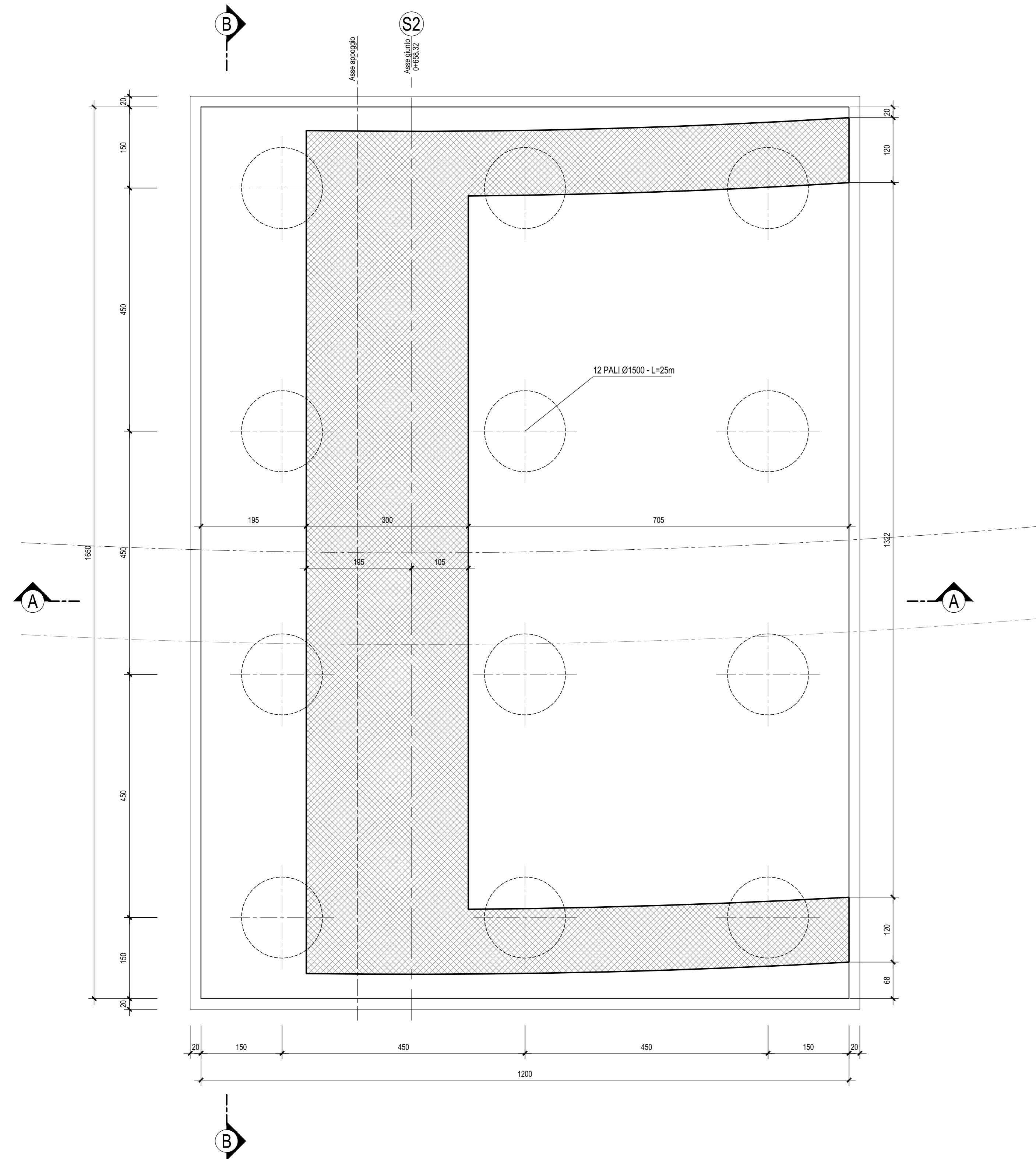
PIANTA FONDAZIONI-Scala 1:50
