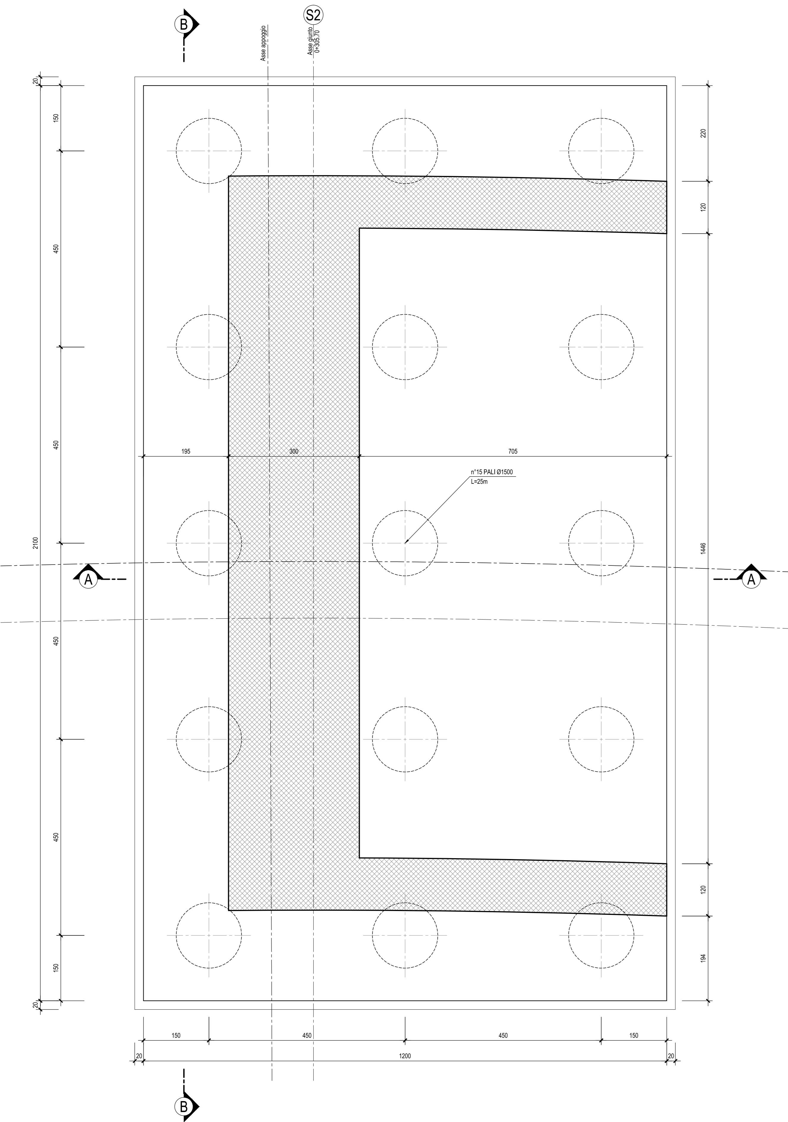
PIANTA FONDAZIONI-Scala 1:50
