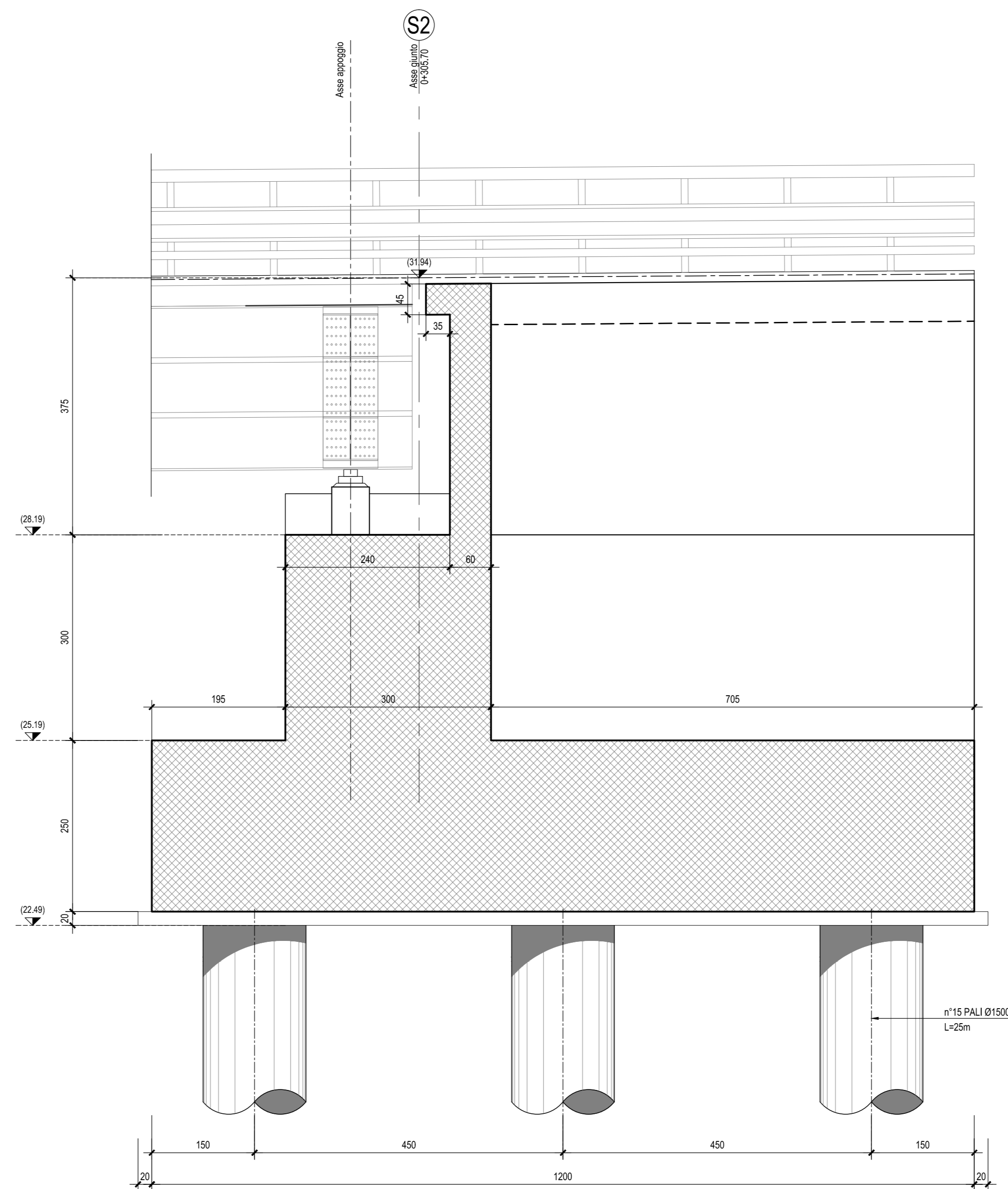
SEZIONE A-A-Scala 1:50
