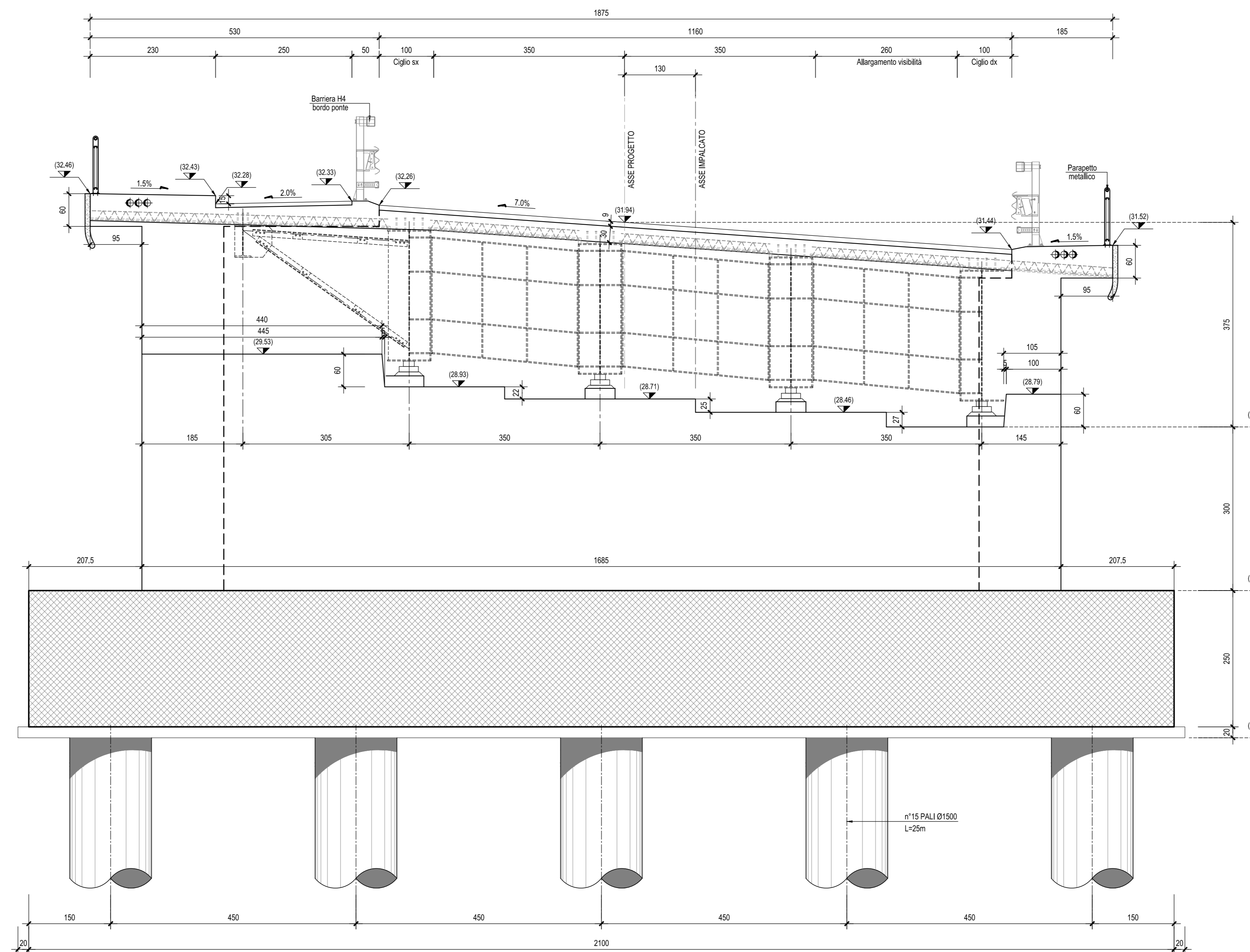
SEZIONE B-B-Scala 1:50
