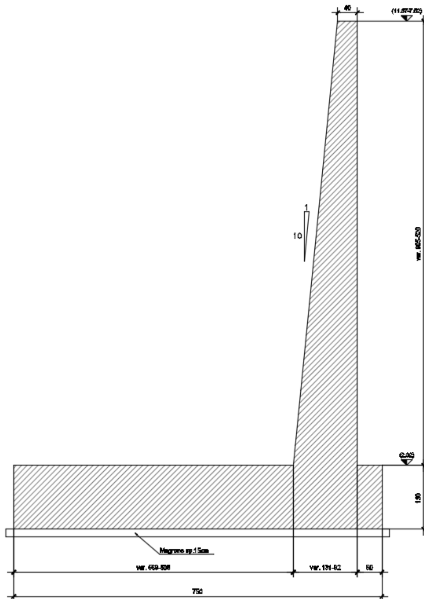
Fig. 5 – Sezione di riferimento muro tipo H_{max}=9.05m
