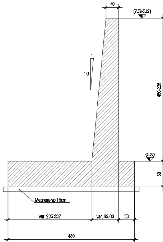
Fig. 6 – Sezione di riferimento muro tipo H_{max}=4.50m
