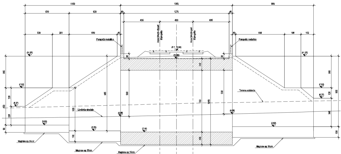
Fig. 1 - Sezione longitudinale
