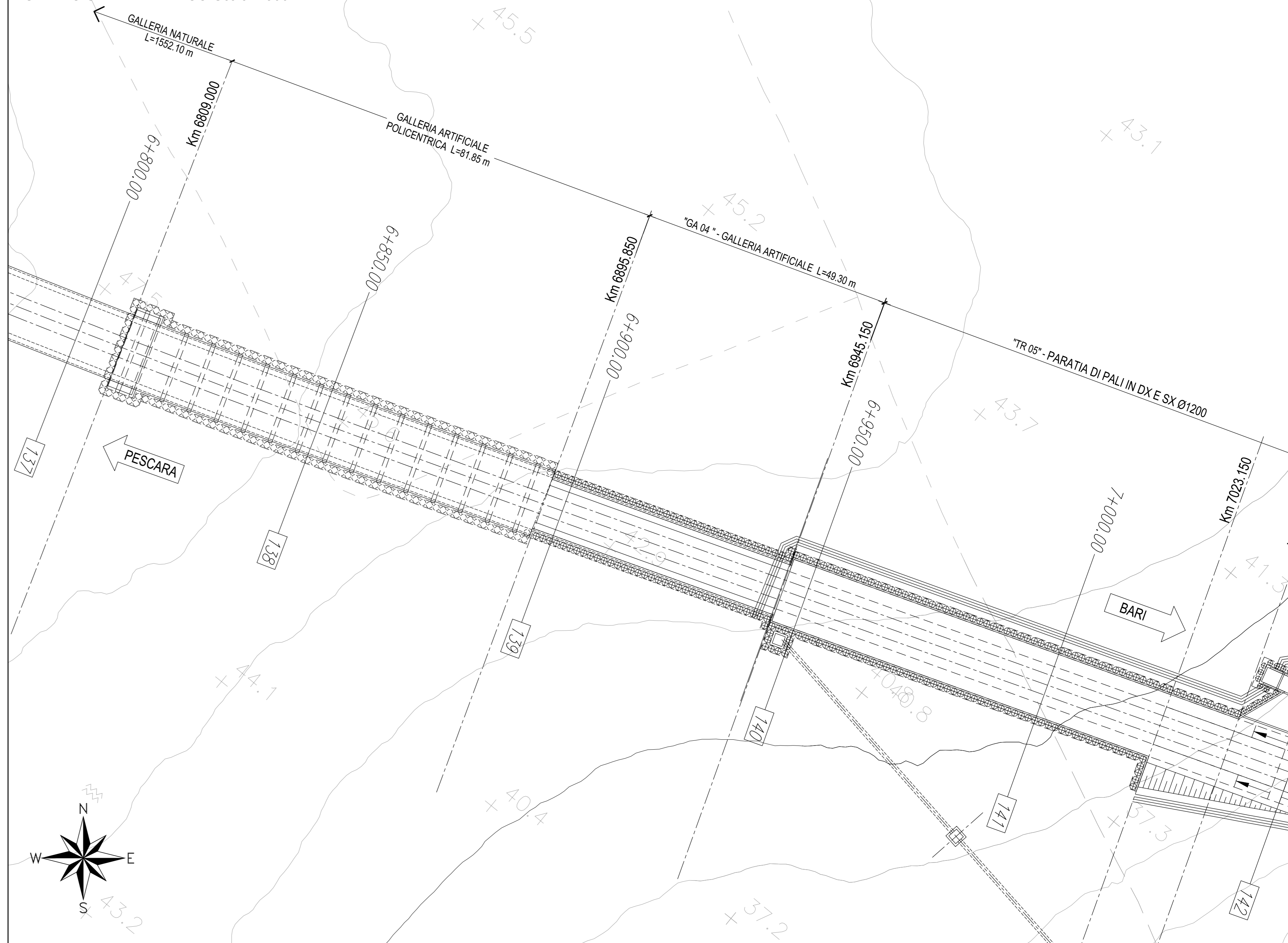
STRALCIO PLANIMETRICO-Scala 1:500
