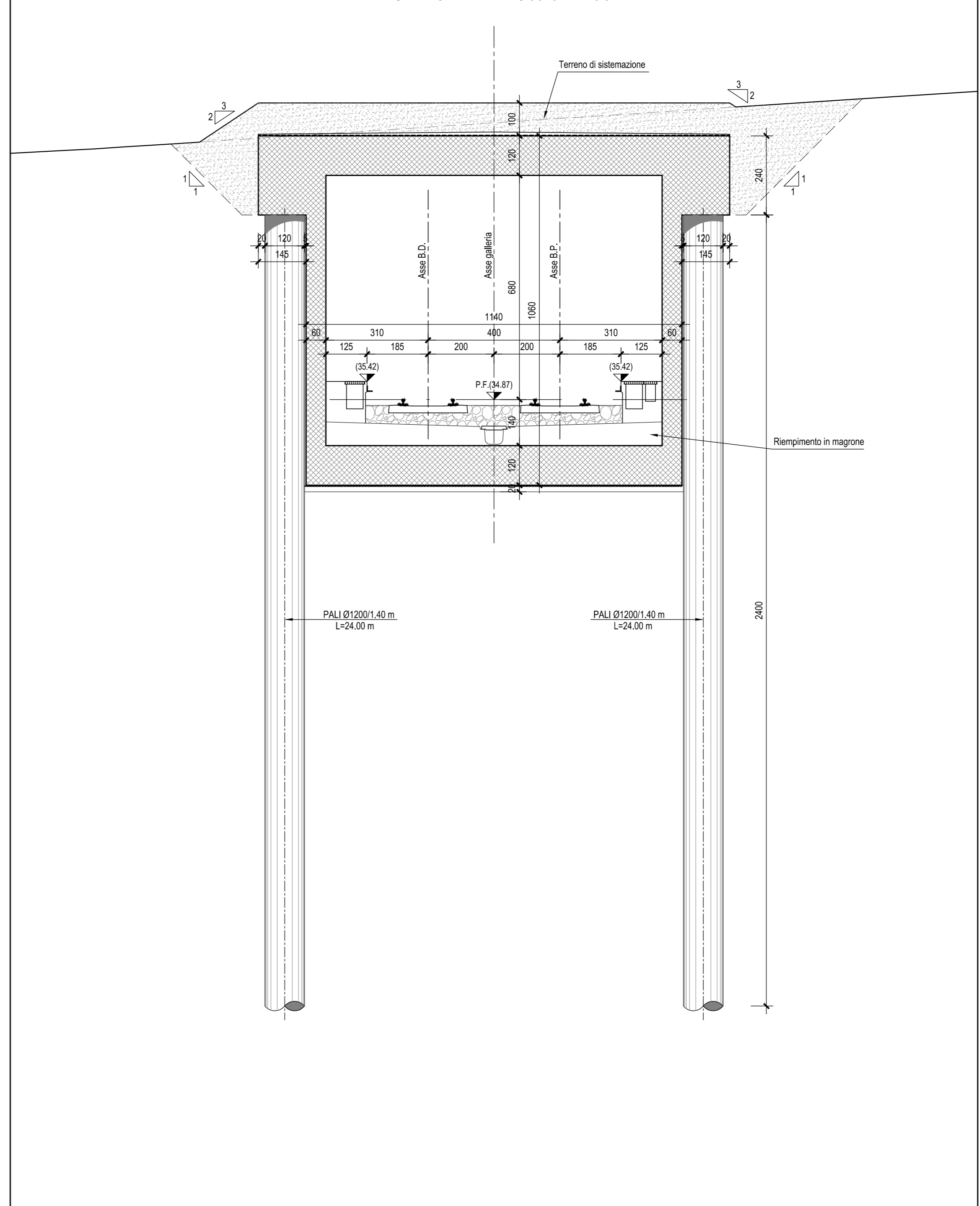
SEZIONE A-A-Scala 1:100
