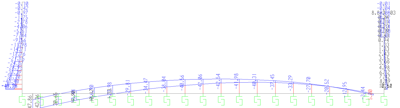
Fig. 6 – Involuppo momenti flettenti SLV
