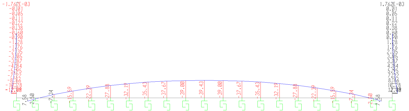
Fig. 9 – Involuppo momenti flettenti SLE rara
