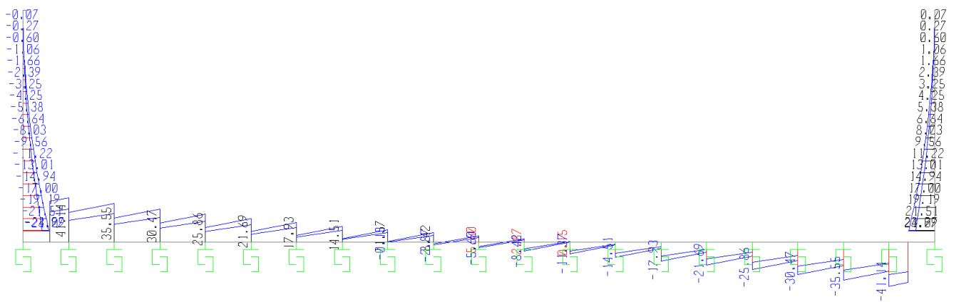
Fig. 4 – Involuppo sforzi taglienti SLU
