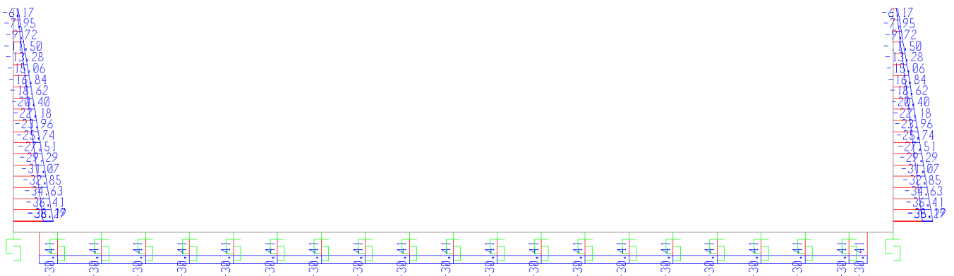
Fig. 5 – Involuppo azioni assiali SLU
