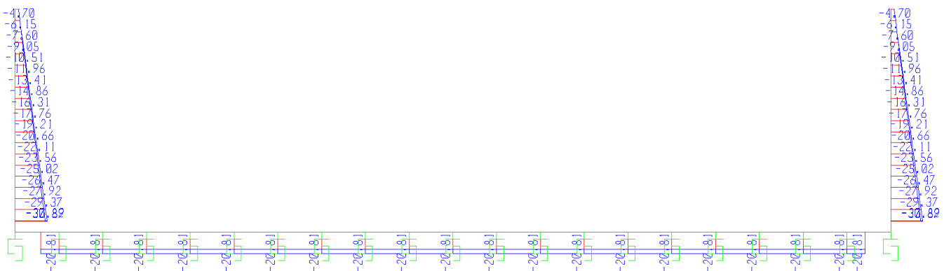
Fig. 8 – Involuppo azioni assiali SLV
