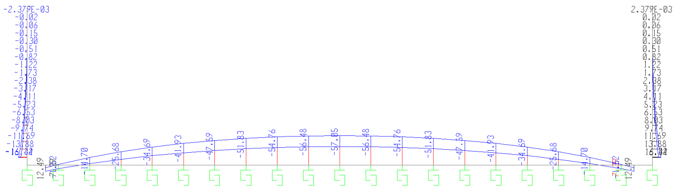
Fig. 3 – Involuppo momenti flettenti SLU
