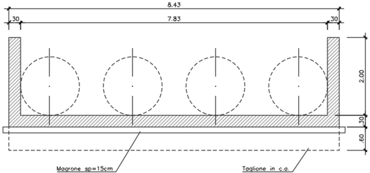
Fig. 1 – Sezione trasversale
